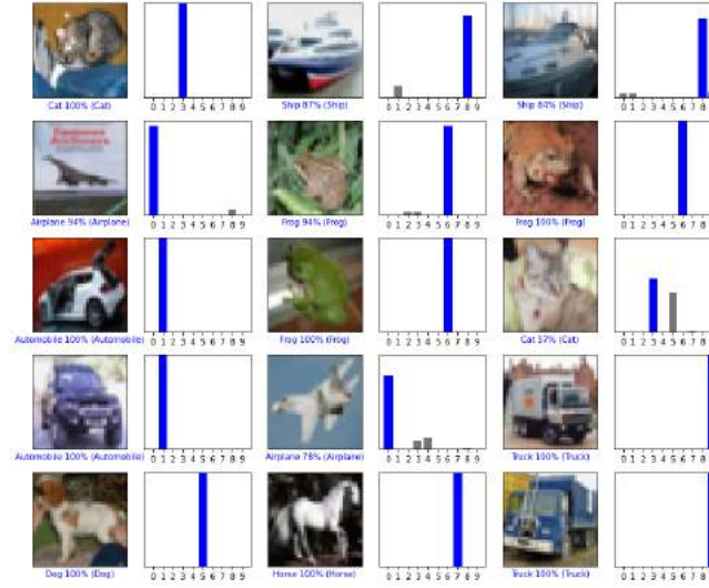
Figura 4.3: Comprobación de las predicciones para las quince primeras fotografías de CIFAR-10.
