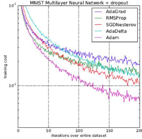
Figura 3.1: Resultado del entrenamiento de una red neuronal multicapa para el conjunto de imágenes MNIST empleando distintos optimizadores (ver [15]).
