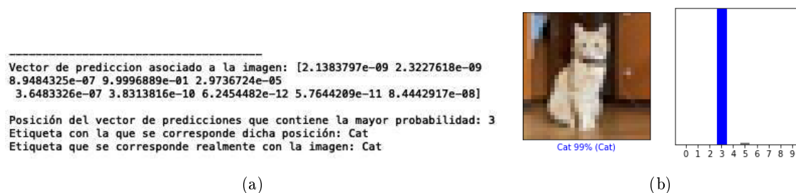
Figura 4.4: Clasificación de una imagen no perteneciente al conjunto CIFAR-10.
