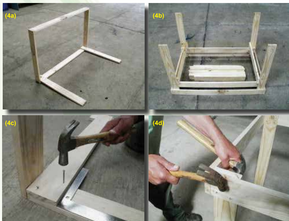
Foto 4. Colocando las 4 piezas de 84 cm que forman las 4 patas del cajón.
