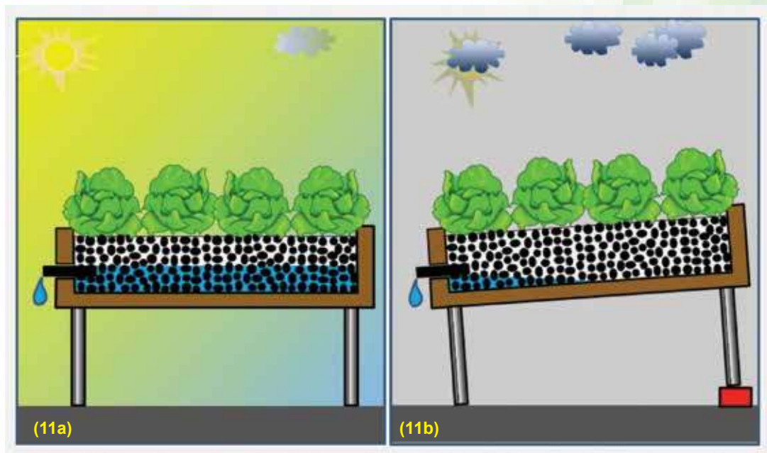
Figura 11. Cama nivelada en verano (11a) y otra mostrando desnivel con calzas en el invierno (11b).
