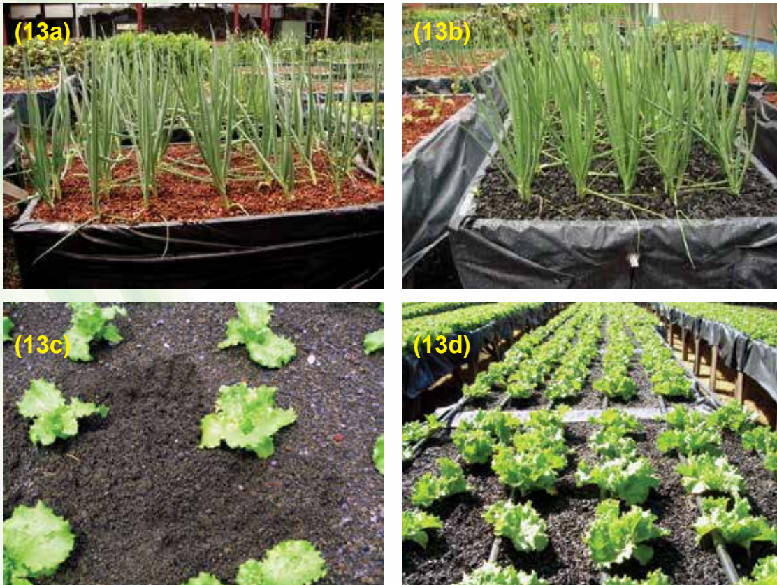
Foto 13. Diferentes tipos de sustratos usados en el cultivo en camas, (13a) piedra roja volcánica, (13b) carbón vegetal, (13c) arena fina de tajo y (13d) piedrilla de tajo.
