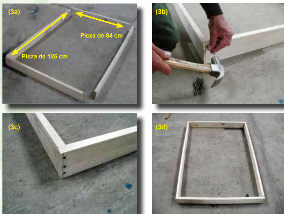
Foto 3. Preparando el marco del cajón con 2 piezas de 84 cm para el ancho y 2 pieza de 125 cm para el largo de la cama.
