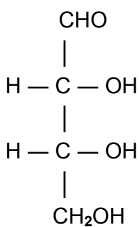
D-erythrose
