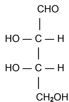
L-erythrose
