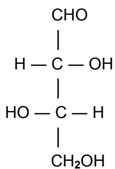
L-threose
