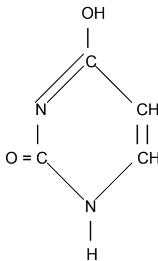
lactim
