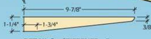
DETAIL 2—STIFFENER—F
