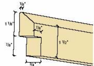
Back Rod
