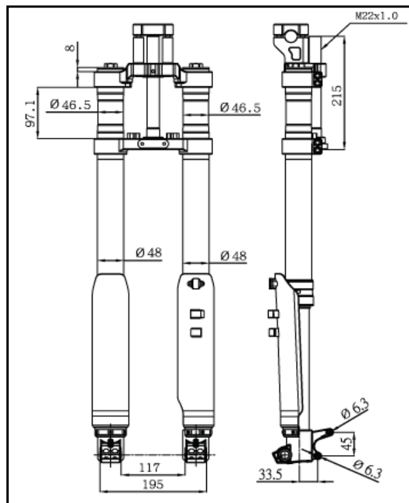
Figura 13. Ejemplo de horquilla
