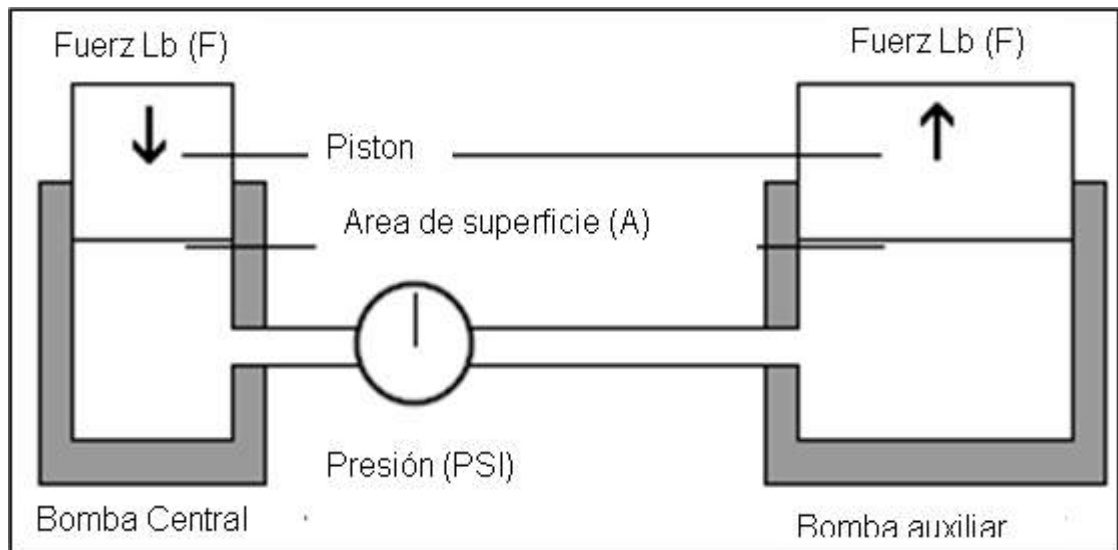
Figura 17. Diagrama de funcionamiento de bomba de frenos
