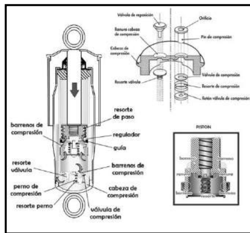
Figura 11. Partes de un amortiguador
