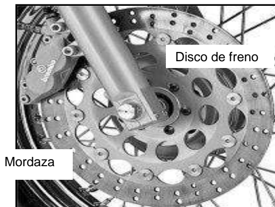
Figura 15. Disco de freno y mordaza
