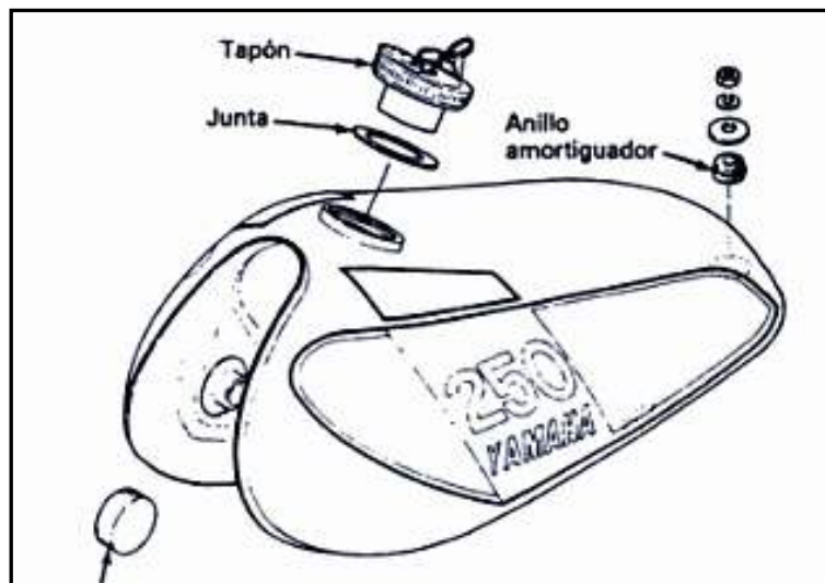
Figura 3. Deposito y tapón de motocicleta, (Yamaha Internacional Corporation)
