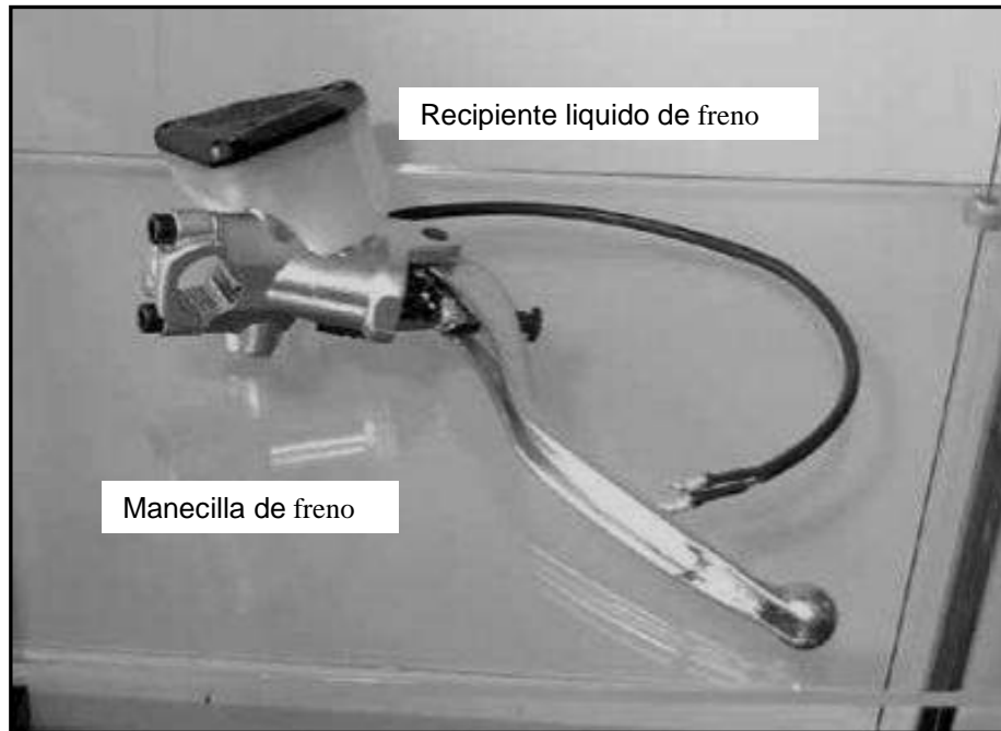
Figura 16. Bomba de freno y manecilla
