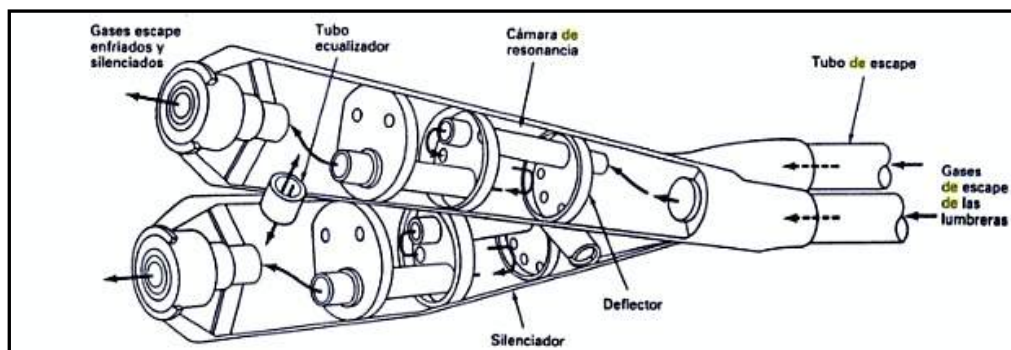
Figura 8. Vista en corte de silenciadores de una moto pluricilindrica, las flechas indican la trayectoria de los gases de escape, (Honda Motor Company, Ltd.)
