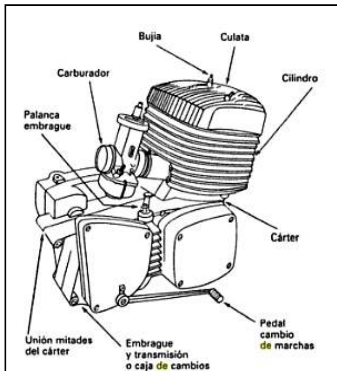
Figura 2. Motor de motocicleta mono cilíndrico de dos tiempos, (Husqvarna)
