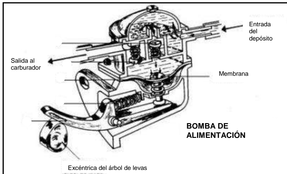
Figura 4. Bomba de alimentación de membrana
