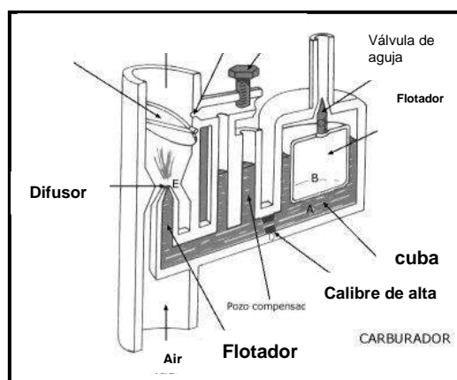
Figura 5. Carburador
