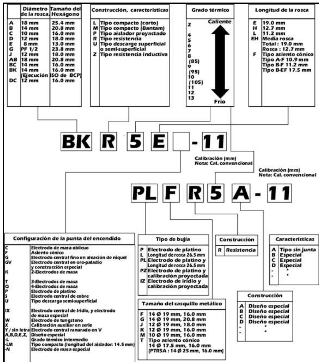
Figura 18. Nomenclatura de las bujías
