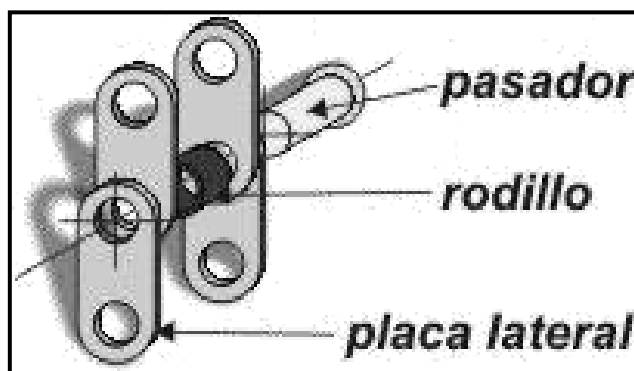
Figura 10. Partes de un eslabón de cadena
