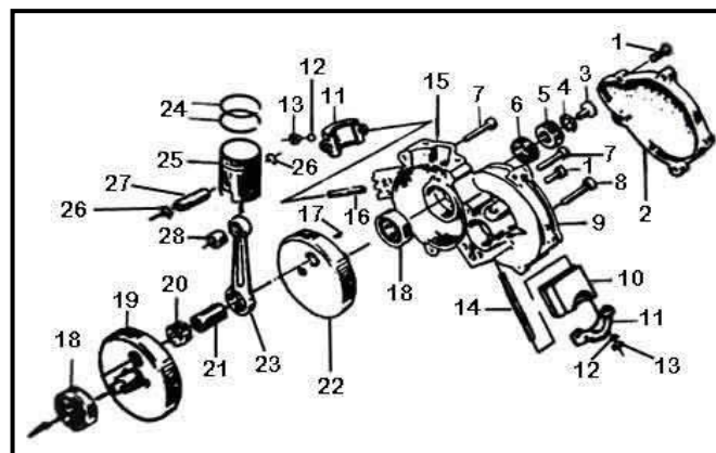
Figura 7. Partes de cigüeñal
