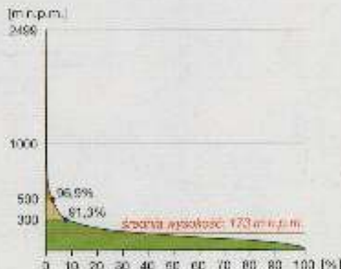
Krzywa hipsograficzna Polski
