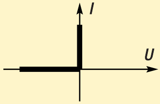
● Curva característica de un diodo ideal.
