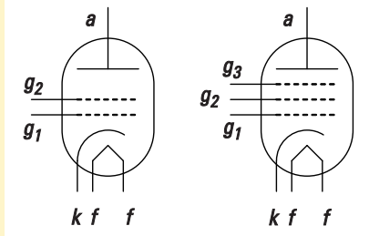
• Válvulas tetrodo y pentodo. ff : filamento; k : cátodo; a : ánodo; g 1 : grilla sensible; g 2 : grilla pantalla; g 3 : grilla supresora.
