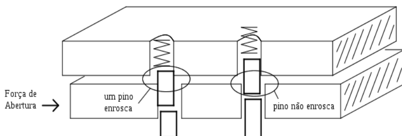
Figura 4.1: A força de abertura faz com que um pino controlador enrosque
