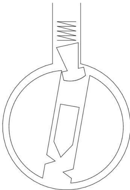
Figura 9.7: Pinos controladores em forma de cogumelo, de carretel e dentado
