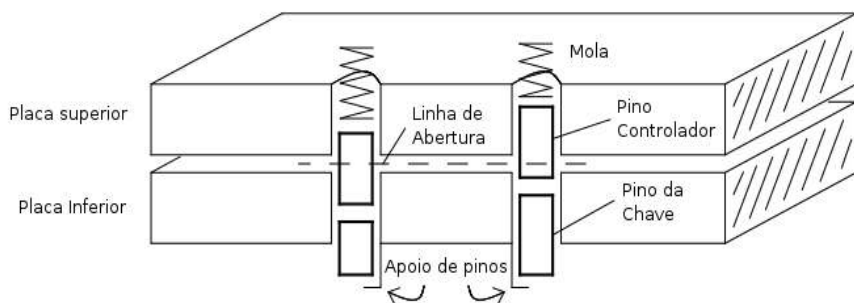
Figura 3.1: Modelo de placas planas de uma fechadura
