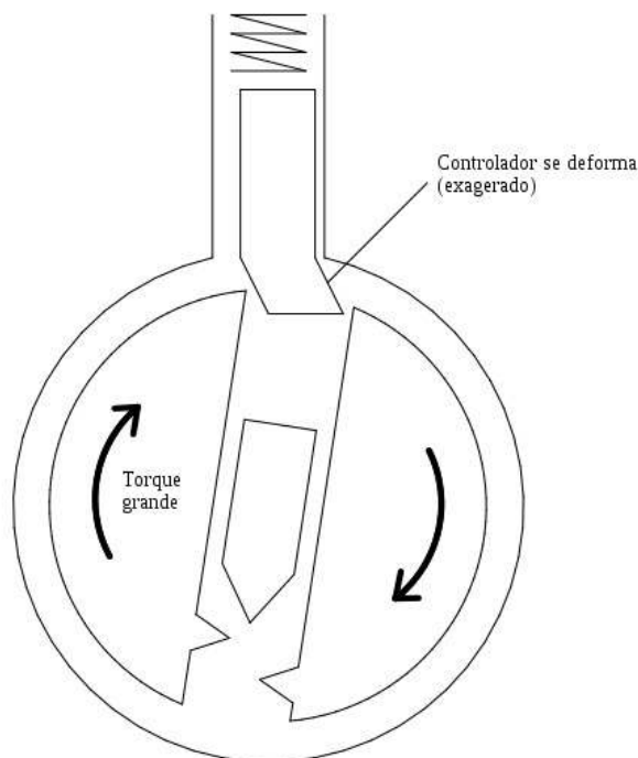
Figure 9.2: Pino controlador com encaixe falso devido à deformação elástica
