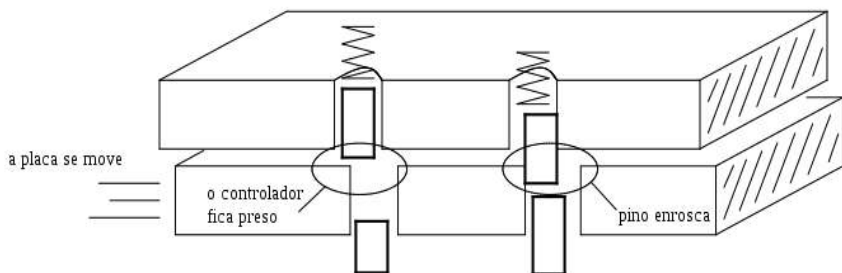
Figure 4.3: O controlador da esquerda está encaixado e o da direita enrosca.
