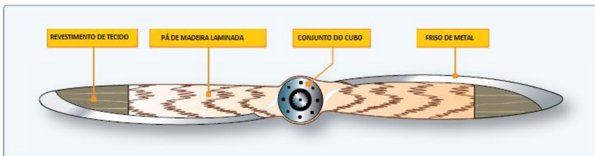
Figura 7-7 Hélice de madeira de passo fixo.
