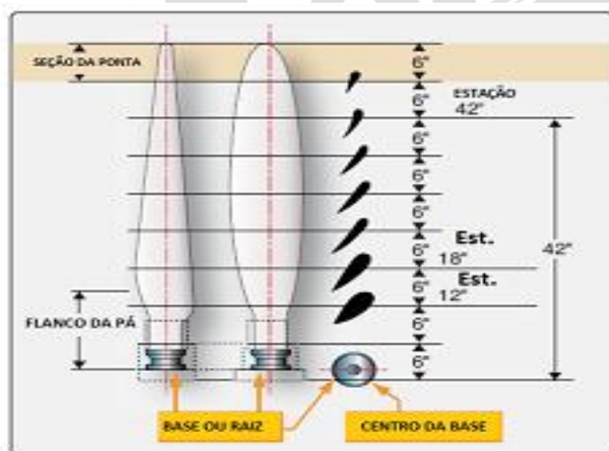
Figura 7-2 Elementos de uma típica pá de hélice.
