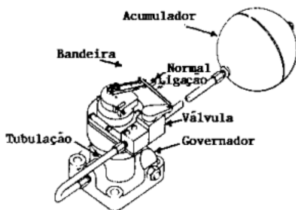
Figura 7-15 Sistema de desembandeiramento.
