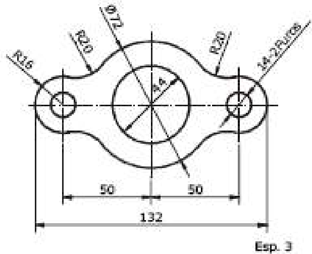
Vista cotada (com as dimensões)
