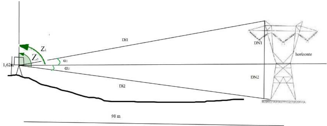
Figura 4.8: Exemplo 4.9
