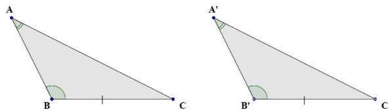
Figura 1.12: Caso LAA_o
