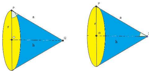
Figura 4.5: Exemplo 4.6
