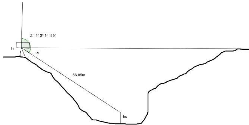
Figura 4.9: Exemplo 4.9
