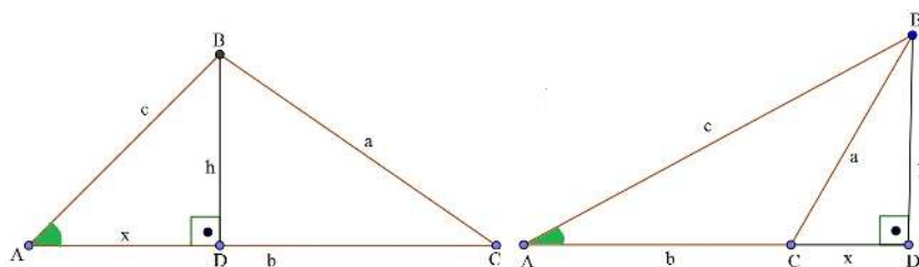
Figura 3.3: \hat{A} < 90^\circ
