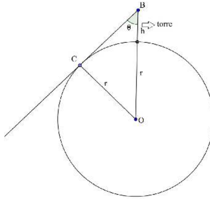
Figura 4.1: Cálculo do raio da terra pelo gregos
