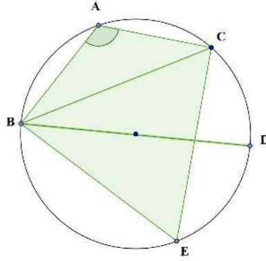
Figura 3.2: Lei dos Senos \hat{A} > 90^\circ
