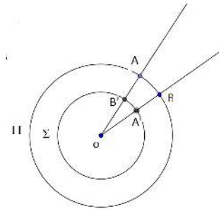
Figura 1.4: Ângulo
