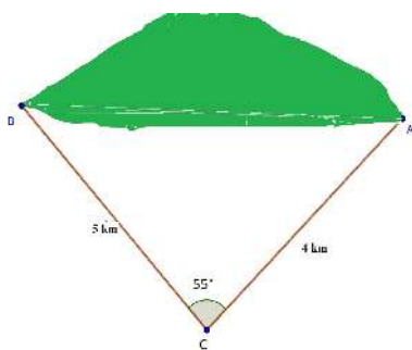
Figura 4.3: Exemplo 4.4
