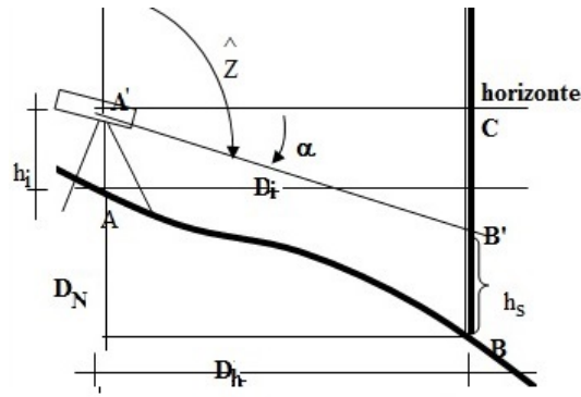
Figura 4.7: Desnível: \hat{Z} > 90^\circ
