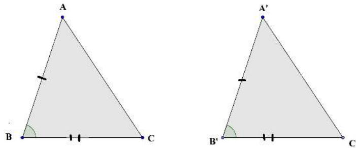
Figura 1.10: Caso LAL
