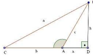
Figura 3.4: \hat{A} > 90^\circ
