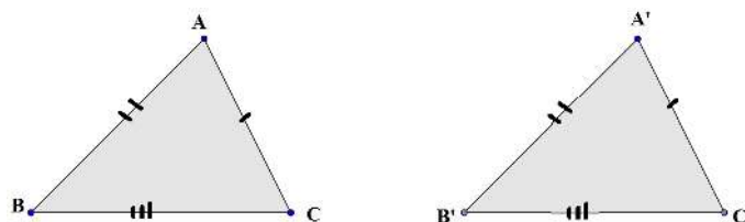
Figura 1.9: Caso LLL
