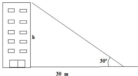
Figura 4.2: Exemplo 4.1
