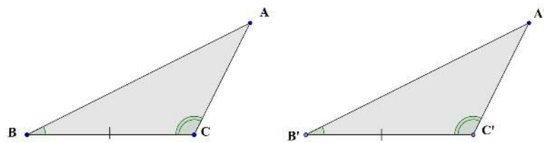
Figura 1.11: Caso ALA
