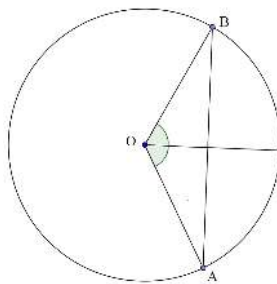
Figura 2.1: comprimento da corda
