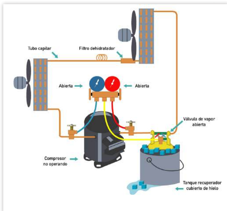
Recuperación de vapor cuando el compresor está operando
