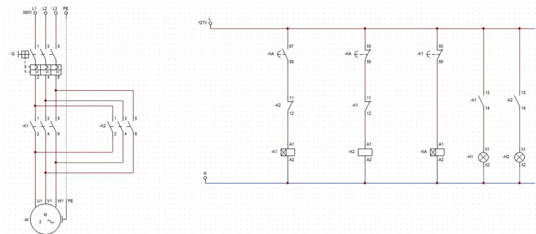
Figura 4: Partida reversão de motor com temporização.
