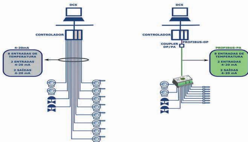
Figure 3: Funcionamento de um sistema multiponto
