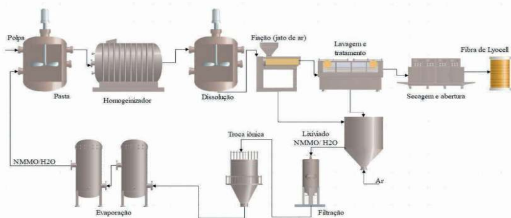
Figura 2. Processo de liocel baseado em NMMO
