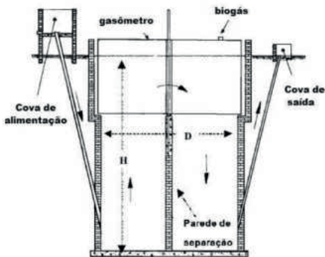
Figura 2 - Biodigestor bifásico.
