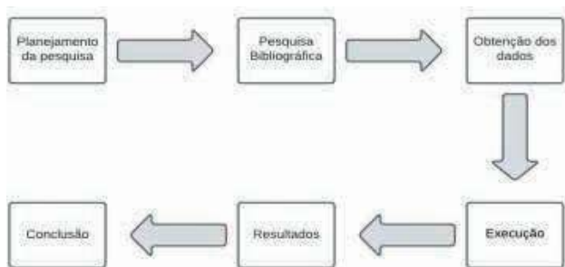
Figura 3 - Fluxograma metodológico.
