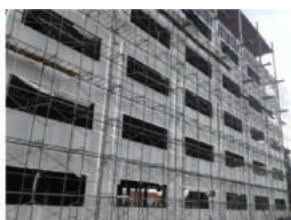
Figura 45: Fachada em light steel framing com vedaç o em Placas Ciment cias (Fonte: Saint-Gobain)
