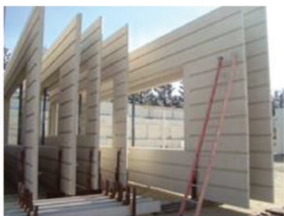
Figura 1: Painéis de vedação pré-fabricados de concreto (Fonte: ABCIC)
