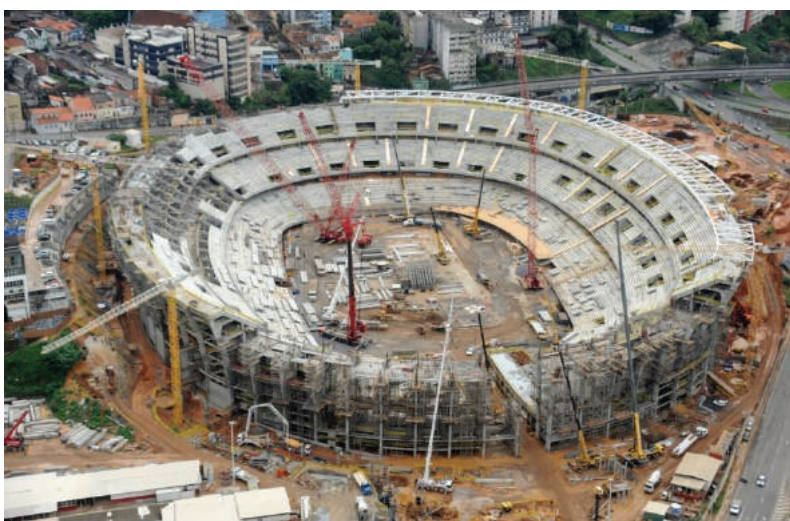
Figura 63: Estádio Arena Fonte Nova durante a montagem da estrutura pré-moldada
