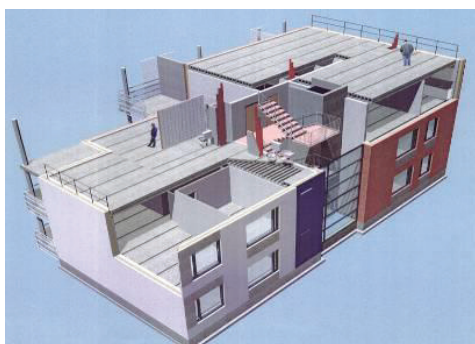
Figura 75: Sistema estrutural com painéis portantes e lajes alveolares protendidas (Fonte: FIB, CEB-FIP, 2002)
