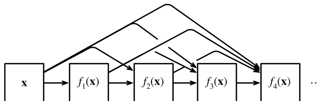
Fig. 7.7.2: Conexões densas na DenseNet.
