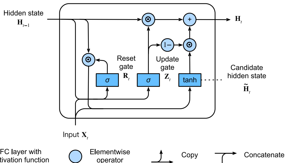
Fig. 9.1.3: Computing the hidden state in a GRU model. Calculando o estado oculto em um modelo GRU.
