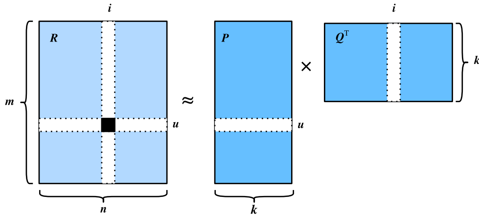
Fig. 16.3.1: Ilustração do modelo de fatoração de matriz
