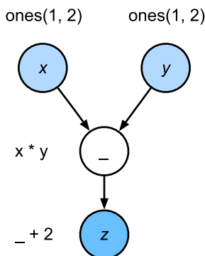
Fig. 12.2.2: Dependências.
