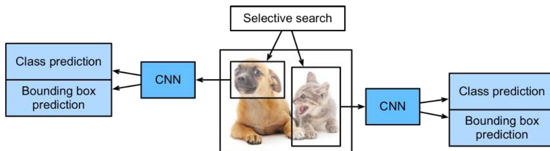
Fig. 13.8.1: Modelo R-CNN.
