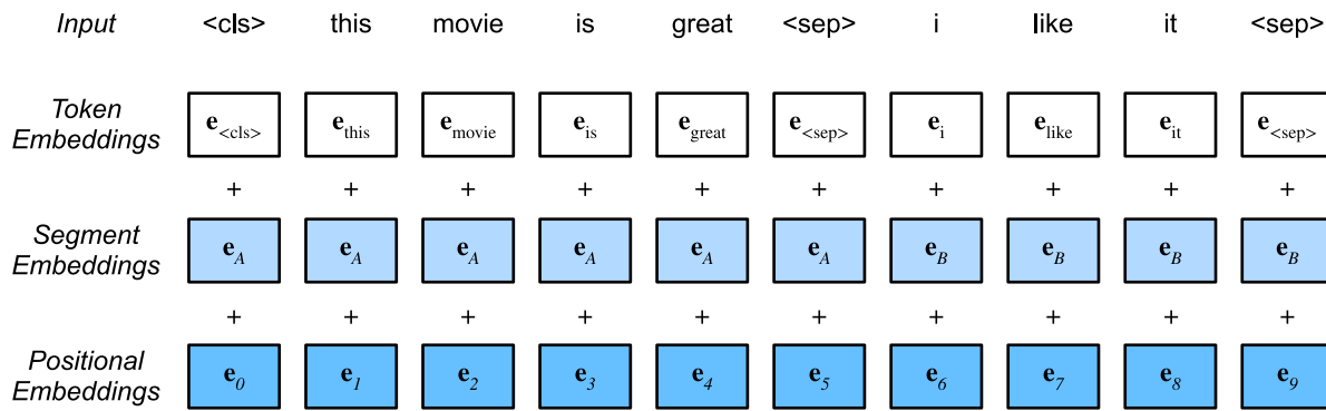
Fig. 14.8.2: Os embeddings da sequência de entrada de BERT são a soma dos embeddings de token, embeddings de segmento e embeddings posicionais.
