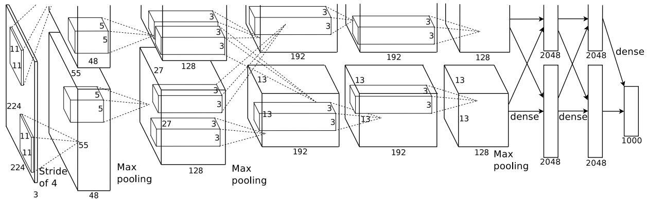
Fig. 12.5.1: Paralelismo de modelo no design AlexNet original devido à memória GPU limitada.
