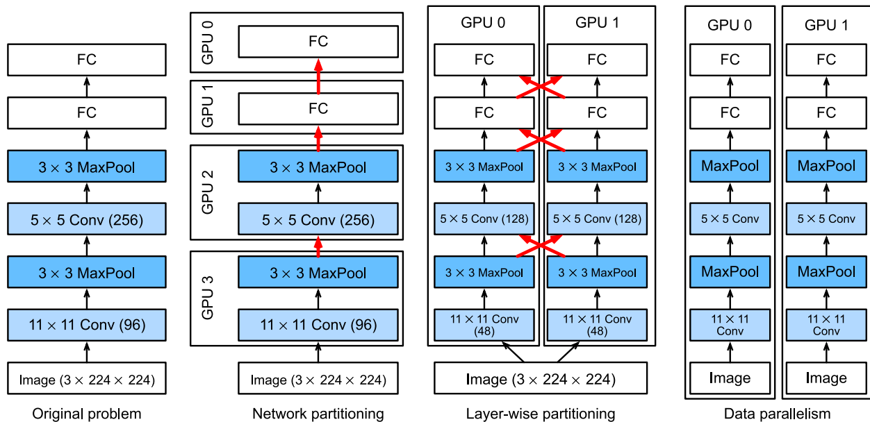
Fig. 12.5.3: Paralelização em várias GPUs. Da esquerda para a direita - problema original, particionamento de rede, particionamento de camada, paralelismo de dados.
