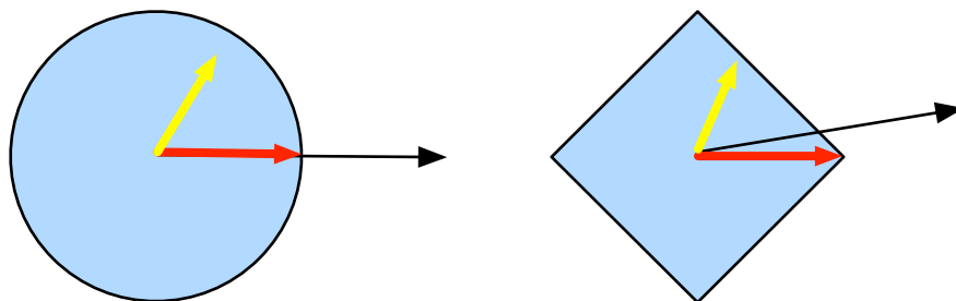
Fig. 11.2.4: Projeções convexas.
