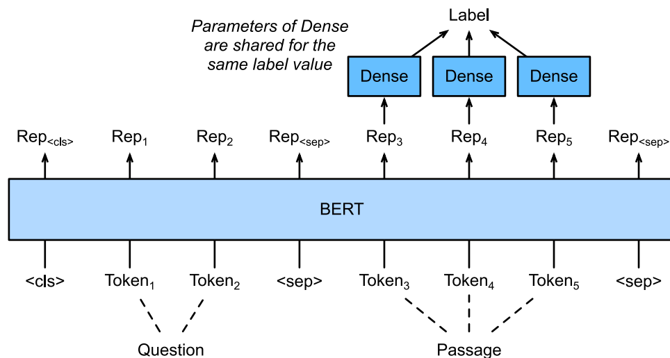
Fig. 15.6.4: Ajuste fino do BERT para resposta a perguntas. Suponha que o par de texto de entrada tenha dois e três tokens .
