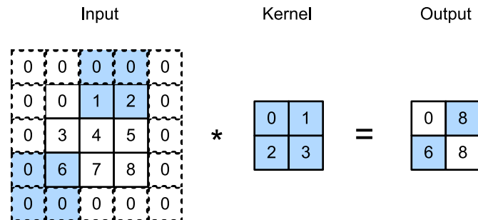
Fig. 6.3.2: Correlação cruzada com passos de 3 e 2 para altura e largura, respectivamente.
