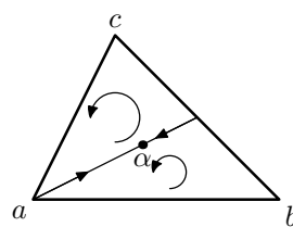
Figura 2.5: Caso 4
