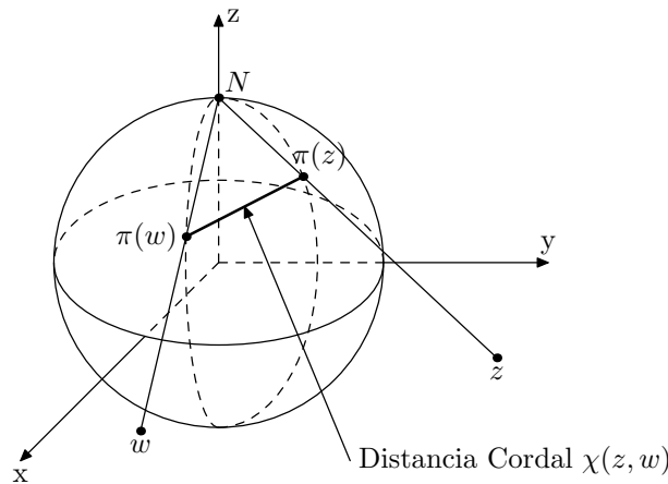
Figura 5.1: Proyección estereográfica
