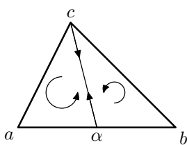
Figura 2.4: Caso 3
