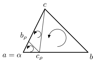
Figura 2.3: Caso 2
