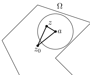
Figura 2.2: Dominio estrellado
