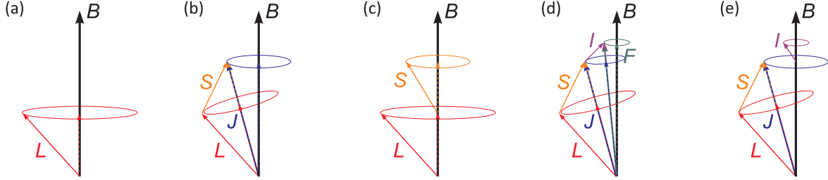
Figura 6.2: Acoplamento dos momentos angulares para o efeito (a) Zeeman normal, (b) Zeeman anormal, (c) Paschen-Back, (d) Zeeman da estrutura hiperfina e (e) Paschen-Goudsmith.
