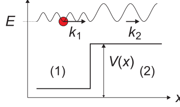
Figura 2.2: Esquema de um potencial com várias seções de profundidades constantes.
