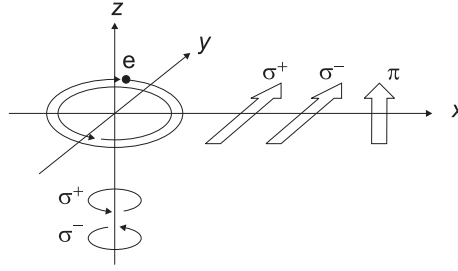
Figura 6.4: Descrição clássica do efeito Zeeman normal.
