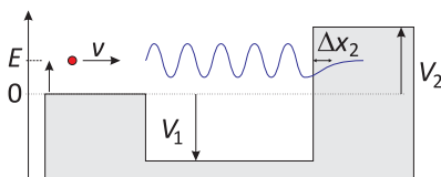
Figura 2.9: Partícula num paisagem de potencial.
