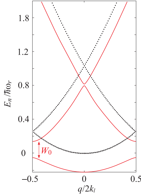
Figura 8.1: (Linha vermelha contínua) Bandas de Bloch. (Linha preta pontilhada) Sem potencial, V_0 = 0 . Os parâmetros são \omega_r = (2\pi) 20 kHz, \omega_{ho} = (2\pi) 12 kHz, \lambda_L = 689 nm e V_0 = 0.2\hbar\omega_r .
