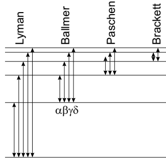
Figura 3.4: As transições do hidrogênio.
