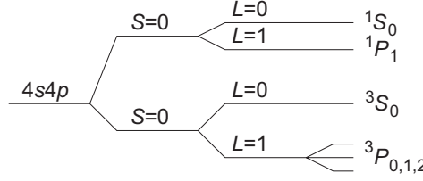
Figura 6.3: Acoplamento spin-órbita.
