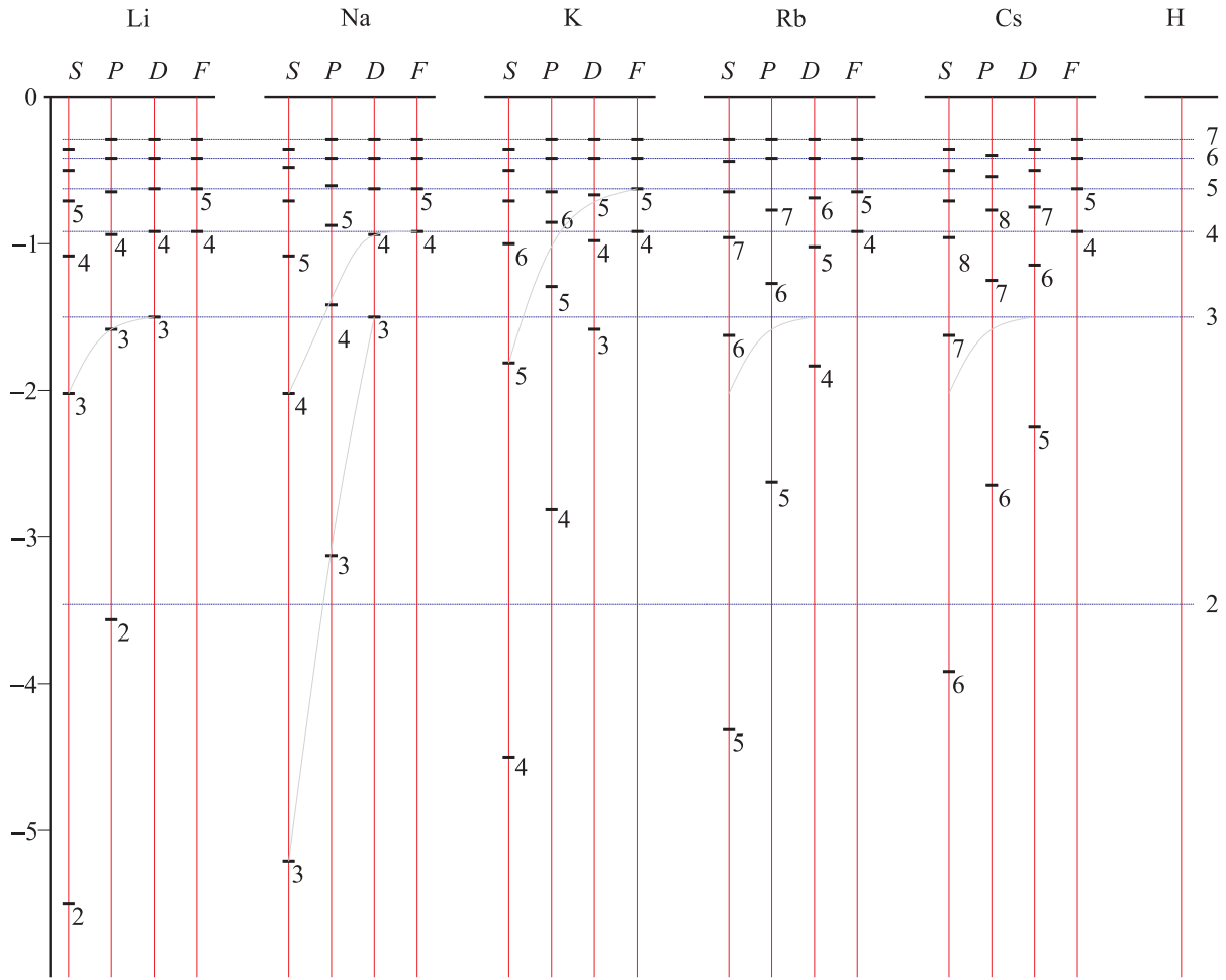
Figura 7.3: Comparação das energias de excitação do elétron de valência para vários átomos alcalinos.
