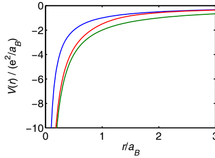
Figura 7.2: Potenciais coulombiano, blindado e efetivo.
