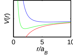
Figura 3.3: (Code: AM_Hidrogenoido_Centrifugal.m) Soma de um potencial coulombiano e um potencial centrífuga para \ell = 0 (vermelho), \ell = 1 (verde) e \ell = 2 (azul).
