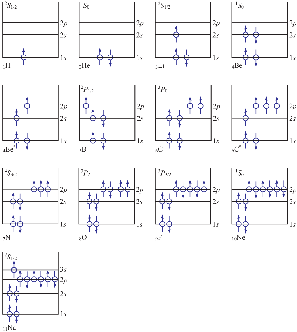
Figura 7.4: A regra de Hund.
