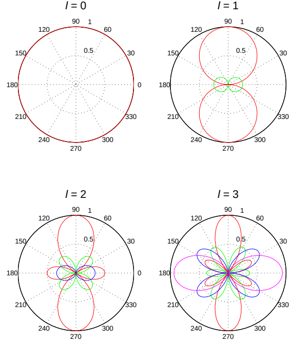
Figura 3.2: (Code: AM_Hidrogenoido_Legendre.m) Funções de onda angulares. Mostradas são os polinômios de Legendre P_\ell^m(\cos \vartheta) para \ell = 0, 1, 2, 3 e m = 0, \dots, \ell .
