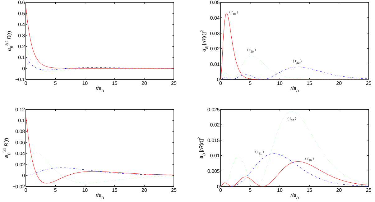
Figura 3.6: (Code: AM_Hidrogenoido_Laguerre.m) Funções de onda radiais, esquerda R ; direita u . Acima para (n, \ell) = (1..3, 0) ; embaixo (n, \ell) = (3, 0..2) .
