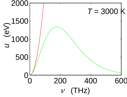
Figura 5.2: Curvas de Rayleigh-Jeans e de Einstein.
