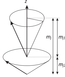
Figura 4.2: Ilustração do acoplamento de dois momentos angulares.
