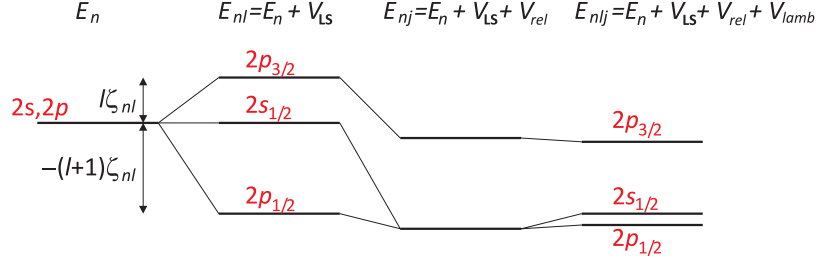
Figura 6.1: Níveis do hidrogênio.
