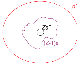
Figura 3.1: O modelo do hidrogênio se aplica em outros átomos desde que eles têm um elétron de valência ocupando um espaço tão grande que ele está vendo o núcleo e o resto dos elétrons blindando o núcleo como uma única carga positiva.
