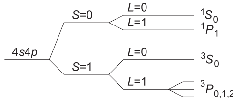
Figura 4.3: Exemplo para o acoplamento spin-órbita \mathbf{L} \cdot \mathbf{S} para dois elétrons.
