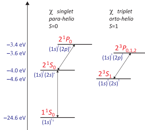
Figura 7.1: Níveis do hélio. Note que o estado (1s)^{\uparrow\uparrow} não existe.
