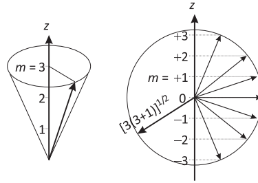
Figura 4.1: Ilustração do momento angular na mecânica quântica.
