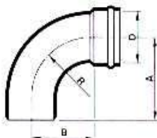
curva 90° curta
