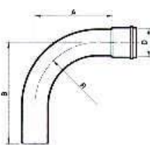
curva 90° longa
