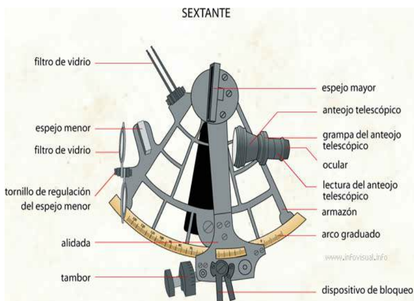
Ilustración 8. Sextante. Fuente: www.infovisual.info
