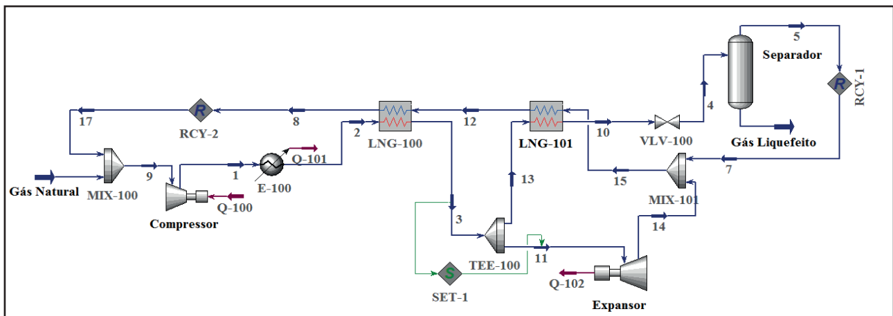
Figura 8. Fluxograma da simulação do processo de liquefação do gás natural elaborado com o Aspen Hysys neste trabalho.
