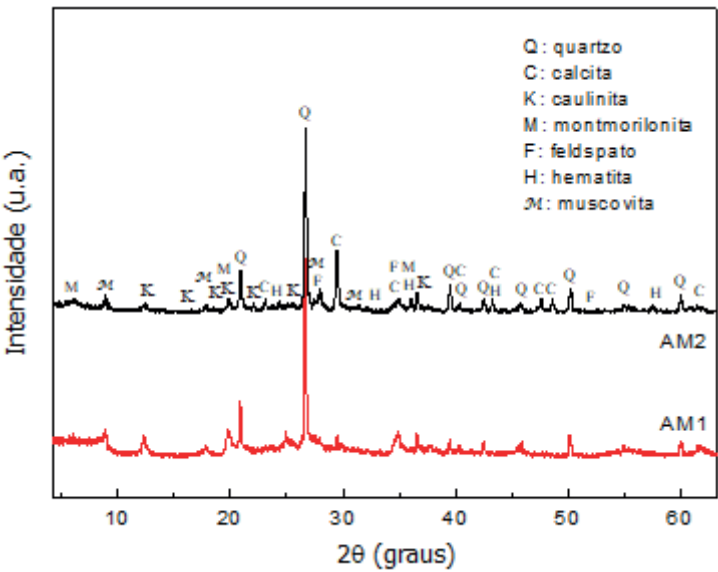
Figura 2. Padrões de difração de raios X das amostras e seus respectivos minerais.
