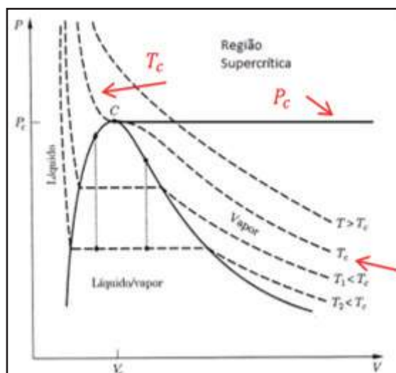
Figura 1. Diagrama PVT genérico de uma substância pura.
