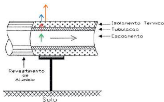
Figura 1. Processos de transferência de calor nas linhas de injeção aéreas.
