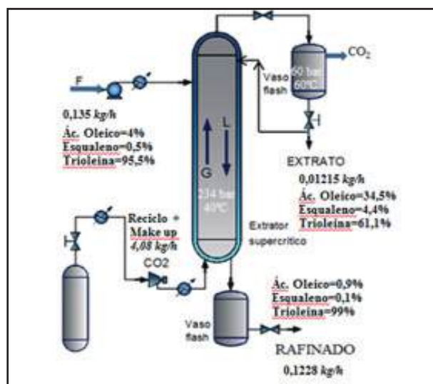
Figura 11. Representação esquemática da simulação do processo de extração supercrítica em coluna de multiestágios em contracorrente de FORNARI et al. (2007).
