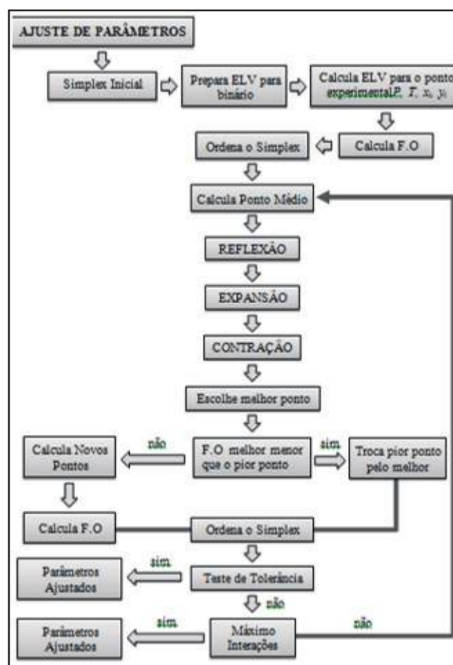
Figura 3. Ajuste de parâmetros pelo Método Simplex (EDEflash).
