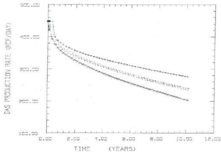
Figura 4. Efeito do coeficiente de compactação da rocha-matriz na produção de gás do aquífero Sweet Lake .
