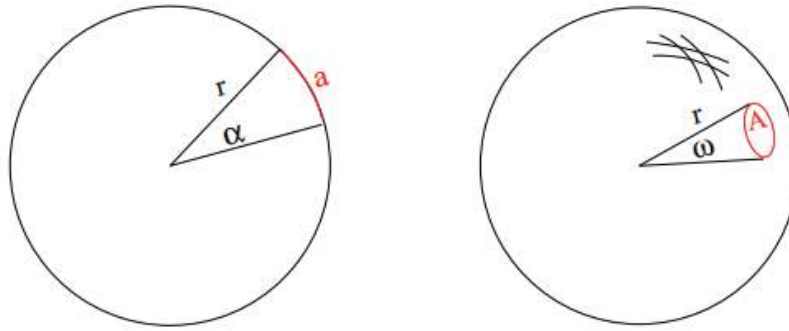
Figura 3. Representação de um ângulo plano e um ângulo sólido. Outra definição de I_\lambda é a energia por unidade de área, \lambda , de tempo e de ângulo sólido.
