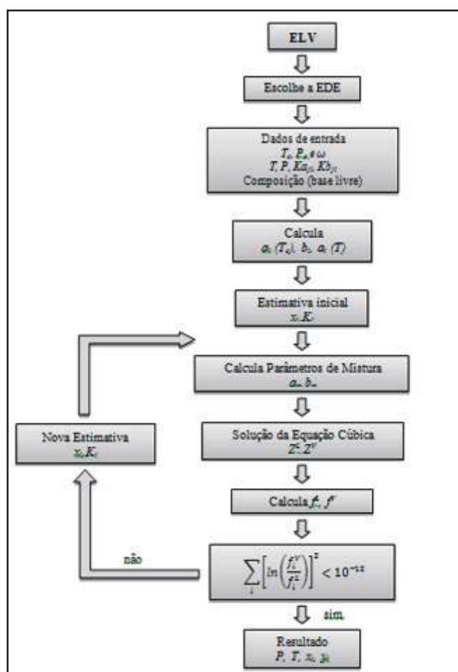
Figura 2. Cálculo do Equilíbrio Líquido-Vapor com as Equações de Estado (EDEflash).
