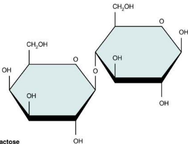
Lactose
