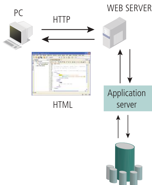
Figura 3.1: Imagem ilustrativa do funcionamento do protocolo HTTP
