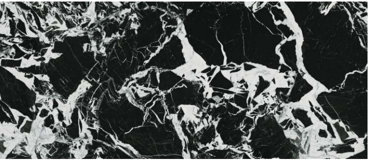
Black Breccia
