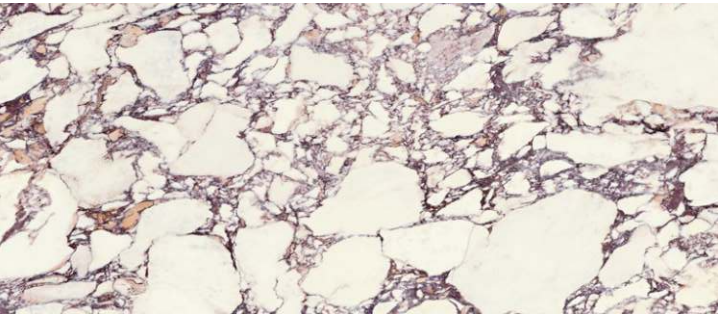
Breccia
