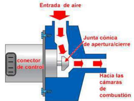
Flujo de aire controlado por la válvula IAC
