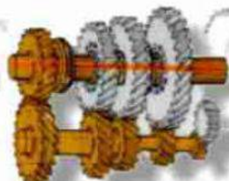
CUARTA VELOCIDAD
