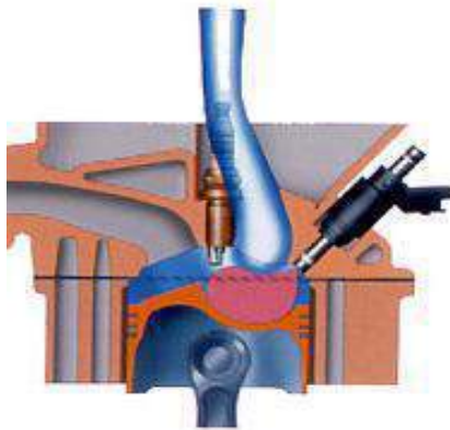
Inyección directa
