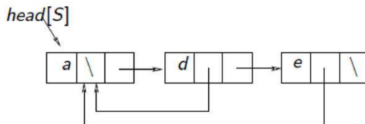
Figura 18: Estrutura de lista encadeada Fonte: www.das.ufsc.br consultado em 10/02/2016
