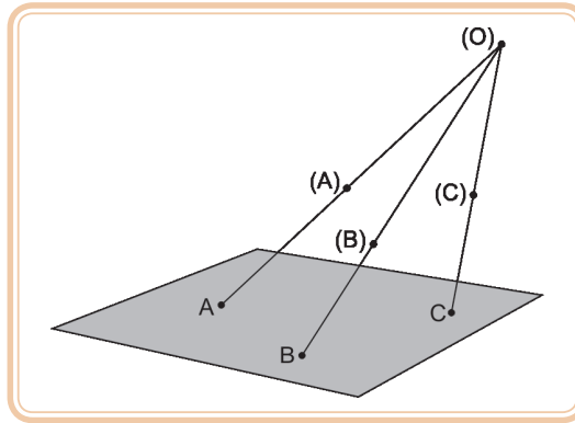
Figura 8.2: Projeção cônica ou central
