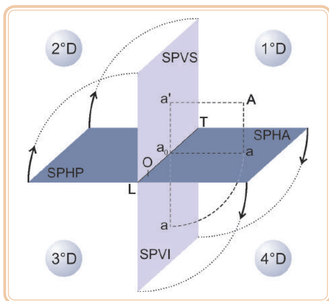
Figura 4.1: Perspectiva da representação de um ponto
