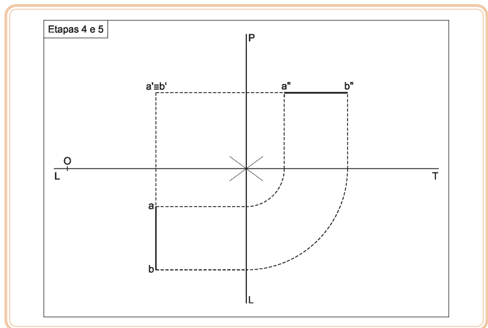
Figura 4.18: Transferência de valores para LT
