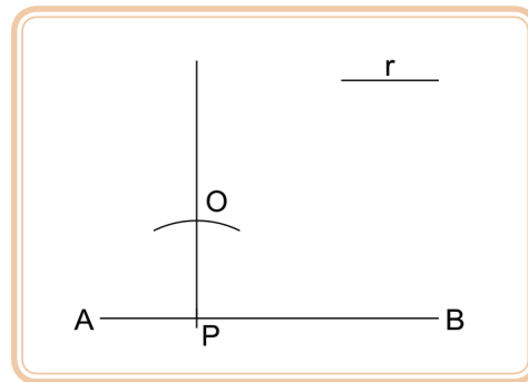
Figura 3.38: Definição do centro do arco de concordância
