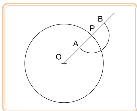
Figura 3.30: Arco para definição dos pontos A e B
