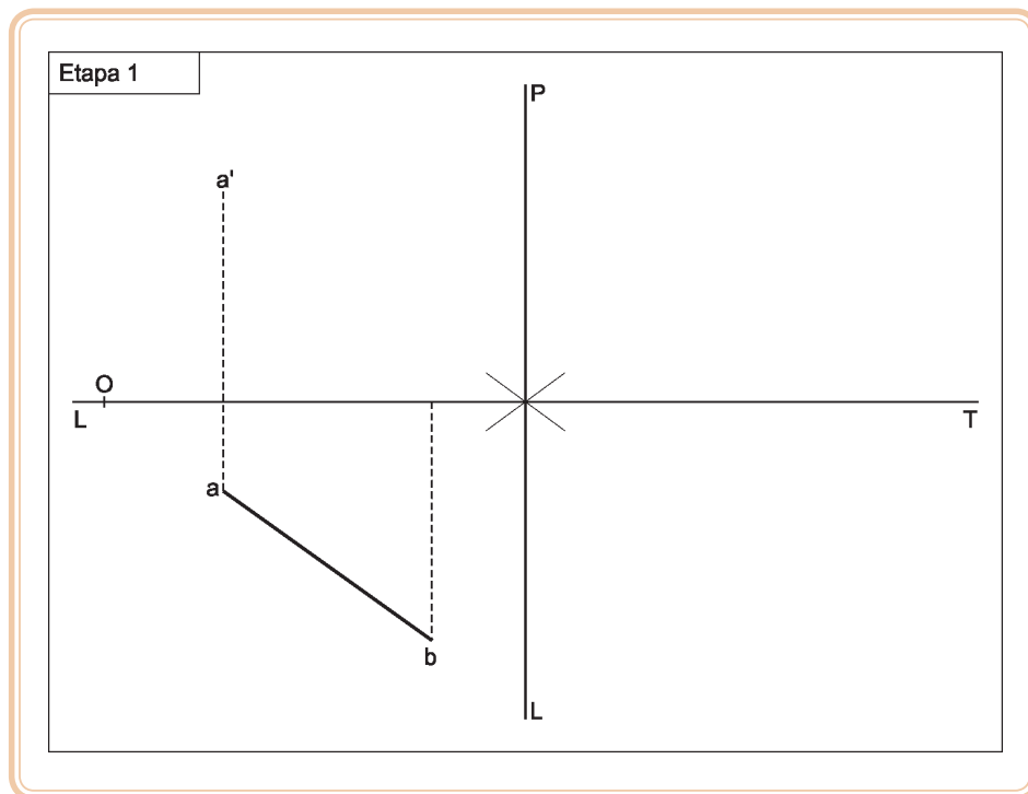
Figura 5.35: Projeção dos pontos
