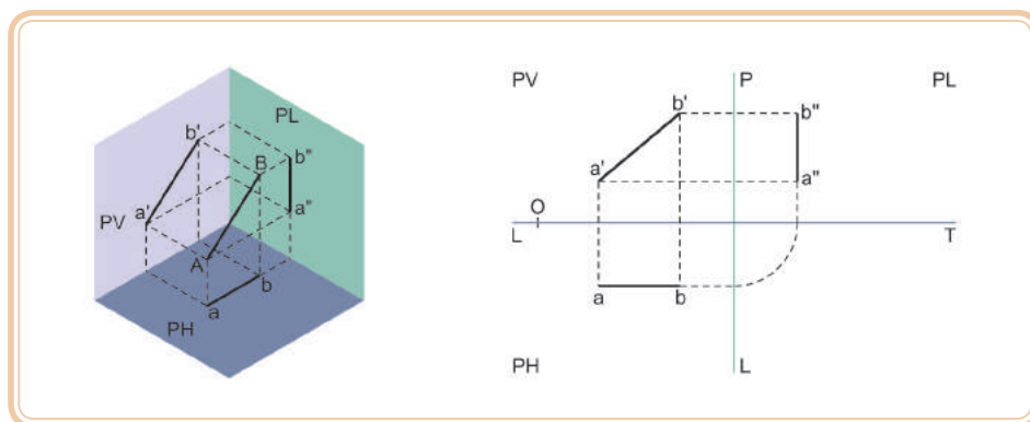
Figura 4.12: Reta frontal
