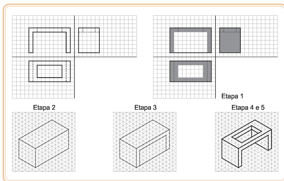
Figura 8.9: Execução de perspectiva isométrica
