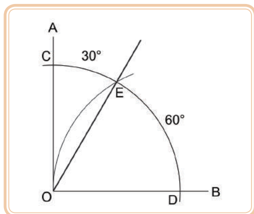
Figura 2.50: Determinação dos ângulos de 30^\circ e 60^\circ
