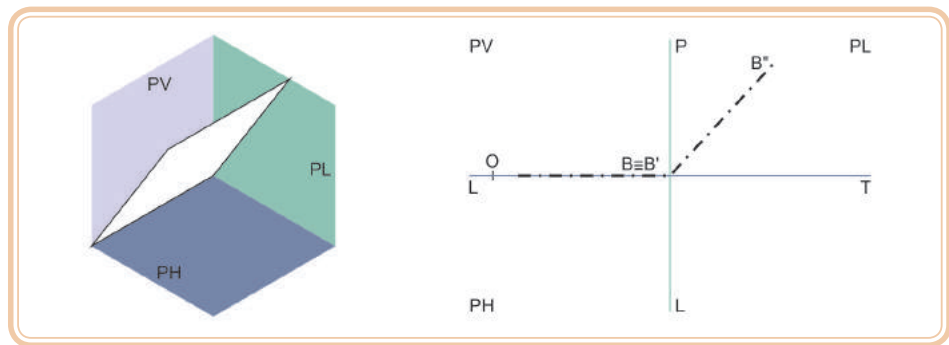
Figura 5.9: Plano que passa pela LT
