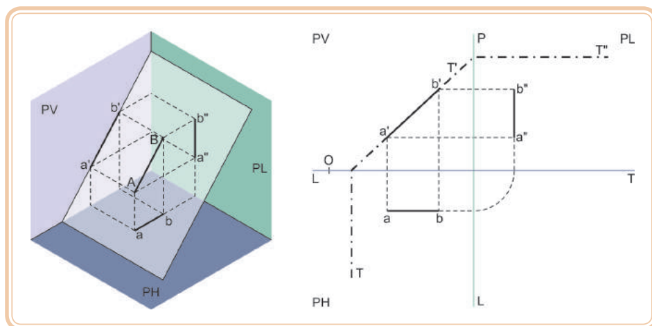
Figura 5.11: Plano de topo – reta frontal
