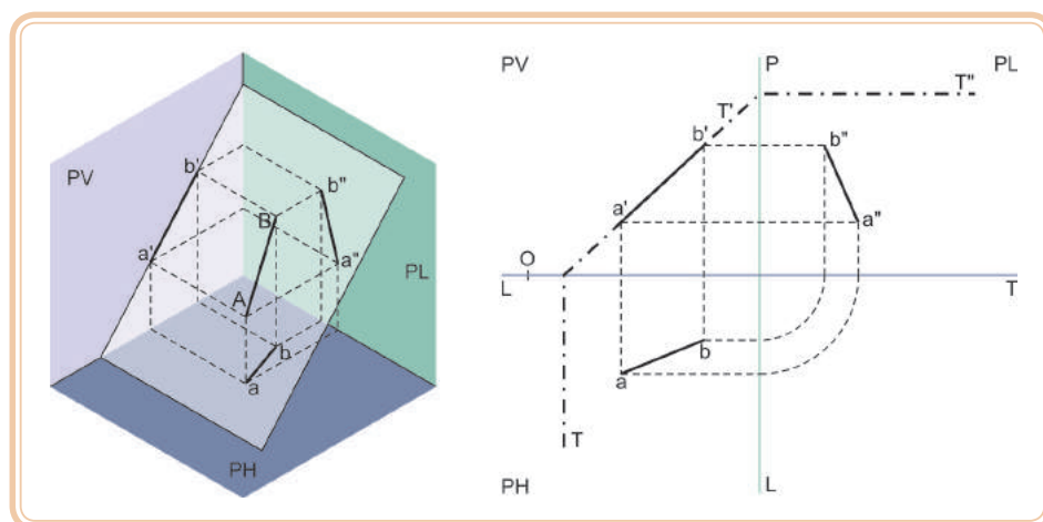
Figura 5.12: Plano de topo – reta oblíqua
