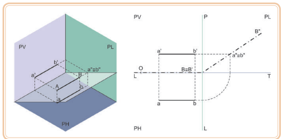
Figura 5.30: Plano que passa pela LT – reta fronto-horizontal
