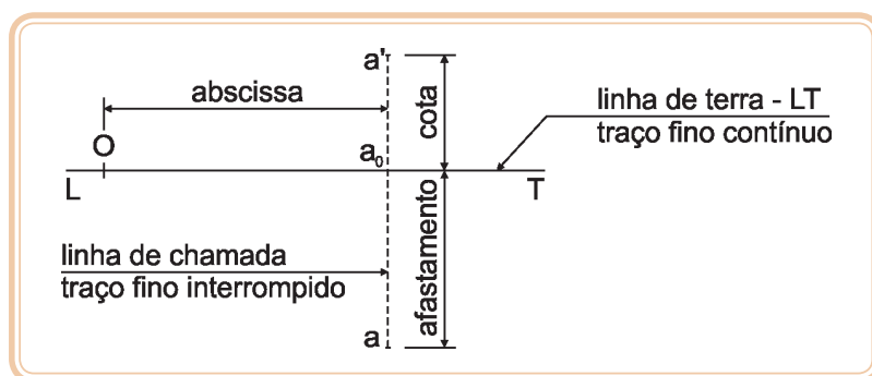
Figura 4.3: Dimensões espaciais relacionadas ao ponto
