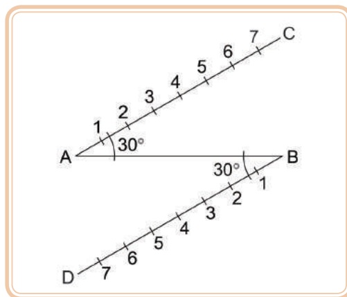
Figura 2.34: Divisão das retas em segmentos
