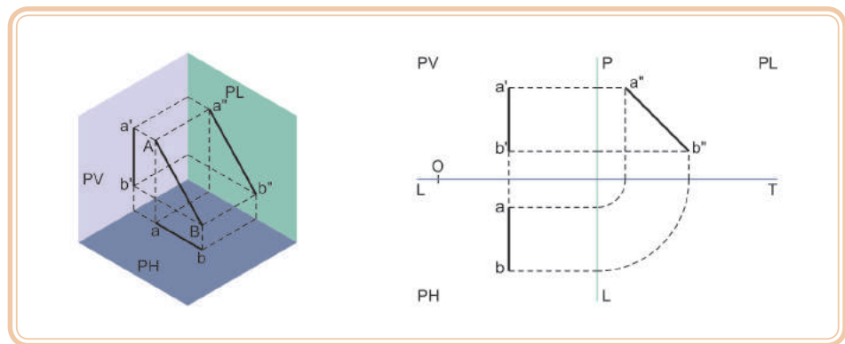
Figura 4.14: Reta de perfil
