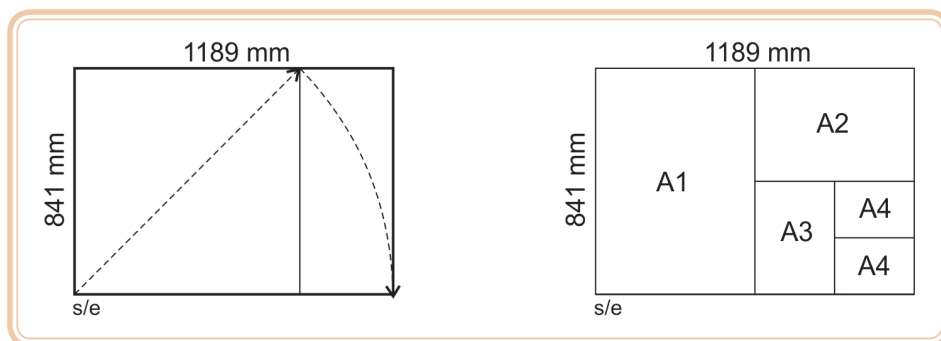
Figura 1.12: Obtenção dos formatos da série A
