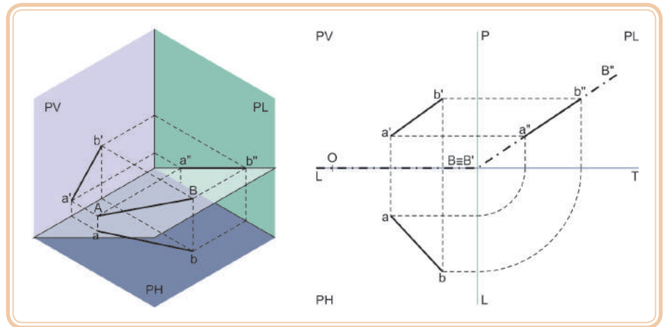
Figura 5.29: Plano que passa pela LT – reta oblíqua
