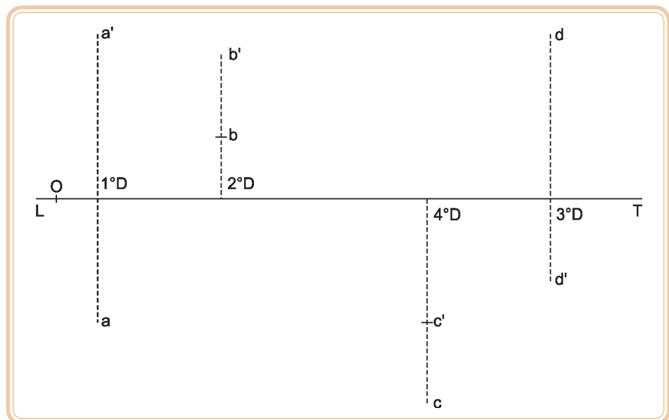
Figura 4.5: Representação de ponto em épura
