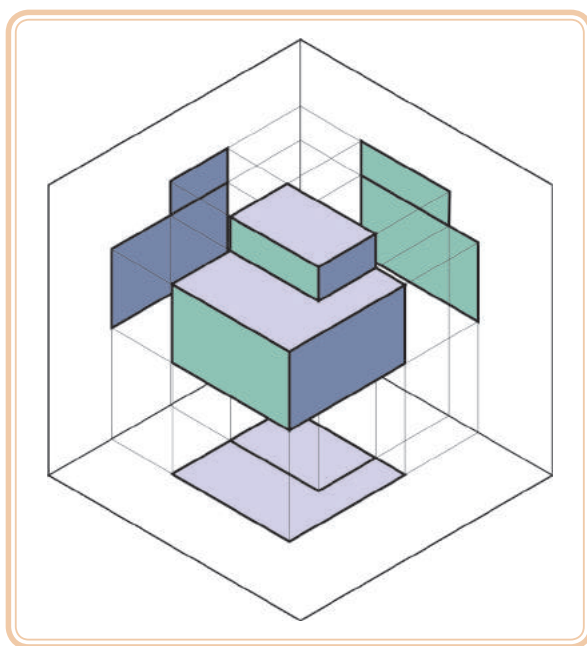
Figura 7.1: Vistas ortográficas
