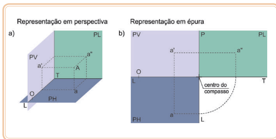
Figura 4.6: Projeção no plano lateral: (a) representação em perspectiva e (b) representação em écura
