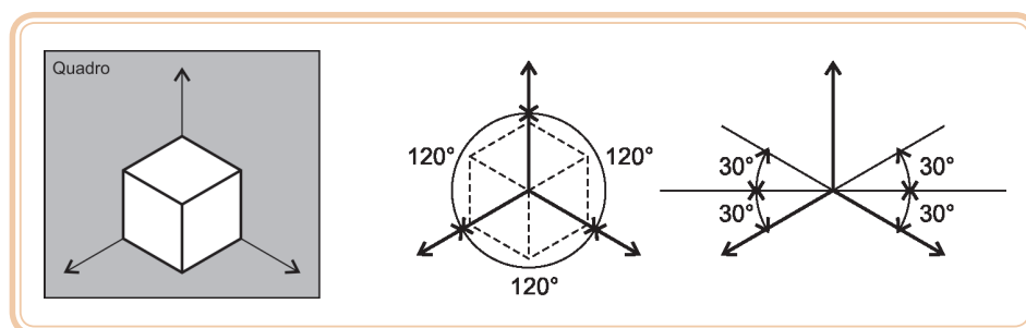
Figura 8.8: Perspectiva isométrica
