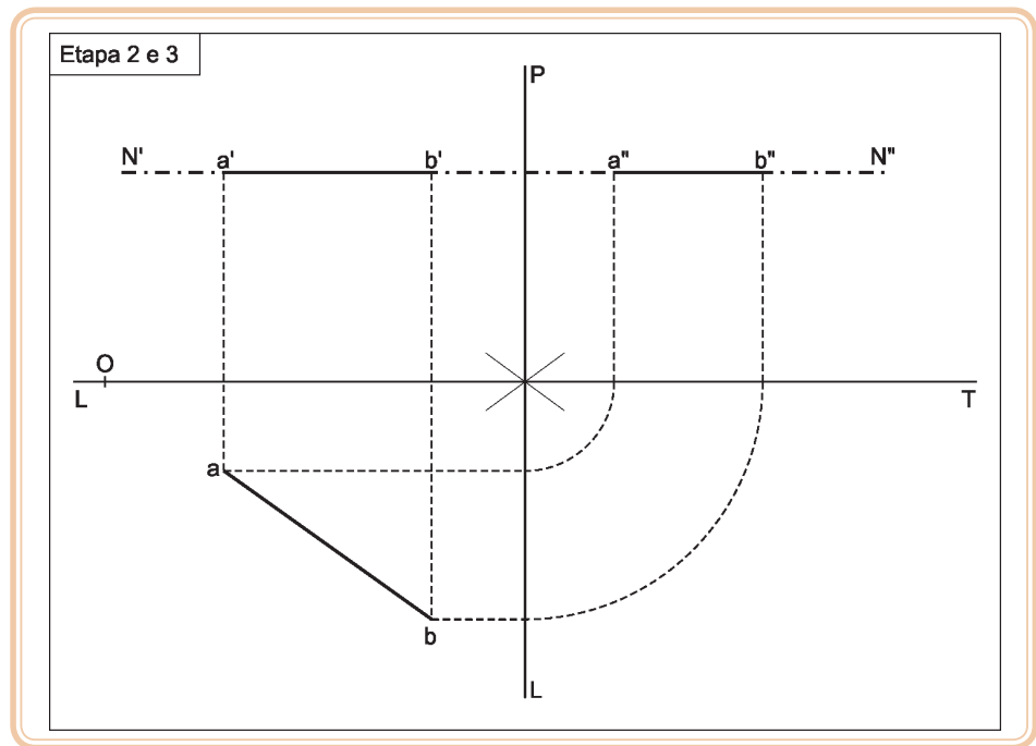
Figura 5.36: Representação do plano de nível
