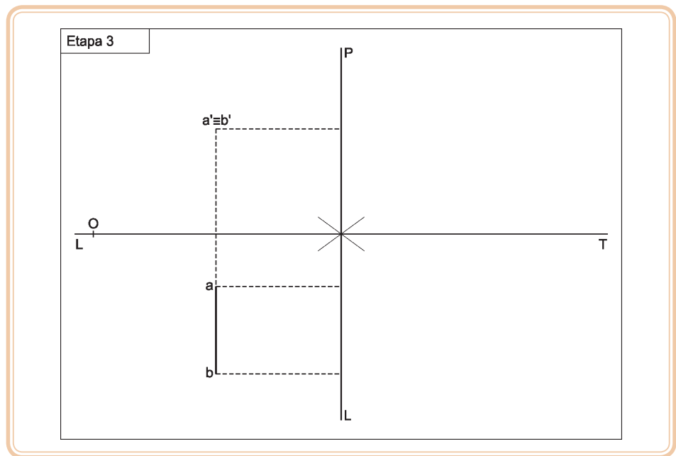
Figura 4.17: Transferência de valores para PL
