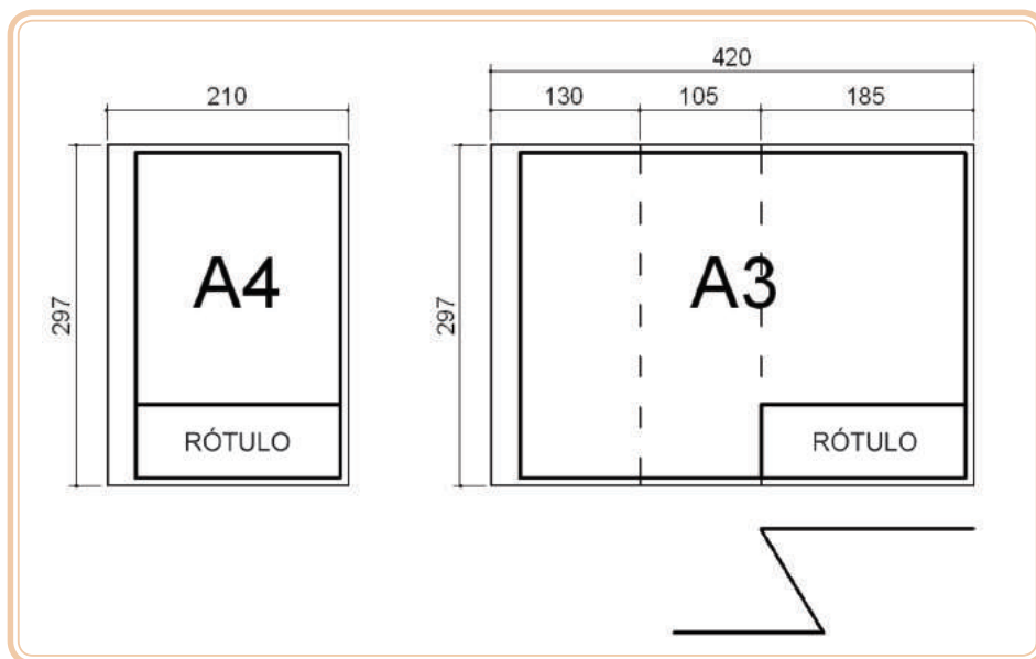
Figura 1.13: Dobramento de folhas A4 e A3
