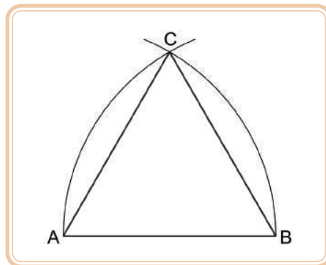
Figura 3.7: Traçado do triângulo equilátero
