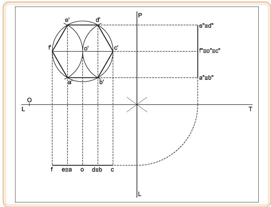
Figura 5.38: Definição das outras projeções no PH e no PL
