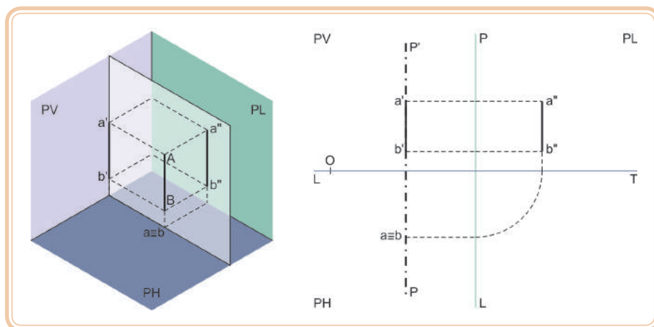
Figura 5.27: Plano de perfil – reta vertical
