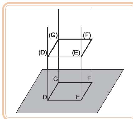
Figura 8.4: Projeção cilíndrico-ortogonal
