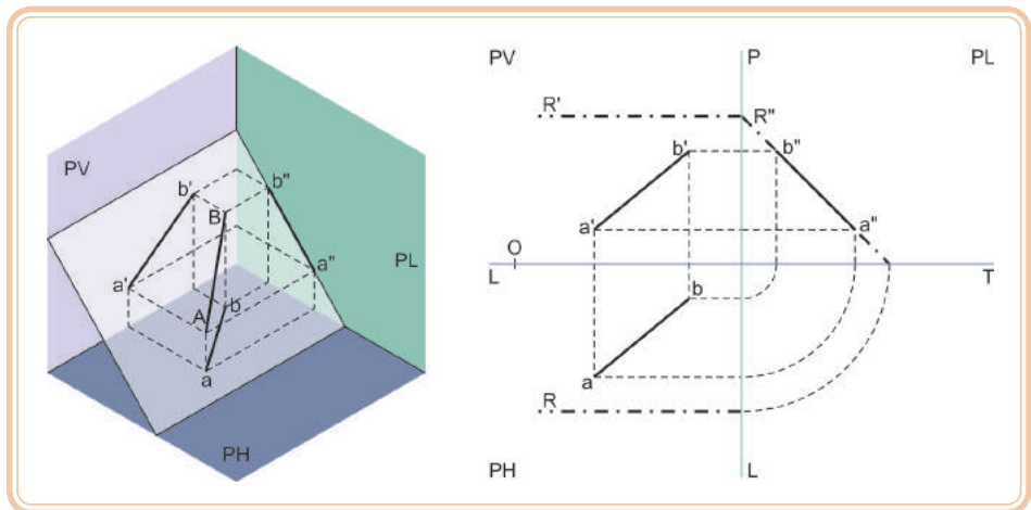
Figura 5.18: Plano de rampa – reta oblíqua
