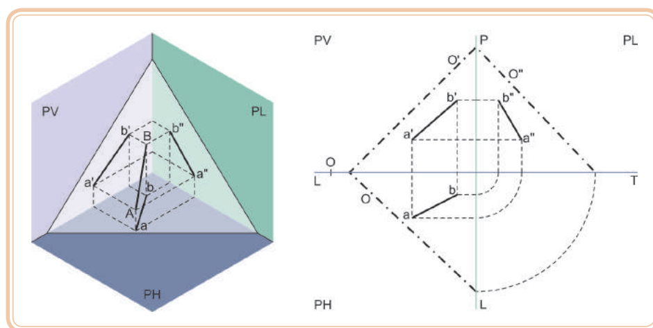
Figura 5.31: Plano oblíquo – reta oblíqua
