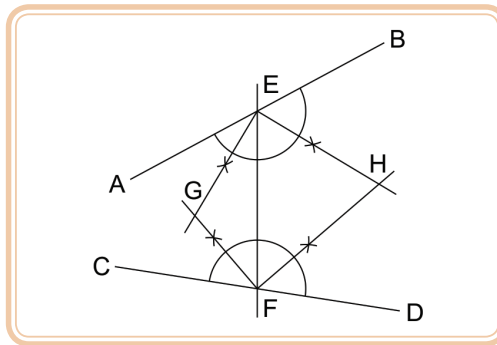
Figura 2.42: Traçado de bissetrizes para definir os pontos G e H
