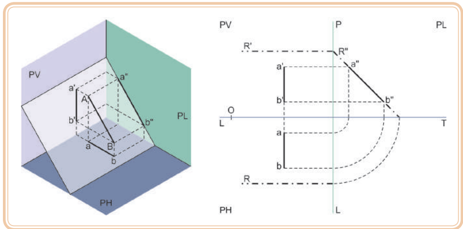
Figura 5.17: Plano de rampa – reta de perfil
