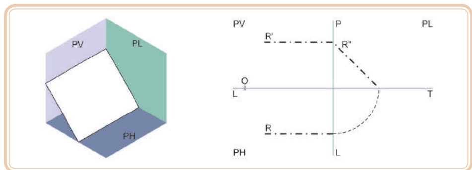
Figura 5.4: Plano de rampa
