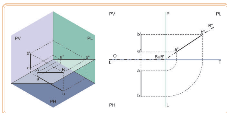
Figura 5.28: Plano que passa pela LT – reta de perfil
