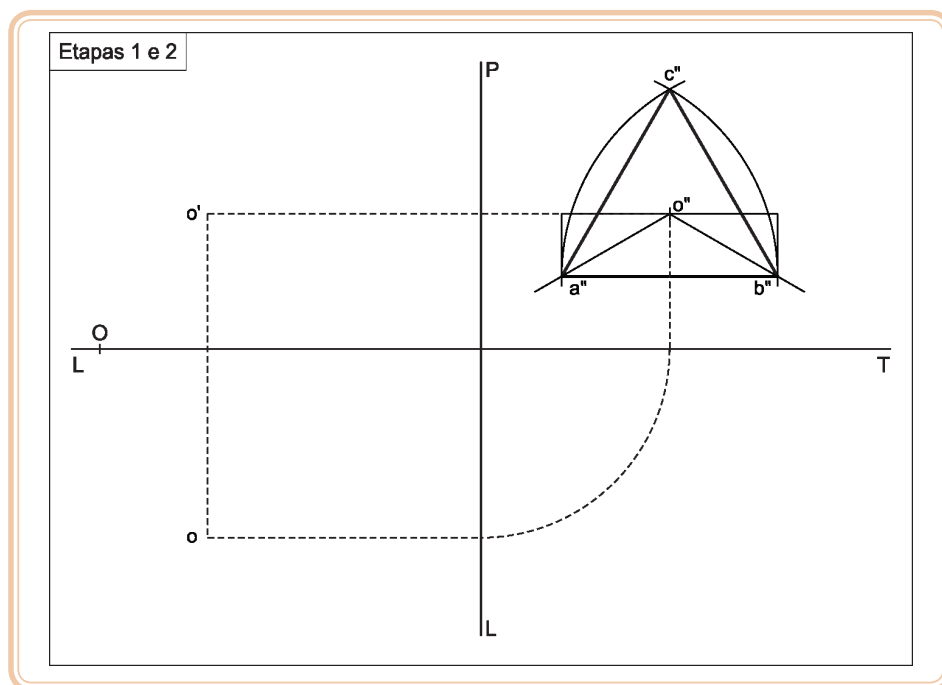
Figura 6.10: Coordenadas do centro da figura e traçado do triângulo equilátero
