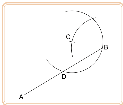
Figura 2.22: Arco que passa em B e corta o segmento AB
