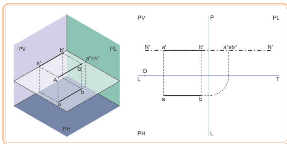
Figura 5.23: Plano de nível – reta fronto-horizontal
