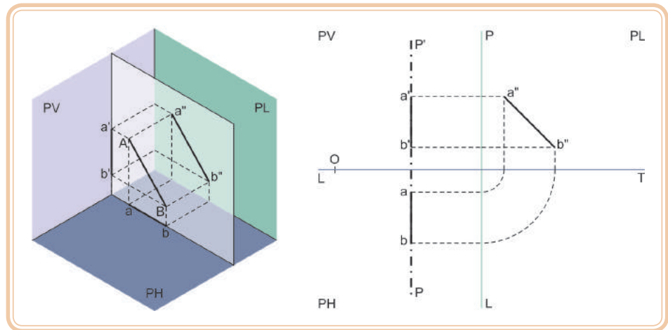
Figura 5.25: Plano de perfil – reta de perfil
