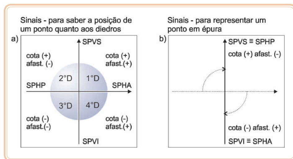
Figura 4.4: Convenções: (a) sinais – para saber a posição de um ponto quanto aos diedros e (b) sinais – para representar um ponto em épura
