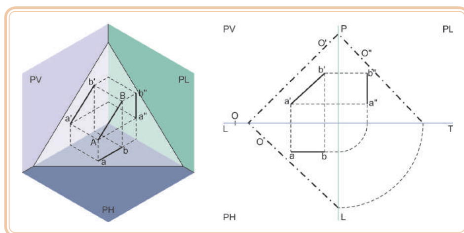
Figura 5.32: Plano oblíquo – reta frontal
