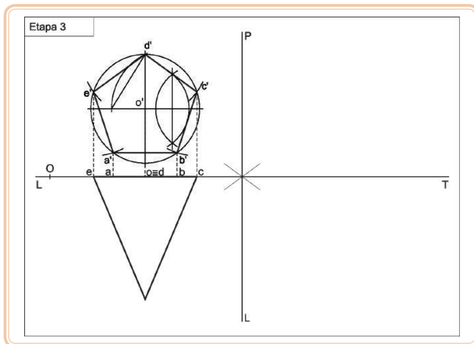
Figura 6.8: Traçado do contorno aparente da projeção no PH Fonte: autor
