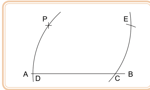
Figura 2.30: Arco com centro em C e mesmo raio
