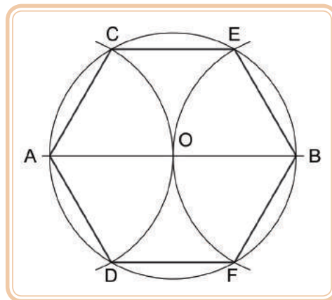
Figura 3.27: Traçado do hexágono regular
