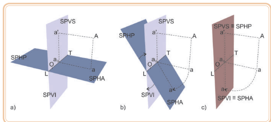
Figura 4.2: Rebatimento de um ponto: (a) perspectiva – projeção do ponto; (b) rebatimento do plano horizontal sobre o vertical e (c) planificação
