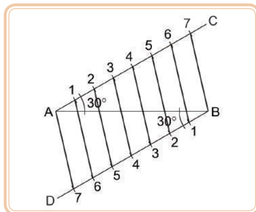
Figura 2.35: Divisão da reta AB em sete partes iguais
