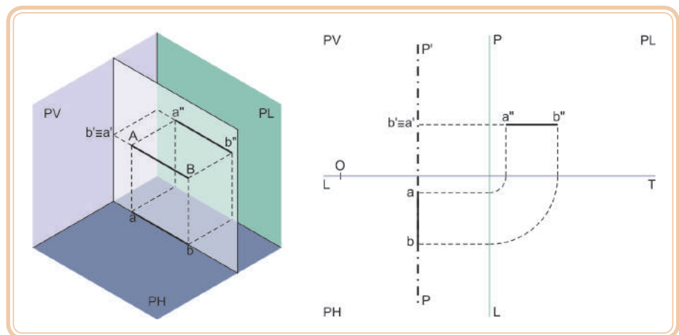
Figura 5.26: Plano de perfil – reta de topo
