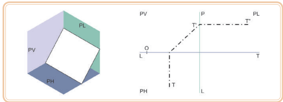
Figura 5.2: Plano de topo
