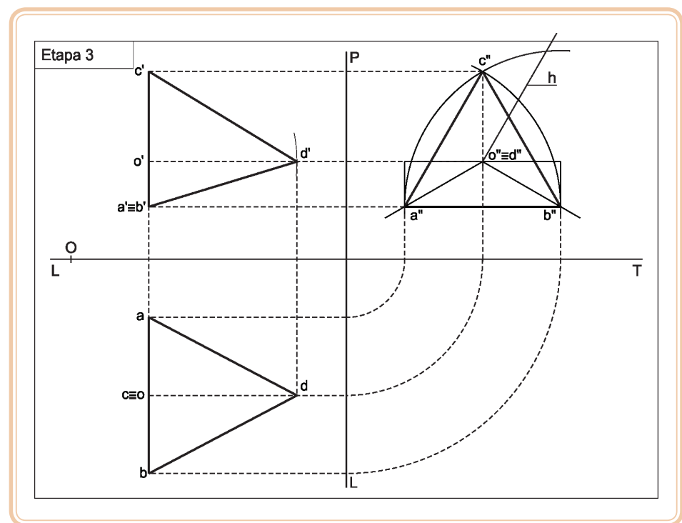
Figura 6.12: Projeção do contorno aparente
