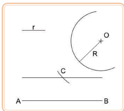
Figura 3.42: Arco com raio R + r que cruze a reta paralela à reta AB
