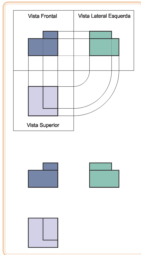
Figura 7.2: Vistas ortográficas frontal, superior e lateral esquerda
