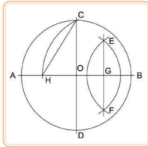
Figura 3.22: Reta CH que define o tamanho do lado do pentágono regular
