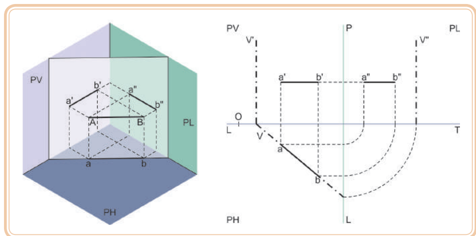
Figura 5.14: Plano vertical – reta de nível
