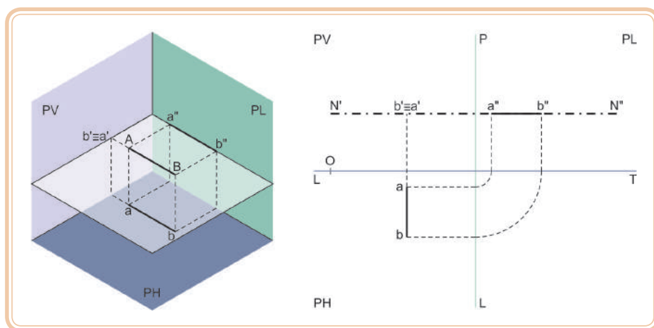
Figura 5.24: Plano de nível – reta de topo
