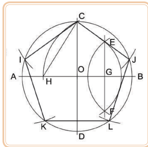
Figura 3.23: Traçado do pentágono regular
