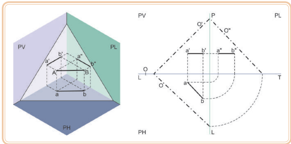
Figura 5.33: Plano obluo – reta de nvel
