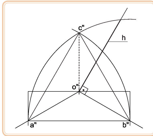
Figura 6.11: Definição da altura do tetraedro
