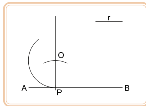
Figura 3.39: Traçado do arco de concordância
