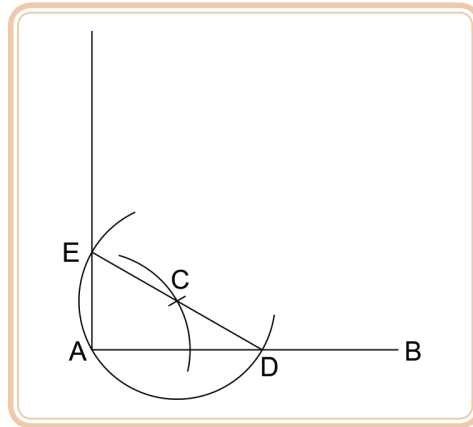
Figura 3.13: Reta perpendicular à reta AB
