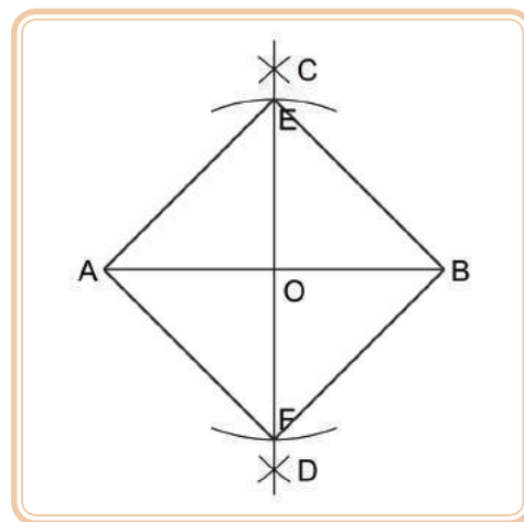
Figura 3.19: Traçado do quadrado
