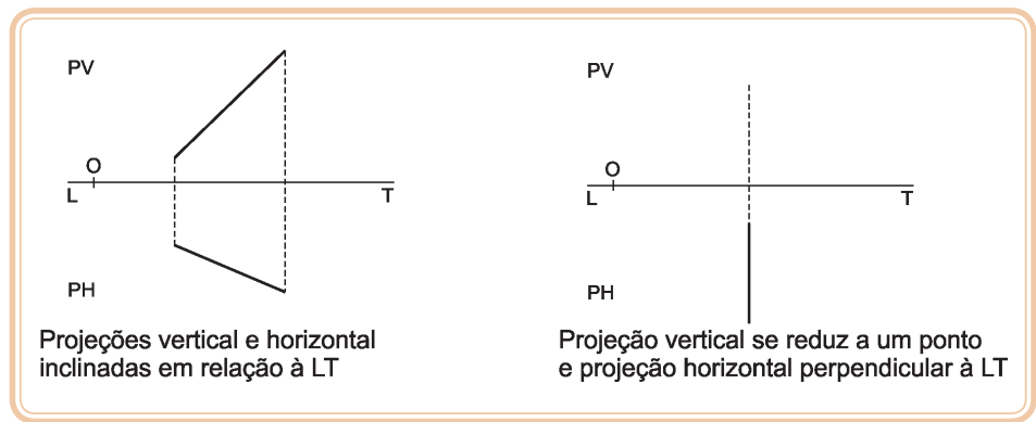
Figura 4.8: Projeção de um segmento de reta em relação à LT
