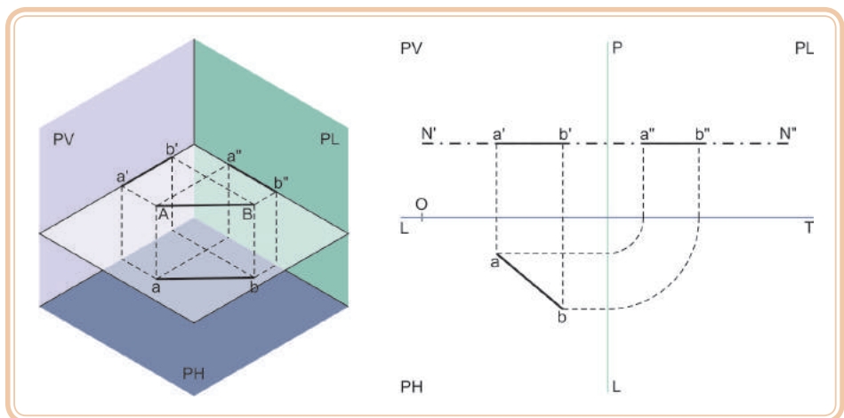
Figura 5.22: Plano de nível – reta de nível
