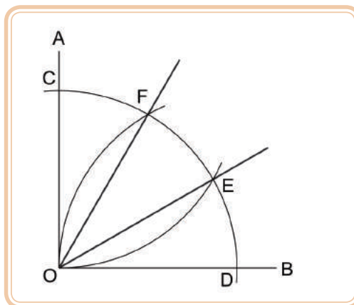
Figura 2.47: Divisão do ângulo reto em três partes iguais Fonte: autor
