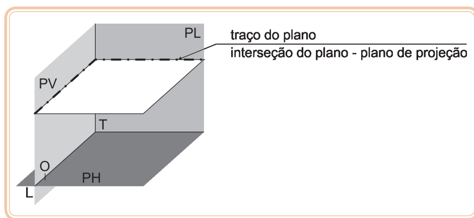
Figura 5.1: Representação dos traços nos planos
