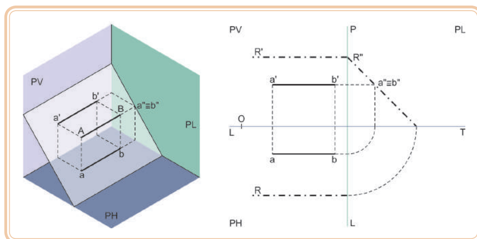
Figura 5.16: Plano de rampa – reta fronto-horizontal
