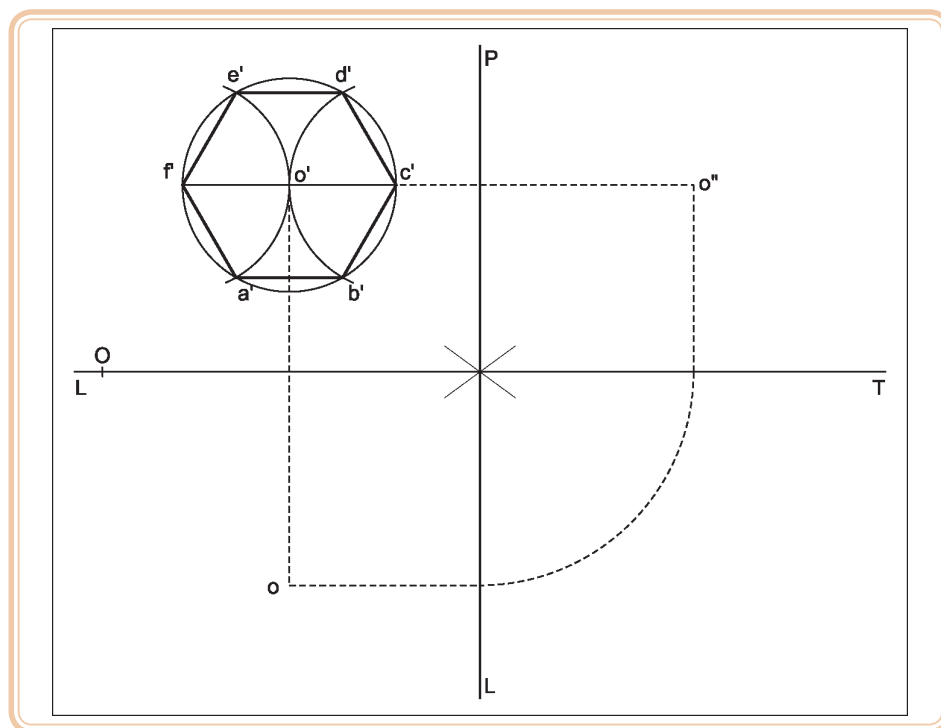
Figura 5.37: Projeções do centro da circunferência e execução do hexágono
