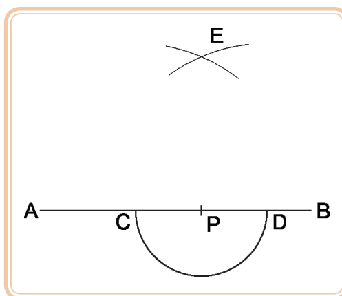
Figura 2.26: Arcos com centro em C e D
