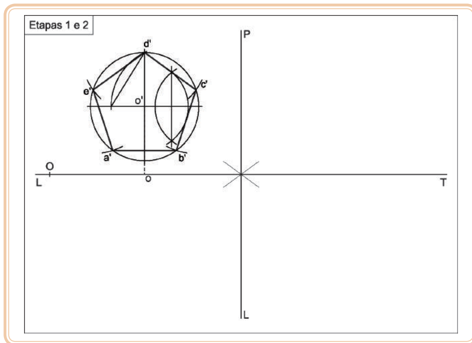
Figura 6.7: Projeção dos pontos e execução do pentágono Fonte: autor
