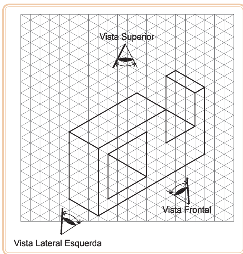
Figura 7.3: Vistas do observador
