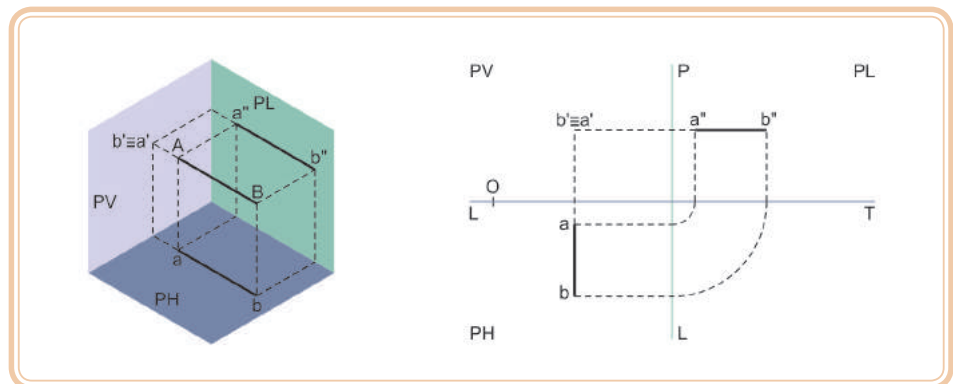
Figura 4.9: Reta de topo
