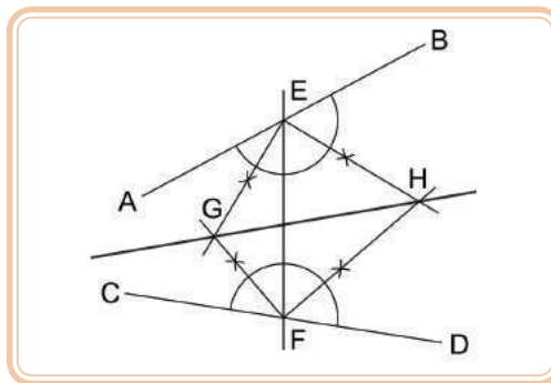
Figura 2.43: Traçado da bissetriz
