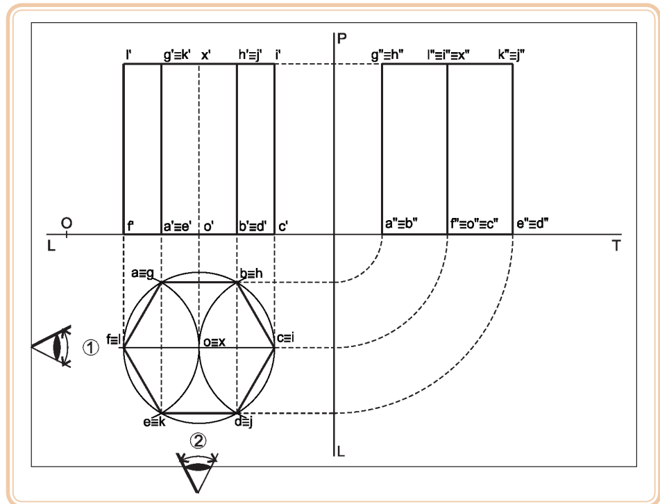
Figura 6.14: Projeções no PL e no PV
