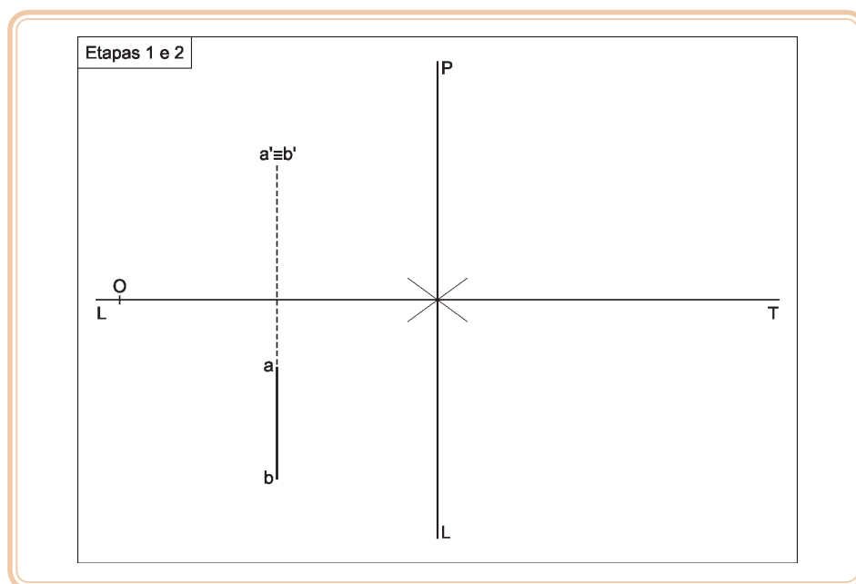
Figura 4.16: Projeção de reta em écura no PV e no PH
