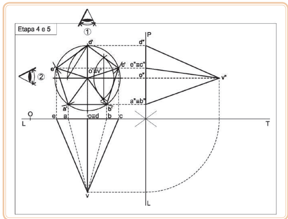
Figura 6.9: Traçado da projeção da pirâmide no PL
