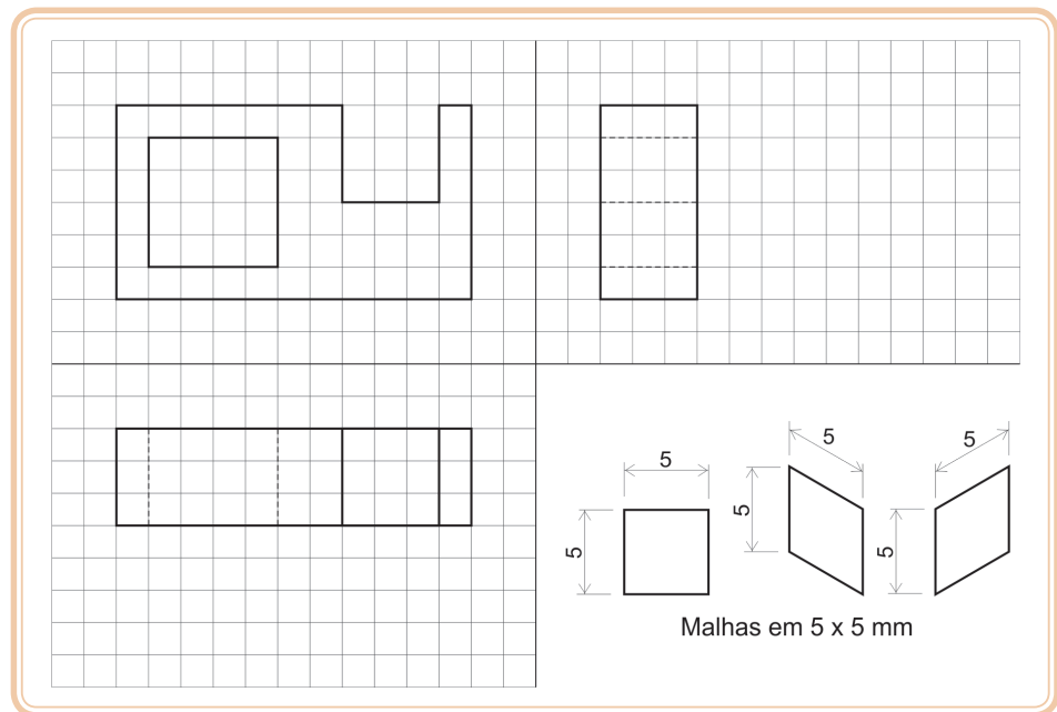
Figura 7.4: Vistas ortográficas da Figura 7.3
