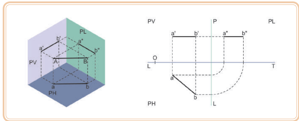
Figura 4.13: Reta de nível
