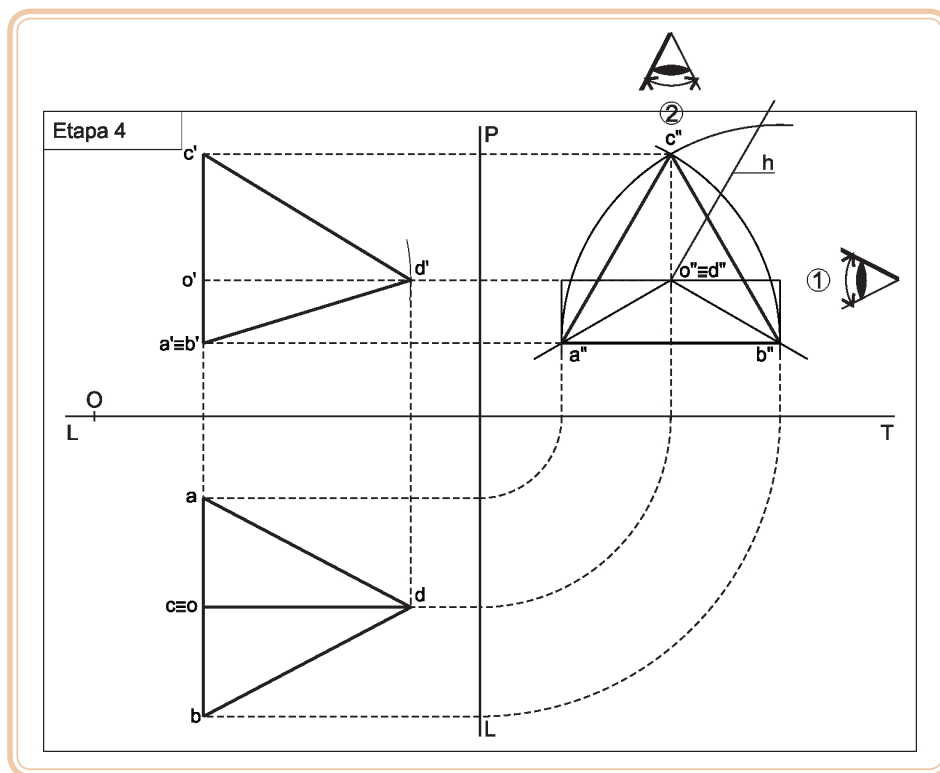
Figura 6.13: Projeções no PV e no PH
