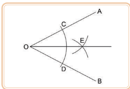
Figura 2.39: Traçado da bissetriz
