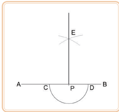
Figura 2.27: Traçado da perpendicular
