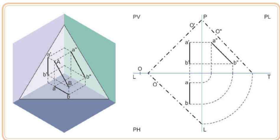
Figura 5.34: Plano obluo – reta de perfil
