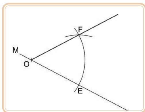
Figura 2.55: Traçado de linha do ângulo transportado
