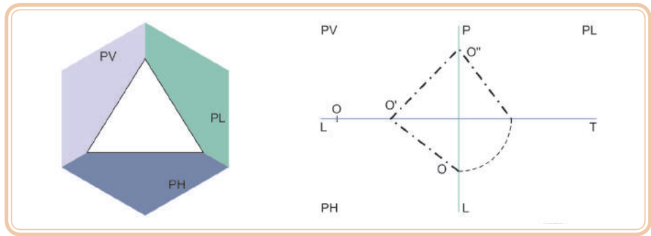
Figura 5.8: Plano oblíquo
