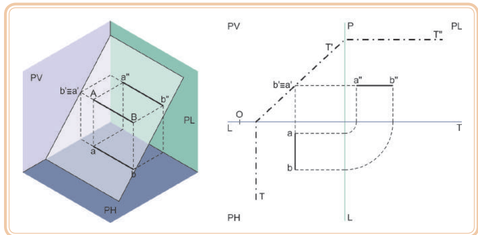
Figura 5.10: Plano de topo – reta de topo
