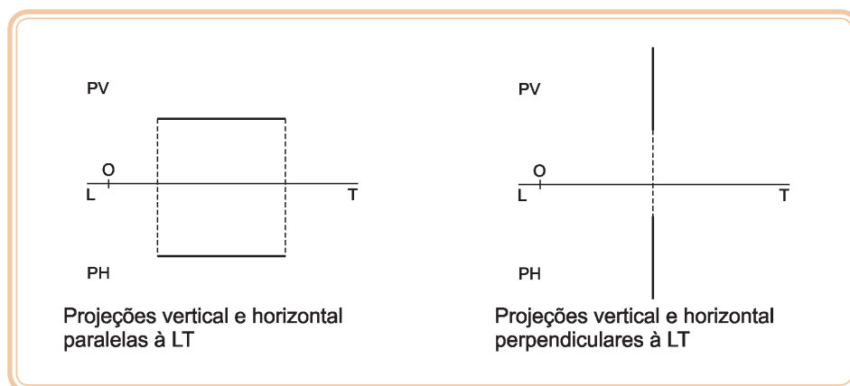
Figura 4.7: Projeção de um segmento de reta em relação à LT
