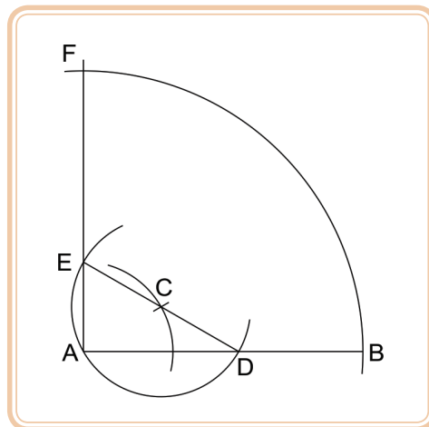
Figura 3.14: Arco para determinar o ponto F
