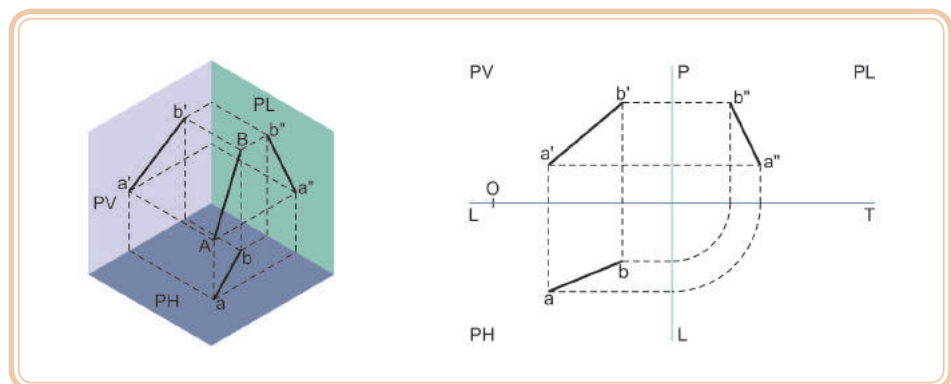
Figura 4.15: Reta oblíqua
