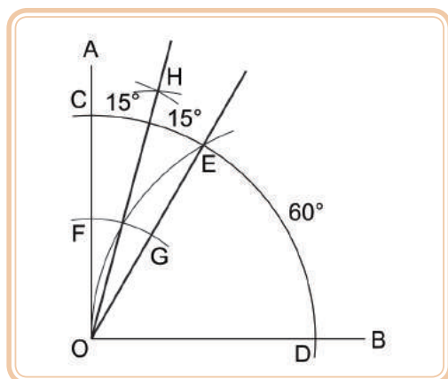
Figura 2.51: Traçado da bissetriz que define o ângulo de 15^\circ
