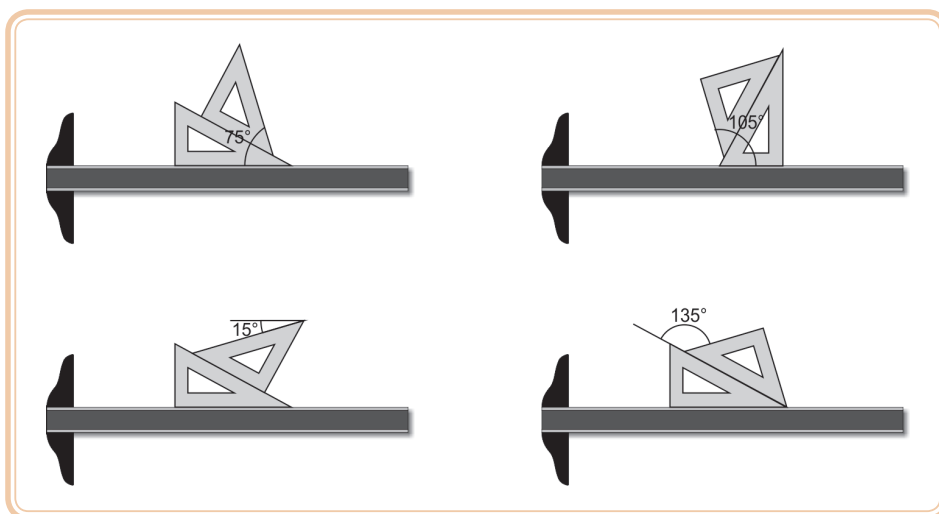
Figura 1.8: Ângulos obtidos com os esquadros
