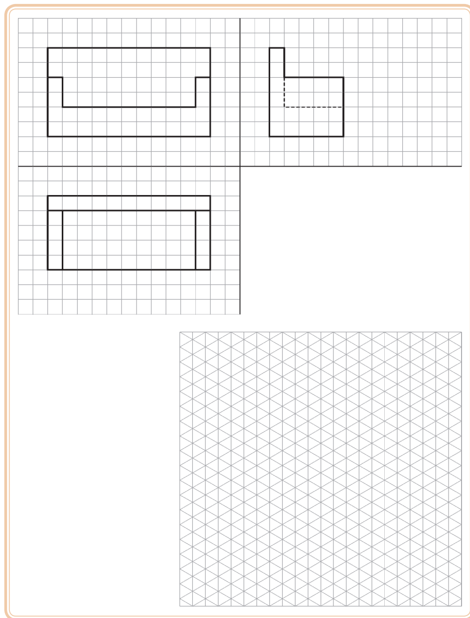
Exercício 1.1: Execução da perspectiva isométrica
