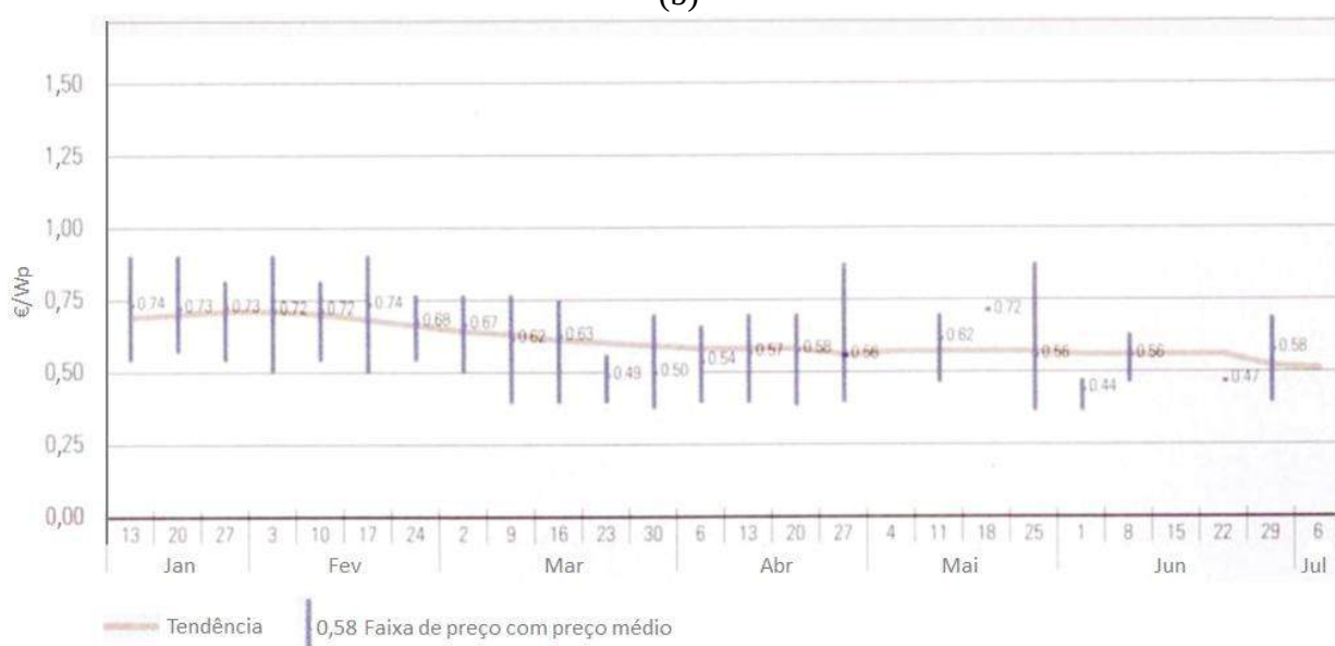
Figura A2.6 - Preços praticados no mercado alemão, de 13/01 a 06/07/2012, para módulos FV de silício, (a) monocristalino (m-Si), (b) policristalino (p-Si) e (c) amorfo (a-Si). Fonte: [PHOTON 2012].
