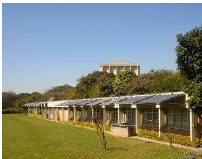
Figura A3.13 - Sistema fotovoltaico de 12 kW instalado na fachada do prédio da administração do IEE. Fonte: LSF.
