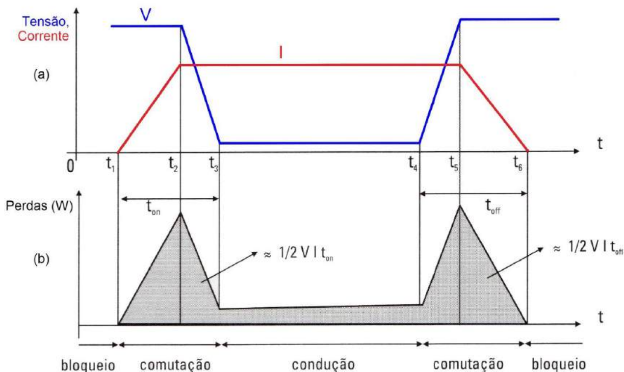
Figura 4.30—(a) Formas de onda de tensão (V) e corrente (I) sobre um dispositivo semiconductor em chaveamento e condução, e (b) potência dissipada em um dispositivo semiconductor em chaveamento e condução (adaptado de PROCEL, 2004).
