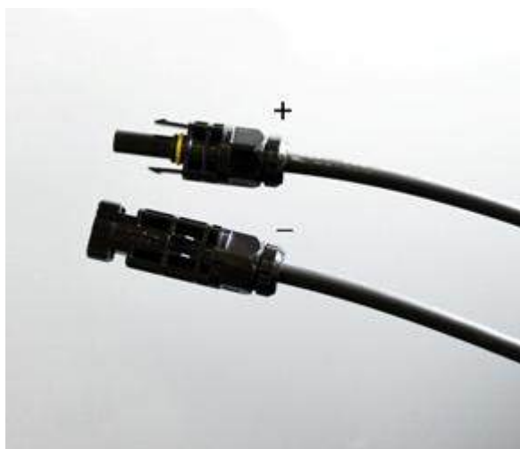
Figura 4.7 – Conectores de engate rápido MC4 para conexão série de módulos fotovoltaicos.
