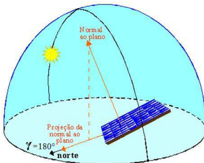
Figura 7.6 – Orientação da face dos módulos fotovoltaicos para o norte verdadeiro em um dado local no hemisfério Sul (ângulo azimutal de superfície igual a 180^\circ ).
