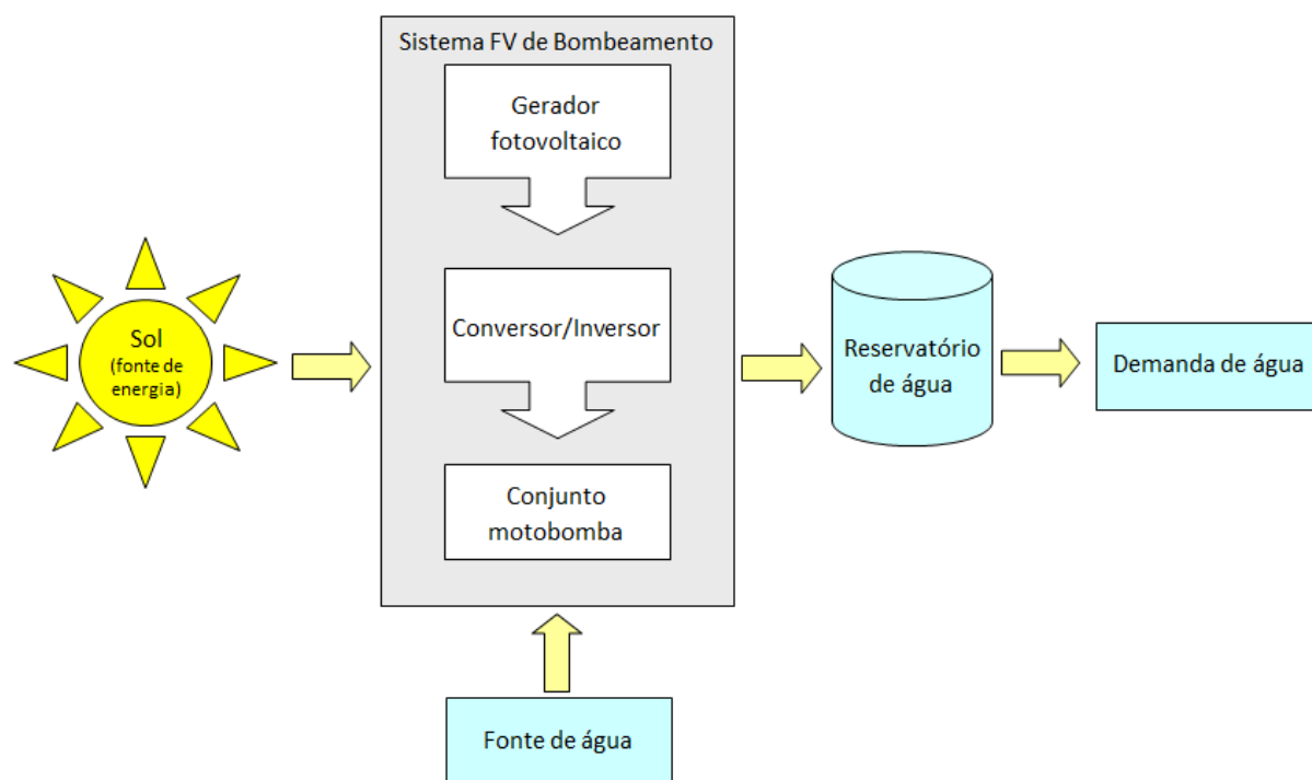
Figura 5.11 – Diagrama esquemático de um sistema fotovoltaico de abastecimento de água. Fonte: Modificado de (FRAINDEIRAICH, 2002).
