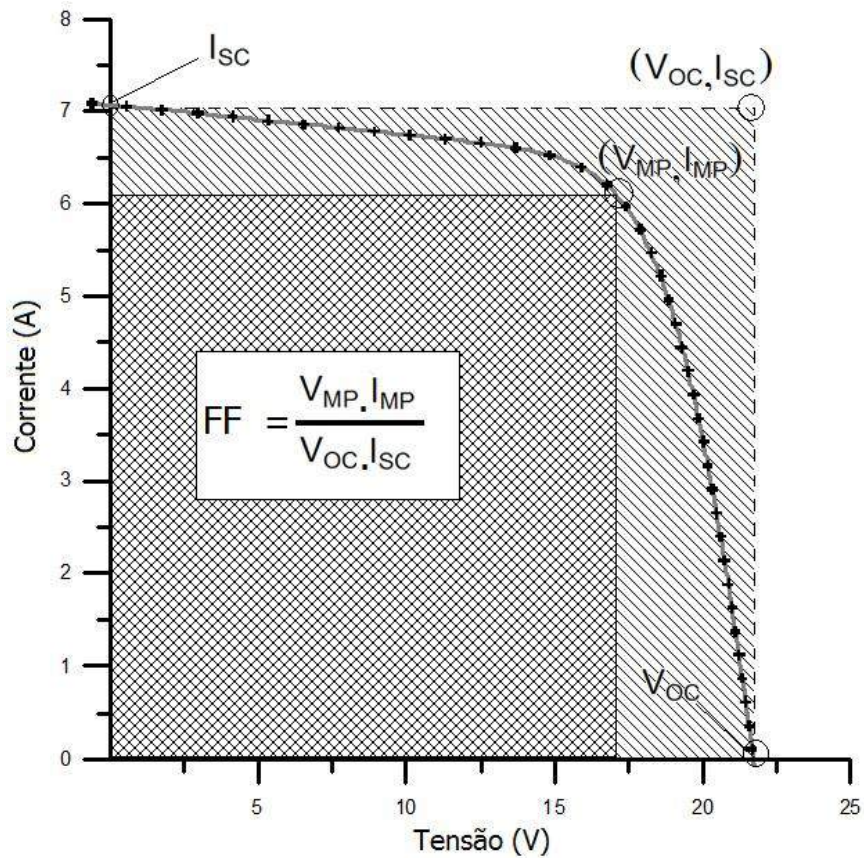
Figura 4.2 – Definição do fator de forma.
