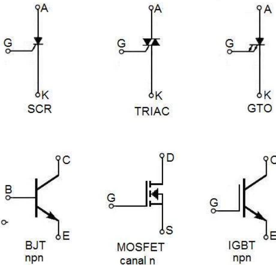
Figura 4.29– Símbolos de componentes utilizados em inversores (A – anodo; K – catodo; G – gate; B- base, C – coletor; E – emissor; D – dreno; S – fonte).
