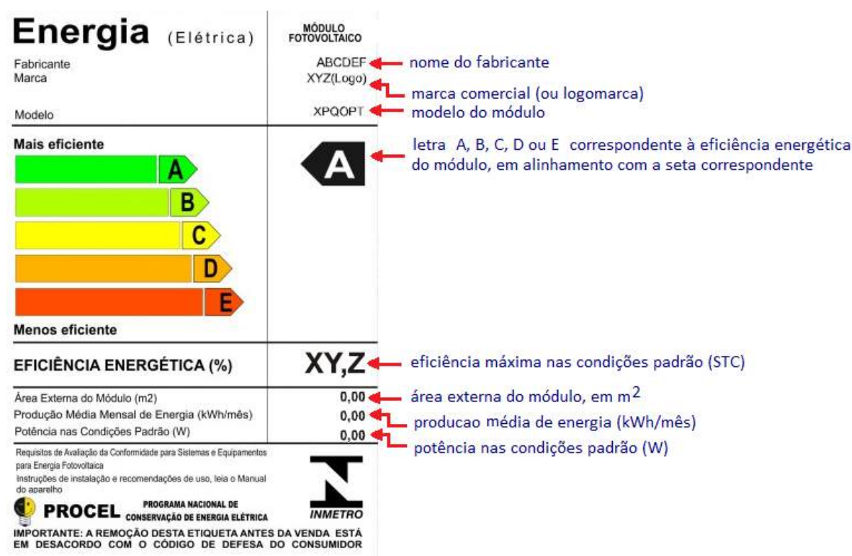
Figura 4.5 – Modelo de etiqueta do Inmetro afixada nos módulos; os dados indicados pelas setas são informados para cada modelo de módulo, depois dos ensaios realizados por laboratório credenciado. Adaptado de (INMETRO, 2011).
