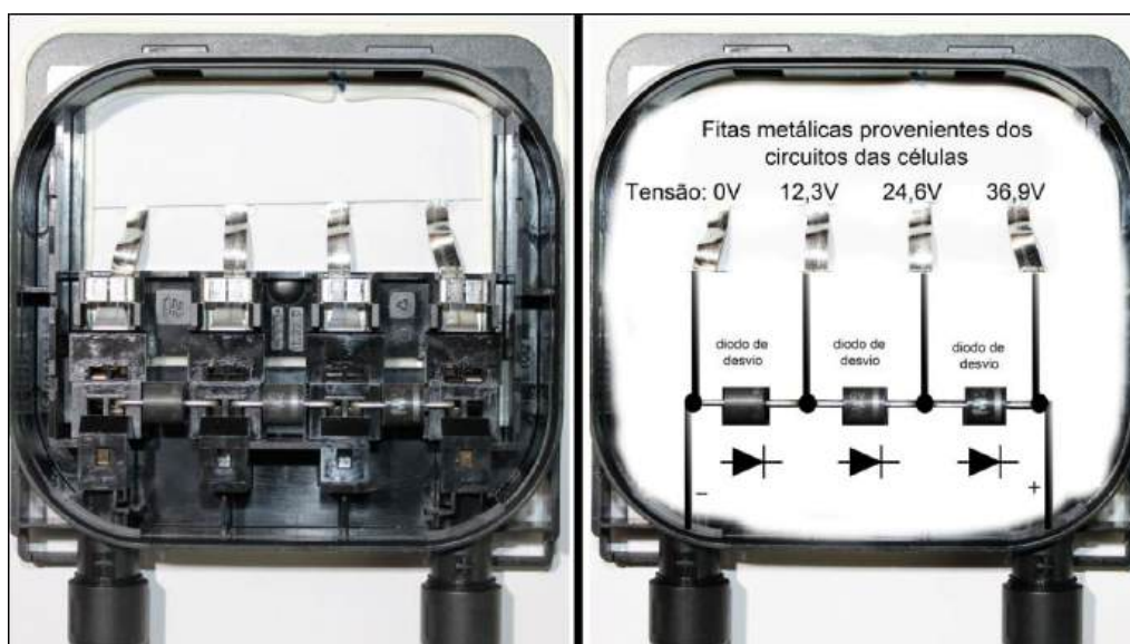
Figura 4.6 – Caixa de conexões (esquerda) e diagrama de ligações (direita) de um módulo de 240 Wp, com 60 células em série (20 para cada diodo), onde V_{OC} = 36,9 \text{ V} .
