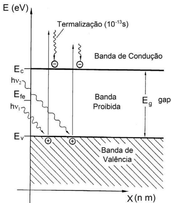
Figura 3.3 – Geração de pares elétron-lacuna pela incidência de fótons no material semicondutor, chamado efeito fotocondutivo: E_c – nível inferior de energia da banda de condução; E_v – nível máximo de energia na banda de valência; E_{fe} – Nível de Fermi; E_g – valor da energia do gap ( E_g = E_c - E_v ). Fonte: adaptado de (OLDENBURG, 1994).
