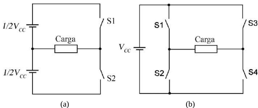
Figura 4.33 – Inversor de (a) meia ponte e (b) ponte completa monofásica.
