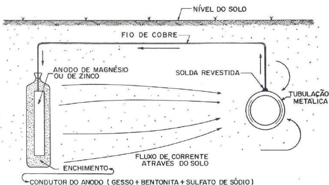
Figura 5.18 – Proteção catódica com anodo galvânico.
