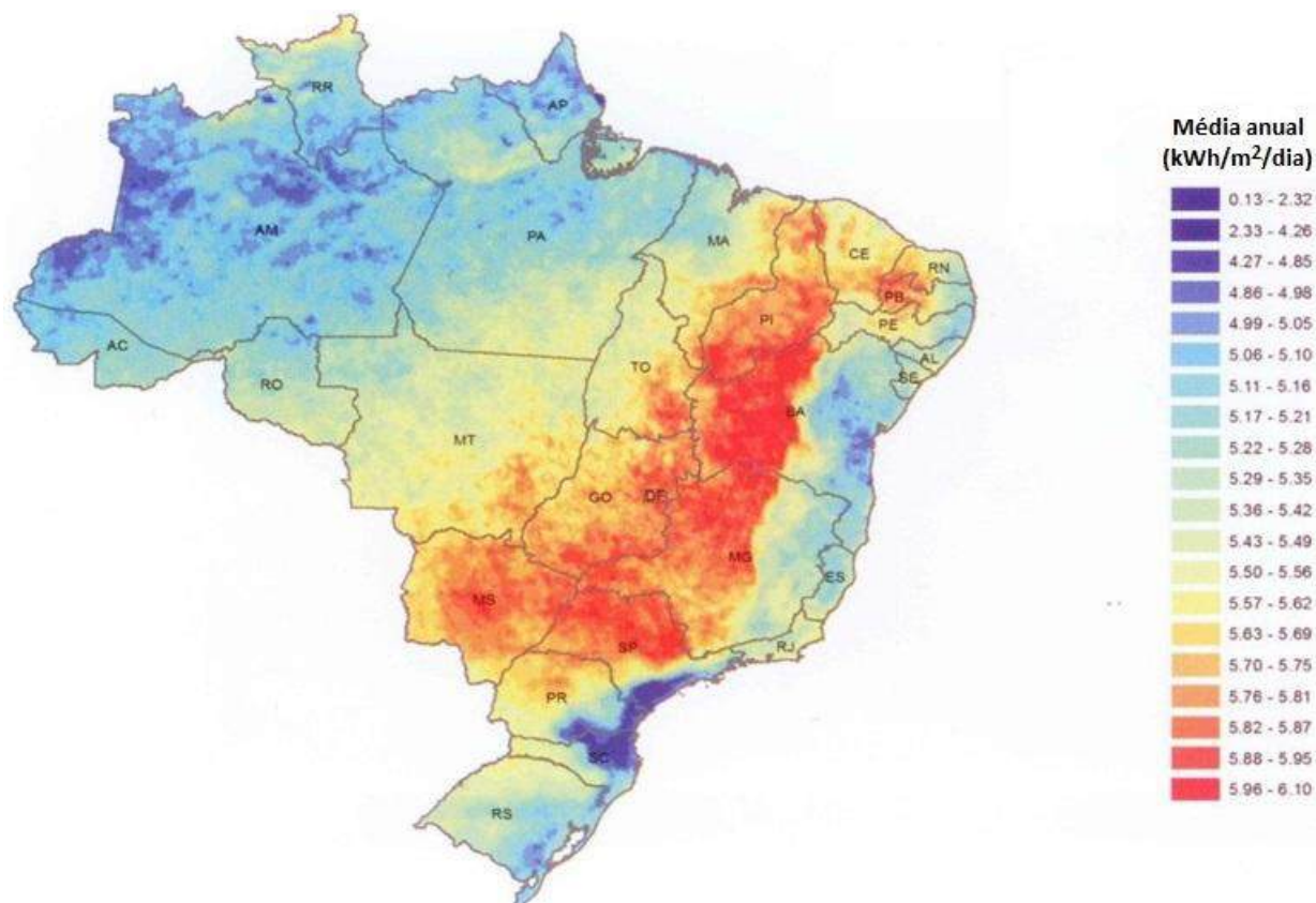
Figura A2.11 - Irradiação solar incidente sobre superfície com inclinação igual à latitude do local e voltada para o equador.
