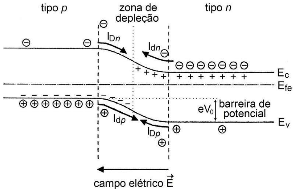
Figura 3.5 – Junção pn no escuro em equilíbrio térmico, mostrando a barreira de potencial ( qV_o ) as correntes de difusão ( I_d ) e de deriva ( i_D ) de portadores: i_{dn} – corrente de difusão de elétrons; i_{dp} – corrente de difusão de lacunas; i_{Dn} – corrente de deriva de elétrons; I_{Dp} – corrente de deriva de lacunas. Fonte: adaptado de (OLDENBURG, 1994).
