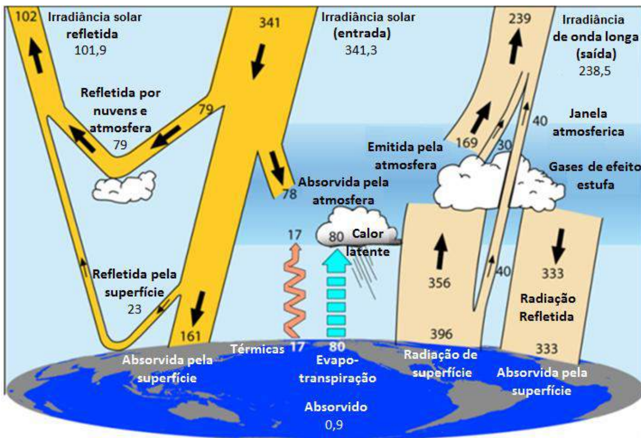
Figura 2.7 - Fluxo de potência global (em \text{W/m}^2 ). O valor da irradiância solar incidente no topo da atmosfera aqui apresentado é um fluxo médio anual recebido ao longo das 24 horas de um dia ( 341,3 \text{ W/m}^2 ) no topo da atmosfera. Fonte: (Trenberth et al. , 2009).
