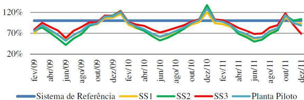
Figura 6.17 - Comparação da produtividade entre a Planta Piloto (subsistemas 1, 2 e 3) e o Sistema de Referência. Fonte: (ZOMER et al., 2012).
