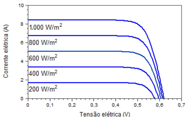
Figura 3.17 - Influência da variação da irradiância solar na curva característica I - V de uma célula fotovoltaica de silício cristalino na temperatura de 25 °C.
