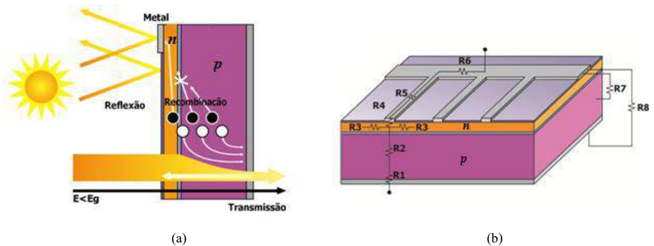
Figura 3.8. Fatores que limitam a eficiência de uma célula fotovoltaica: a) Perdas por reflexão, transmissão (fótons com energia menor que o gap ), recombinação de portadores de carga minoritários e sombreamento proporcionado pela malha metálica frontal. b) Perdas por resistência em série nas junções metal-semicondutor (R4 e R1) existentes nos contatos metálicos frontal e traseiro, perdas nas trilhas metálicas (R5 e R6) e nas regiões n (R3) e p (R2) e perdas por resistência em paralelo entre o contato metálico frontal (malha metálica) e a região tipo p (R7), e entre os contatos metálicos frontal e traseiro (R8). Adaptada de (MOEHLECKE e ZANESCO, 2005).
