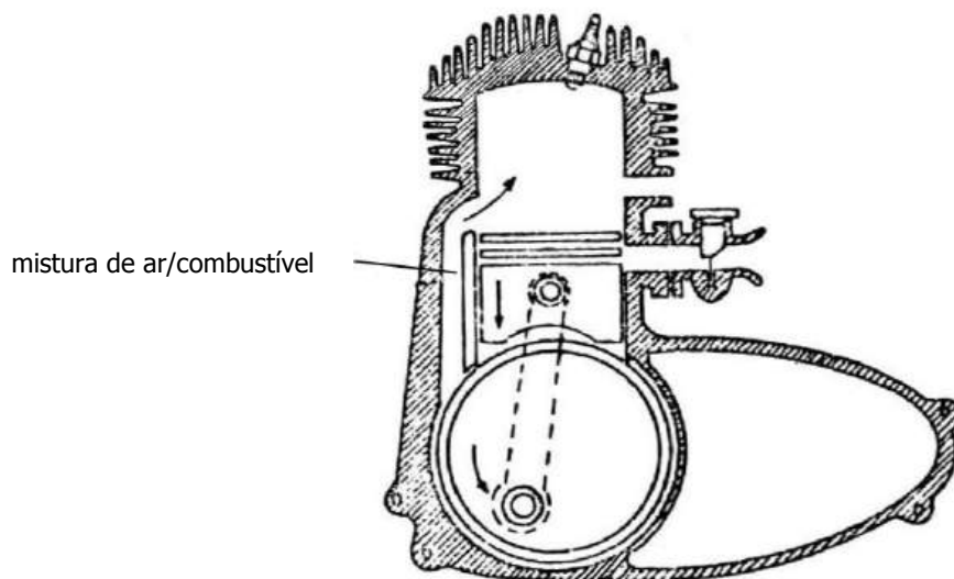
Fig. 9 – Admissão-transmissão do cárter para o cilindro
