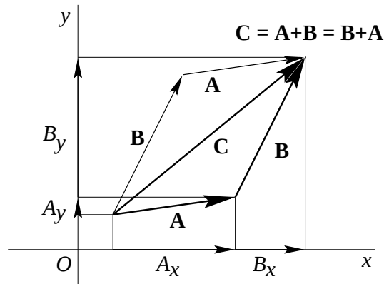
Figura 1.4: Adição de dois vetores.
