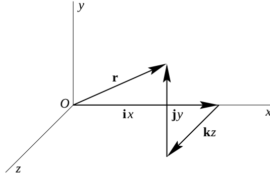
Figura 1.11: O vetor posição.
