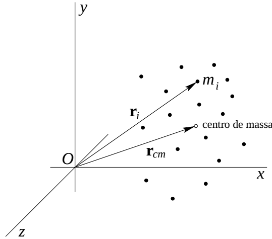
Figura 4.1: Centro de massa de um sistema de partículas.
