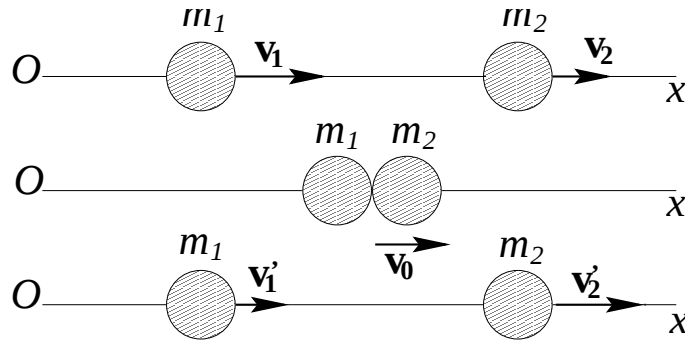
Figura 4.5: Colisão frontal de duas partículas.
