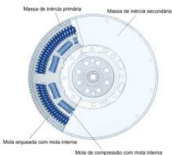
Figura 65 – Volante bi-massa
