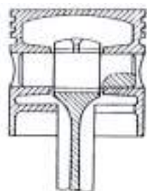
Figura 49 – Pino semiflutuante
