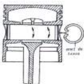
Figura 48 – Pino flutuante
