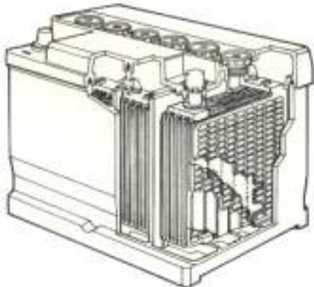
Figura 158 - Bateria
