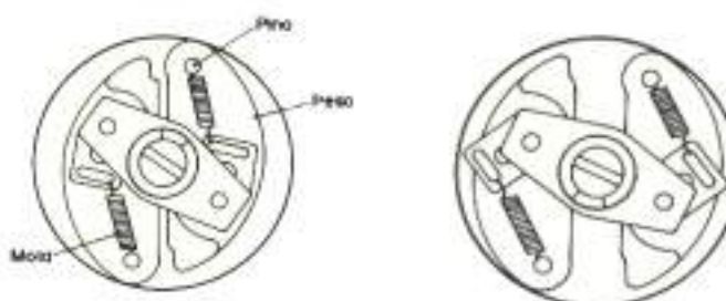
Figura 167 - Funcionamento
