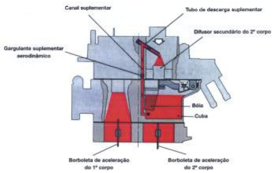
Figura 134 -Sistema suplementar e seus componentes
