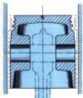
Figura 46 - Dilatação do êmbolo
