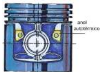
Figura 47– Anel autotérmico
