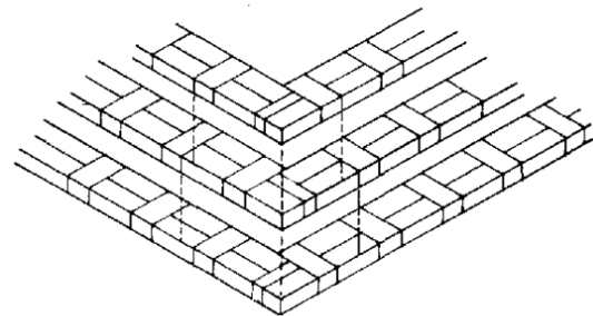
(d) Flemish bond
