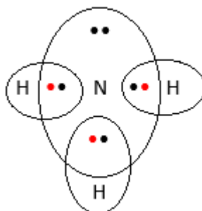
Amoníaco (NH 3 )
