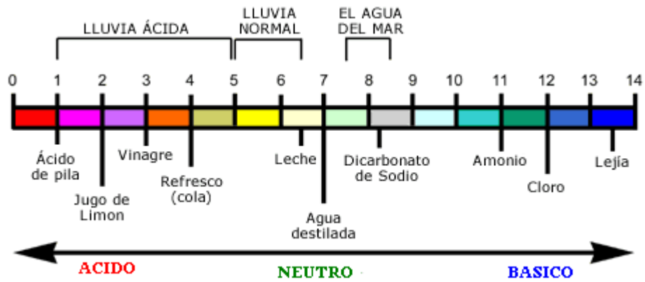
Figura 3.4. Escala de pH.
