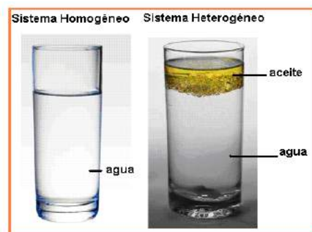
Figura 1. 4. Sistemas materiales
