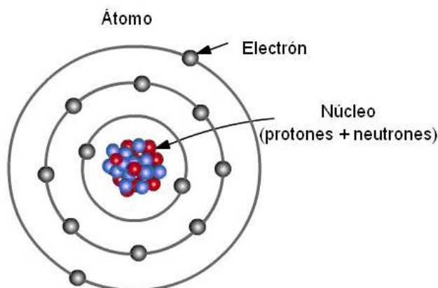
Figura 2. 1. Estructura del átomo
