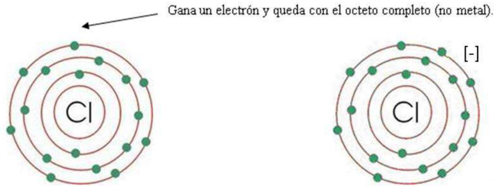
Figura 3.3. El átomo de cloro que se transforma en ion cloruro \text{Cl}^- (anión)
