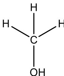
Figura 5.2. Metanol ( \text{CH}_3\text{OH} )
