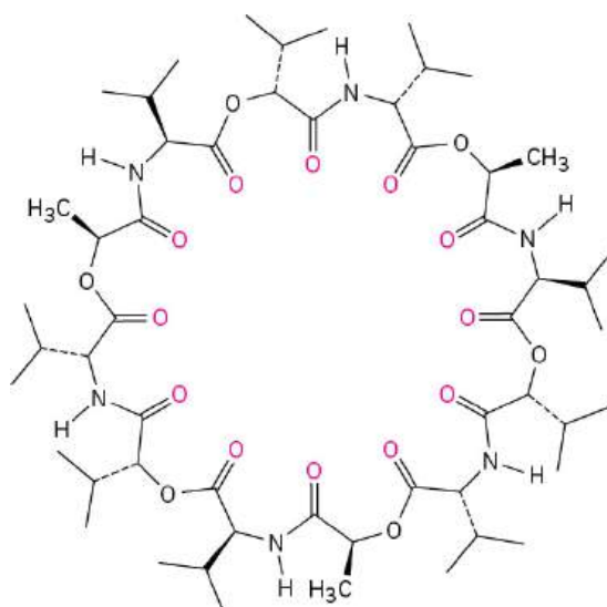
Valinomycin
