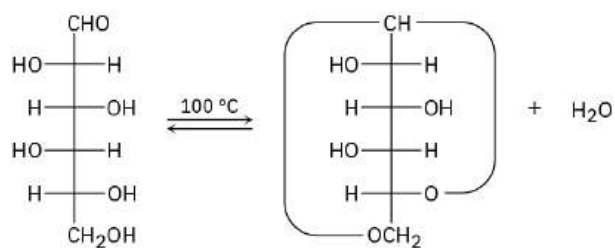
D-Idose
