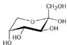
\alpha -D-Fructopyranose
