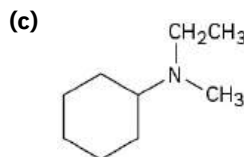
Pyrrolidine
