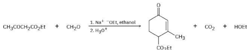
Hagemann's ester
