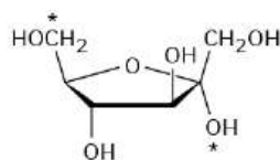
\alpha -D-Fructofuranose
