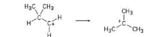
Isobutyl cation
