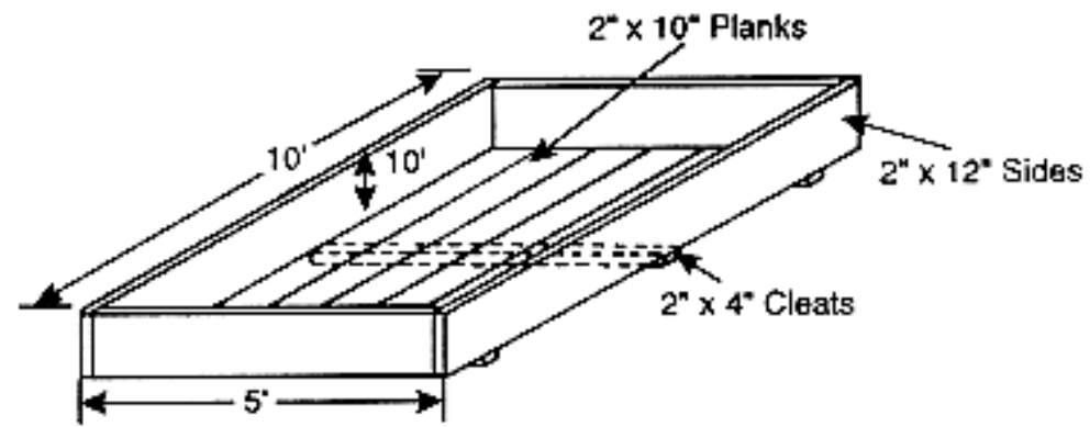
Mortar box
