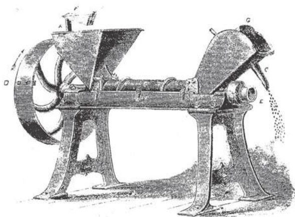
Pulidora "Squier"
