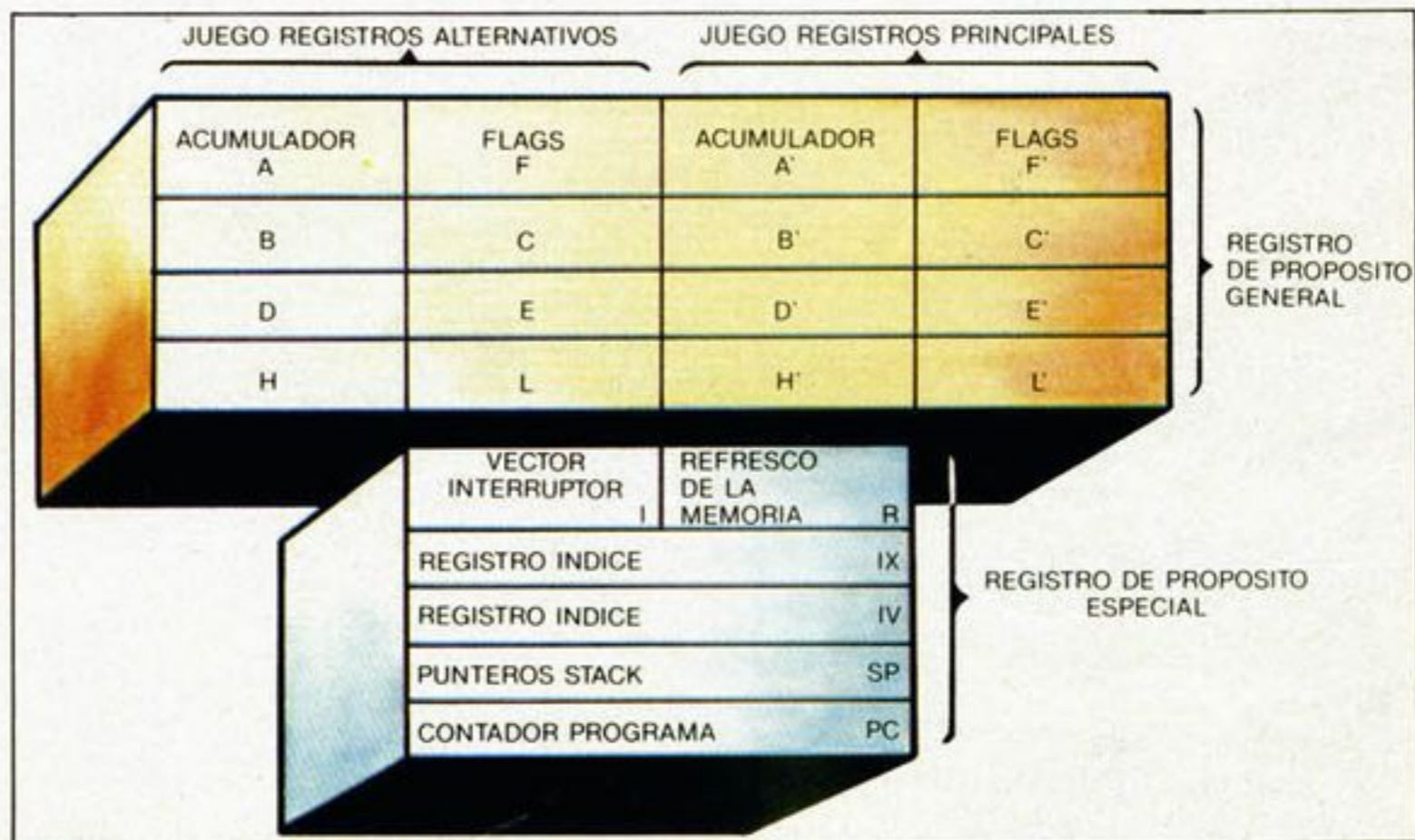
Figura 1: Registros de programación del Z-80.
