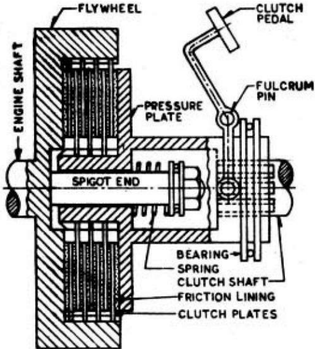
Fig : Multi-Plate Clutch
