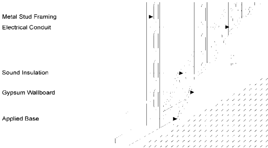
Fig. 1 Stud partition
