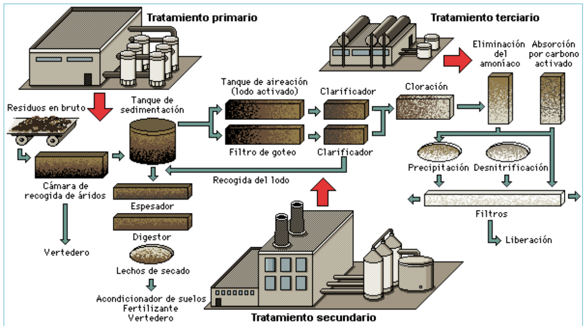
Fig.27 Fases de tratamiento de aguas residuales
