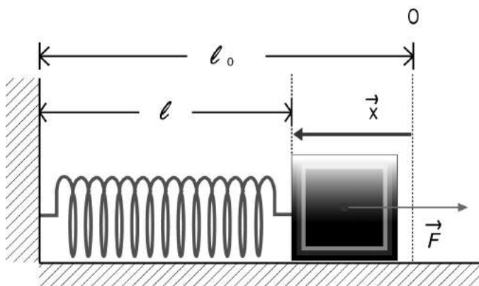
Figura 25: Mola comprimida
