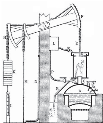
Figura 9: Máquina de Newcomen
