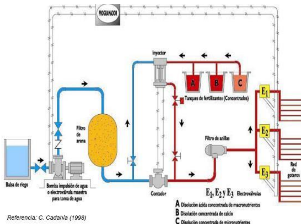
Figura 11. Sistema para fertirriego
