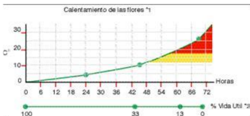
Figura 169. Temperatura con termoregistradores (varias replicaciones) al interior de 10 cajas elegidas al azar, incluidas en un ballet de avión y mantenidas en un cuarto frío a 2 °C. 2. expectativa de vida útil, según la temperatura de embarque en Bogotá.
