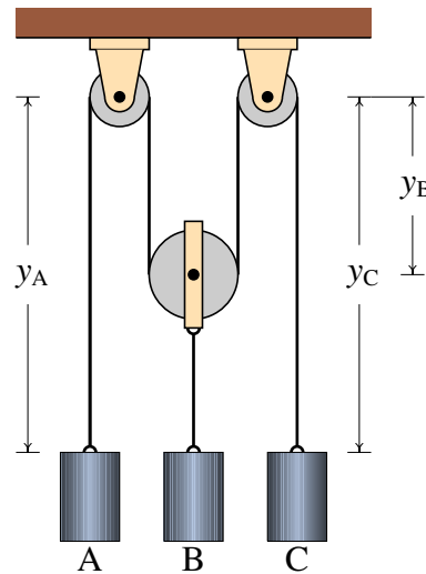
Figura 2.12.: Sistema com movimentos dependentes e dois graus de liberdade.
