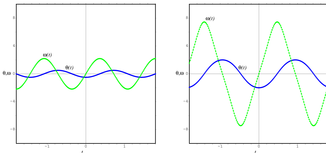
Figura 9.6.: Oscilações do pêndulo, com amplitude angular de 29^\circ (esquerda) e 115^\circ (direita).
