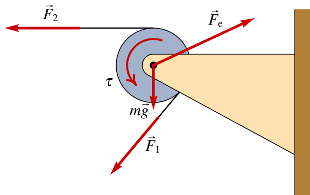
Figura 6.9.: Forças e torques externos sobre uma roldana.
