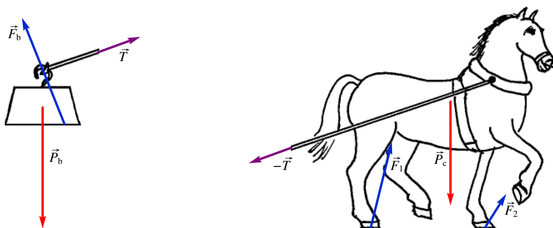
Figura 4.2.: Forças sobre o bloco e sobre o cavalo.
