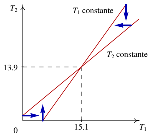
Figura 8.1.: Nulclinas e temperaturas de equilíbrio no exemplo 8.2.
