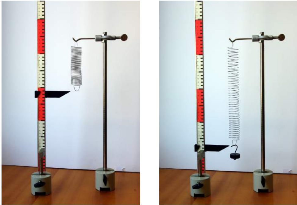
Figura 5.3.: Mola elástica pendurada dum suporte horizontal. A elongação é diretamente proporcional ao peso colocado.
