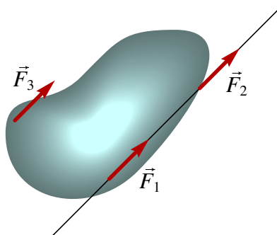
Figura 6.1.: Três forças com o mesmo módulo, direção e sentido. \vec{F}_1 e \vec{F}_2 são equivalentes, mas são diferentes de \vec{F}_3 .
