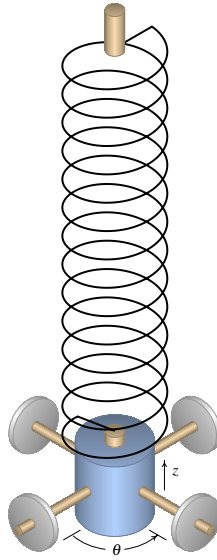
Figura 10.5.: Pêndulo de Wilberforce.
