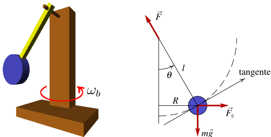
Figura 12.3.: Pêndulo simples com a base em rotação no plano horizontal e diagrama de forças externas.
