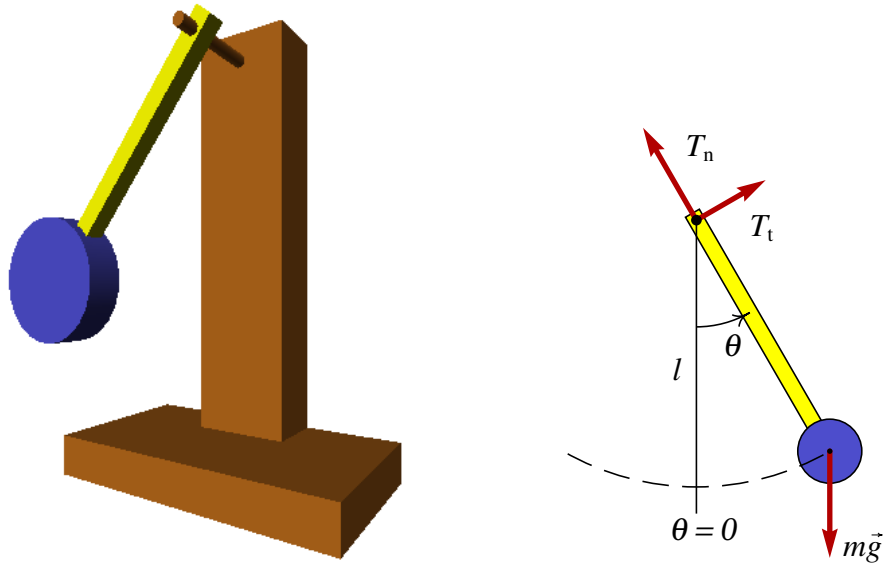
Figura 9.3.: Pêndulo formado por um disco e uma barra que pode rodar à volta de um eixo horizontal.
