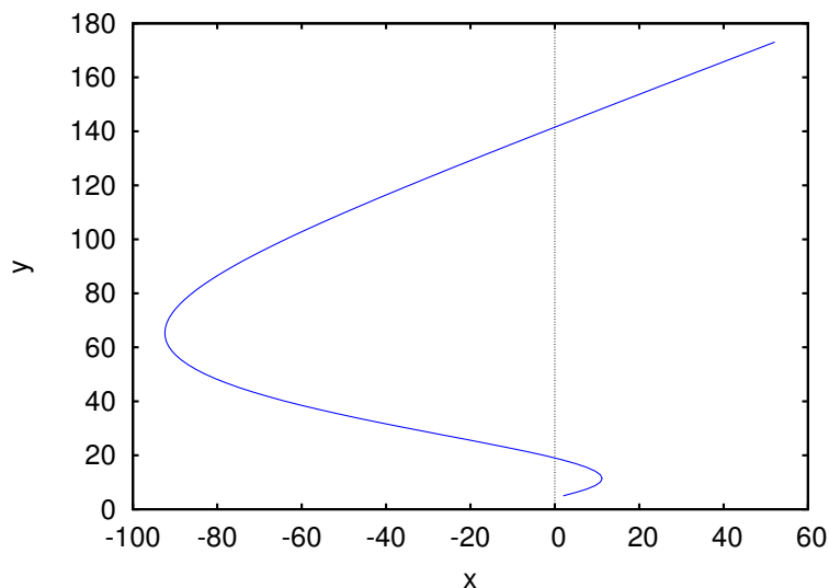
Figura 2.6.: Trajetória da partícula durante os primeiros 60 segundos, desde o instante em que a partícula se encontrava no ponto (5, 2).
