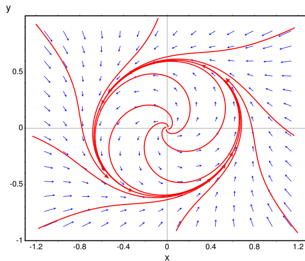
Figura 11.5.: Retrato de fase do sistema \dot{x} = -y + x(1 - 2x^2 - 3y^2) , \dot{y} = x + y(1 - 2x^2 - 3y^2) .
