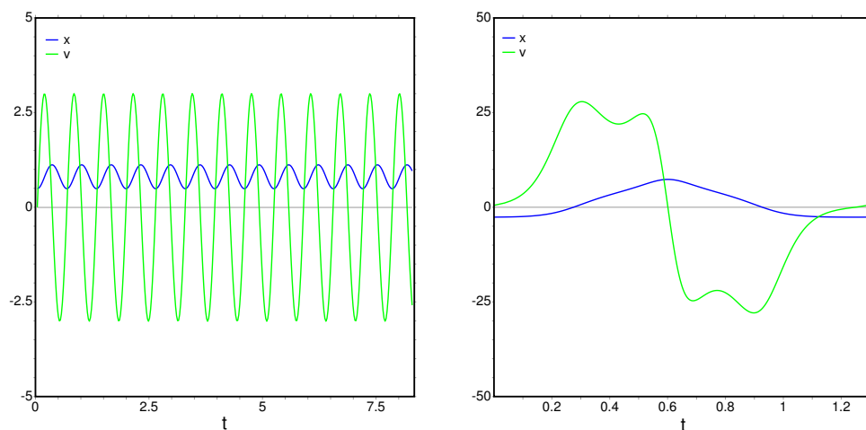
Figura 7.8.: Posição e velocidade em função do tempo no caso de um ciclo (esquerda) e de uma órbita homoclínica.
