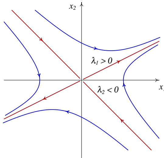
Figura 8.5.: Ponto de sela: existem duas direções em que o estado evolui em linha reta, num dos casos afastando-se da origem e no outro caso aproximando-se.
