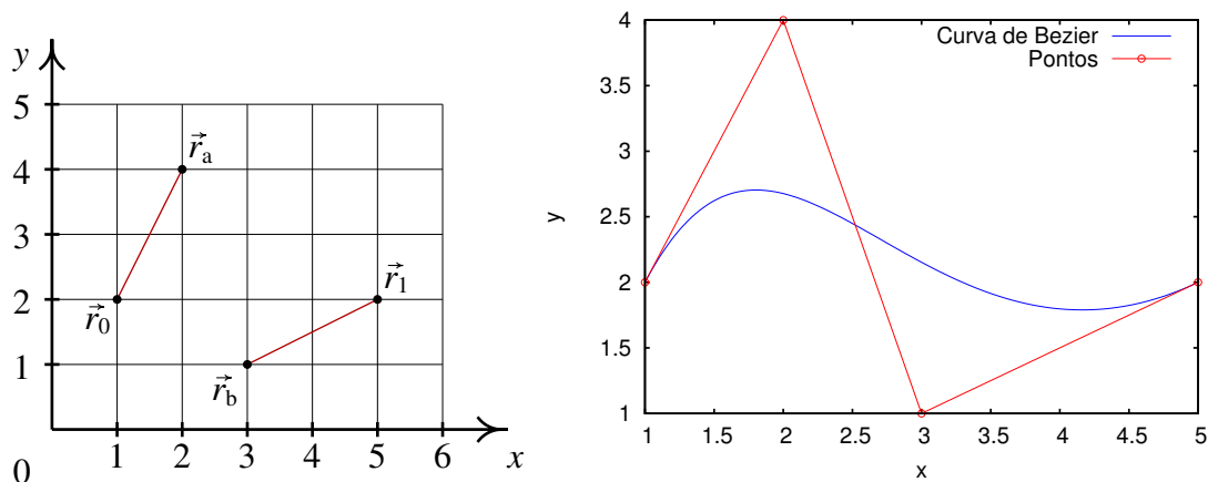
Figura 3.8.: Os quatro pontos de controlo que definem uma curva de Bézier e a curva obtida com esses pontos.
