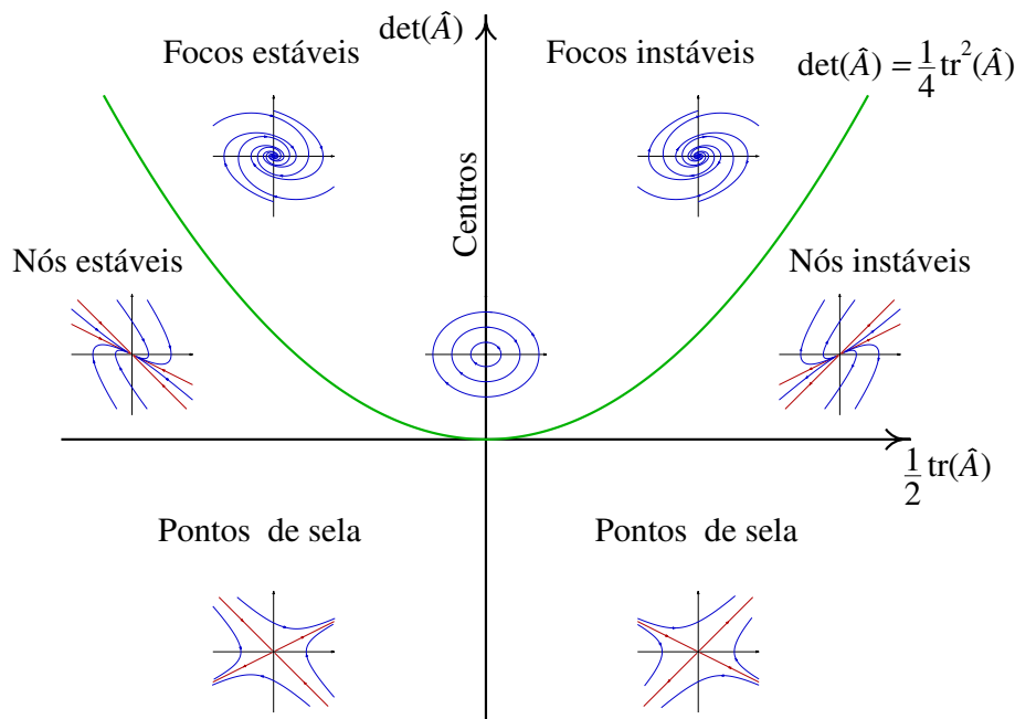
Figura 8.8.: Tipos de ponto de equilíbrio de um sistema linear com duas variáveis de estado.
