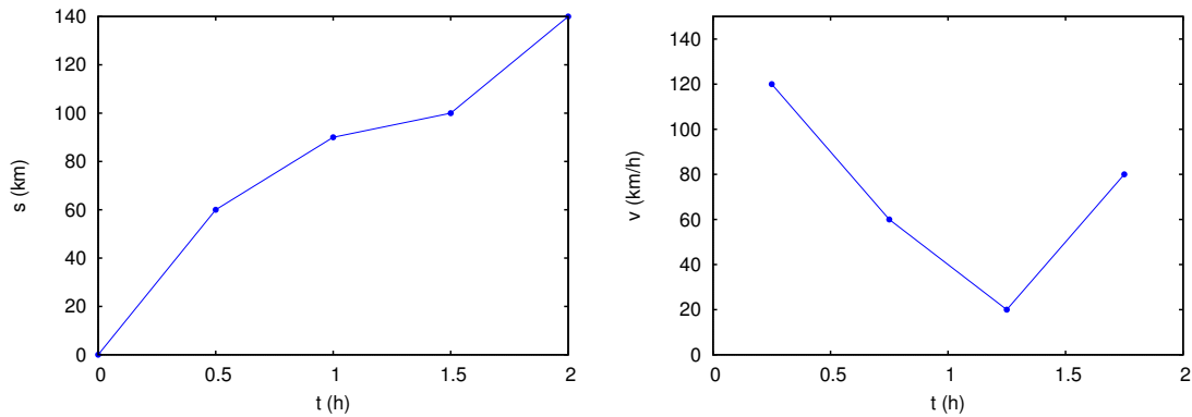
Figura 1.4.: Gráficos da posição, s , e da velocidade média, \bar{v} , em função do tempo, t .
