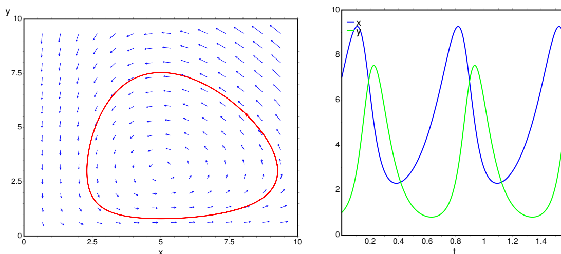
Figura 11.7.: Retrato de fase do modelo de Lotka-Volterra e gráfico das populações em função do tempo.
