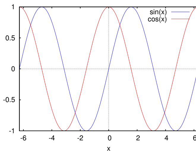
Figura A.3.: Gráfico das funções seno e co-seno.
