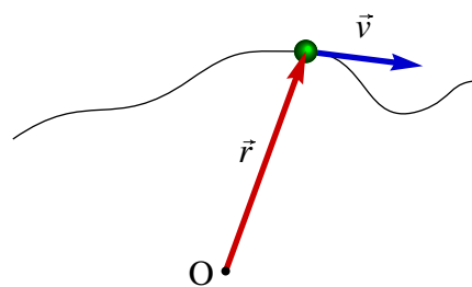
Figura 7.1.: O estado de uma partícula em qualquer instante é dado pelos vetores de posição e velocidade.
