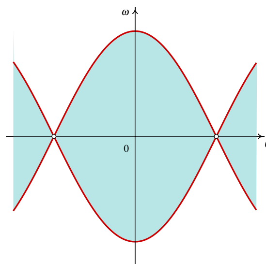
Figura 9.5.: As órbitas heteroclínicas delimitam a região de movimento oscilatório.
