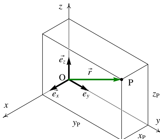
Figura 2.4.: Coordenadas cartesianas ( x_P , y_P , z_P ) de um ponto P, em relação a um referencial definido por 3 versores perpendiculares, \vec{e}_x , \vec{e}_y e \vec{e}_z .
