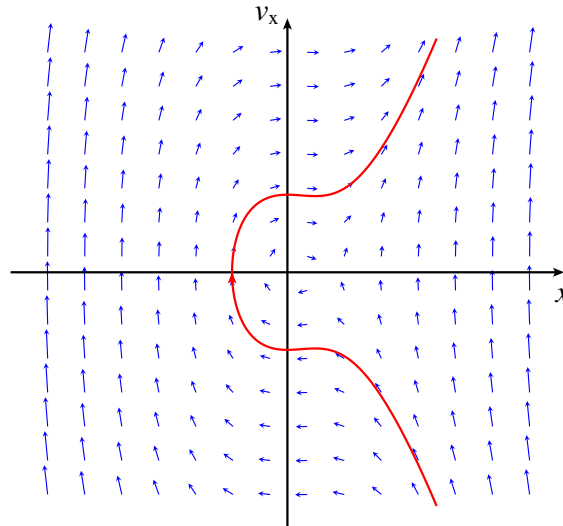
Figura 7.3.: Velocidade de fase em vários pontos do espaço de fase e uma curva de evolução do sistema.
