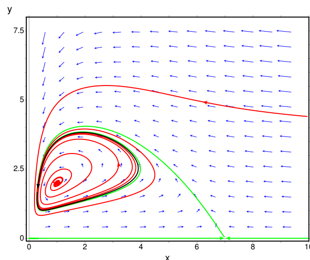
Figura 11.8.: Retrato de fase do modelo de Holling-Tanner.
