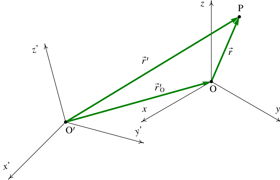
Figura 2.7.: Relação entre os vetores posição de um ponto em dois referenciais diferentes.
