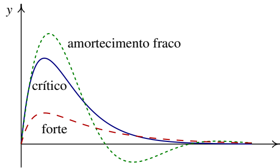
Figura 8.13.: Variação da altura y em função do tempo, para os três tipos de amortecimento.
