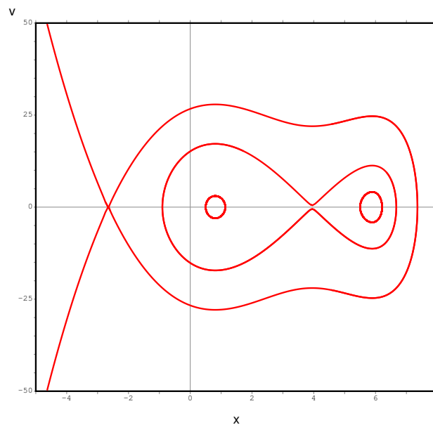
Figura 7.9.: Curvas de evolução do exemplo 7.2, obtidas a partir das curvas com energia constante.
