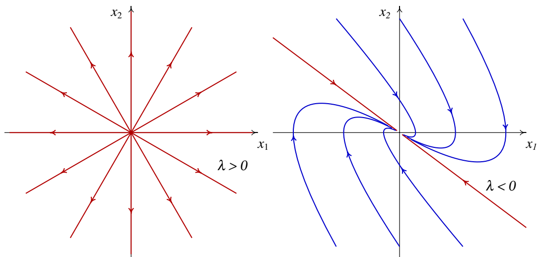
Figura 8.9.: Retratos de fase de um nó próprio instável (esquerda) e de um nó impróprio estável (direita).
