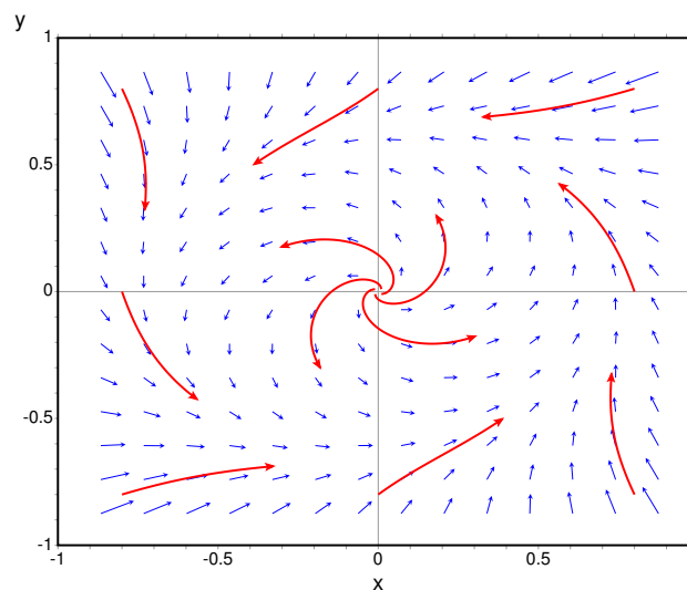
Figura 11.4.: Retrato de fase de um sistema com um ciclo limite.
