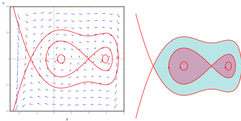
Figura 7.6.: Retrato de fase do exemplo 7.2. No lado direito, as regiões onde o sistema oscila (regressa ao seu estado inicial) foram coloridas.
