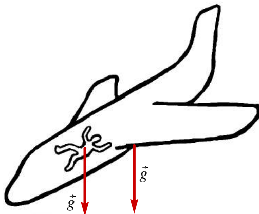
Figura 2.8.: A aceleração de um corpo em queda livre, em relação a um referencial que também está em queda livre, é nula.
