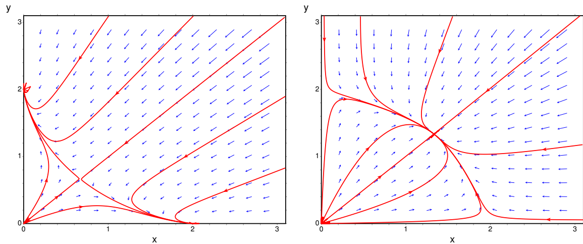
Figura 11.9.: Retratos de fase do exemplo 11.5, nos casos em que c_1 , c_2 e c_3 são todas negativas (esquerda) ou positivas (direita). No primeiro caso o ponto de equilíbrio é instável, e no segundo caso é estável.
