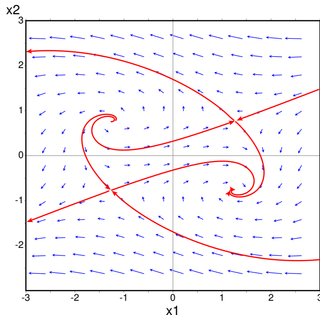
Figura 9.2.: Retrato de fase do sistema \dot{x}_1 = 4 - x_1^2 - 4x_2^2 , \dot{x}_2 = x_2^2 - x_1^2 + 1 .
