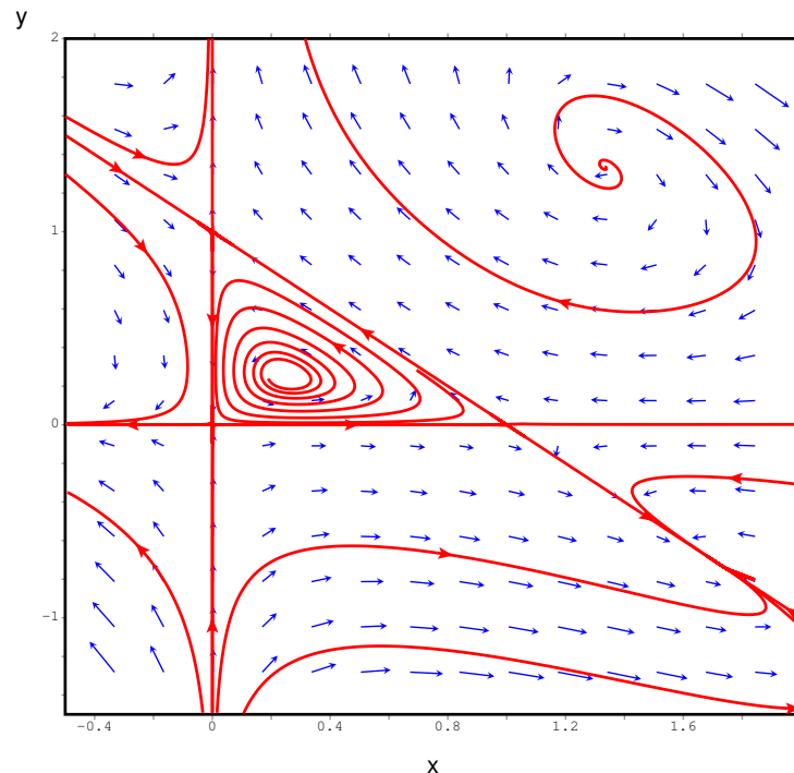
Figura 12.1.: Retrato de fase do exemplo 12.1, com uma órbita heteroclínica atrativa..
