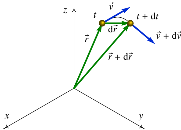
Figura 5.1.: Vetores posição e velocidade num instante t e num instante posterior t + dt .
