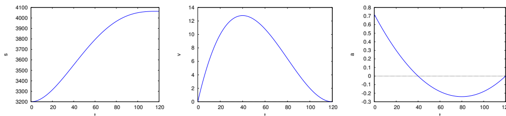
Figura 1.5.: Gráficos da distância percorrida, velocidade e aceleração tangencial do barco no exemplo 1.2.
