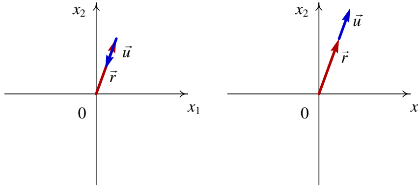
Figura 8.2.: Quando a velocidade de fase é paralela ao vetor de estado, o sistema aproxima-se ou afasta-se do ponto de equilíbrio na origem.
