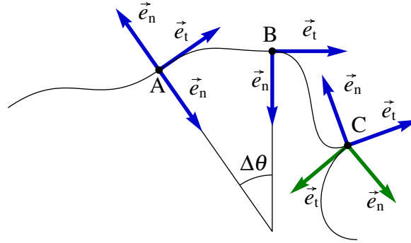
Figura 3.4.: Versores tangencial, \vec{e}_t , e normal, \vec{e}_n em diferentes pontos da trajetória.
