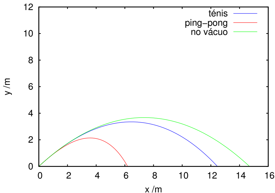
Figura 5.5.: Trajet  rias de uma bola de t  nis, uma bola de t  nis de mesa e uma bola hipot  tica no v  cuo.
