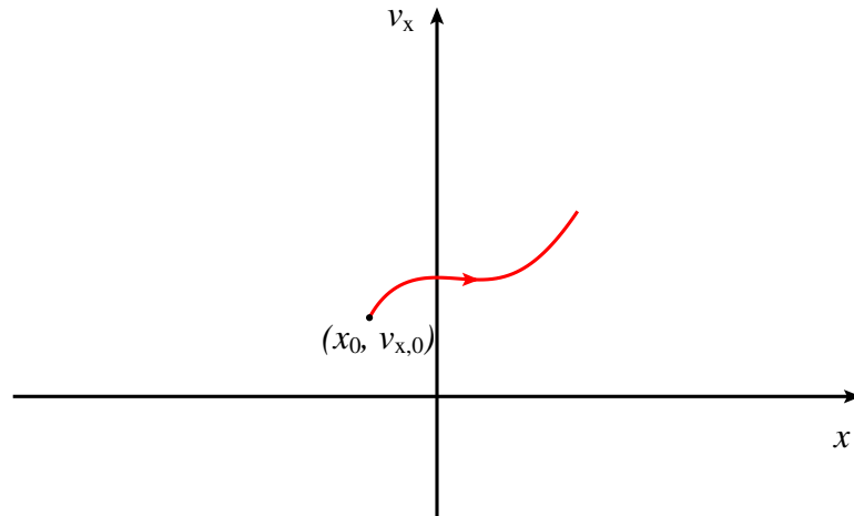
Figura 7.2.: Espaço de fase de uma partícula que se desloca ao longo do eixo dos x .
