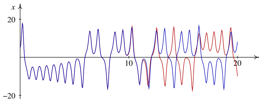
Figura 12.7.: Oscilações do sistema de Lorenz para dois valores muito próximos do valor inicial: x(0) = 5 (vermelho) e x(0) = 5.005 (azul). Parâmetros: \sigma = 10 , b = 8/3 , r = 28 , y(0) = 5 , z(0) = 5 .
