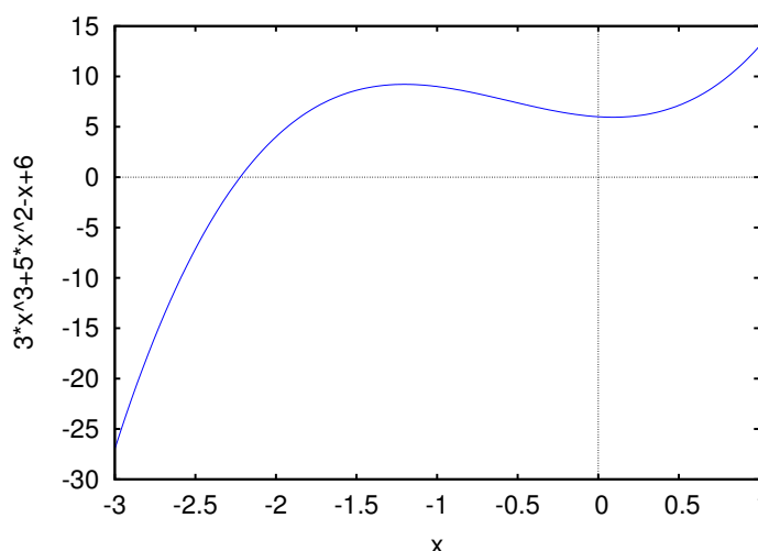
Figura A.2.: Gráfico do polinómio 3x^3 + 5x^2 - x + 6 .
