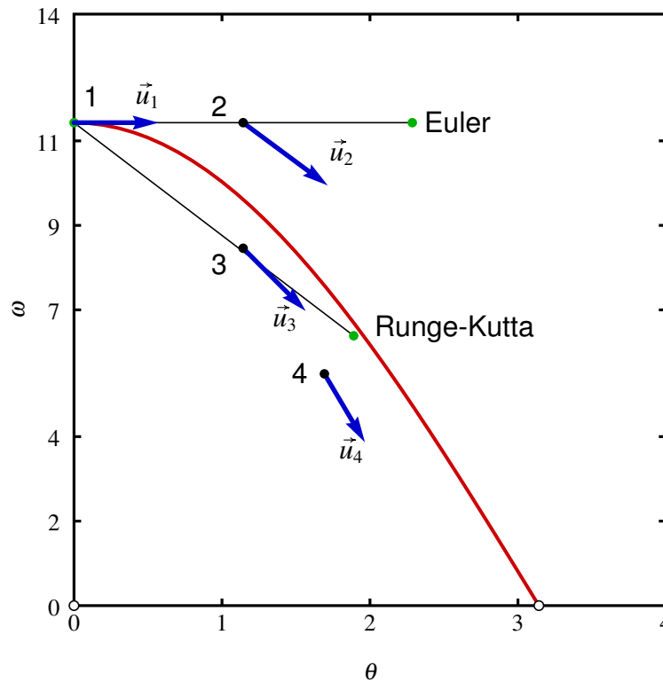
Figura 10.1.: Separatriz do pêndulo com l = 30 cm, mostrando as aproximações obtidas com \Delta t = 0.2 s, pelos métodos de Euler e de Runge_Kutta.
