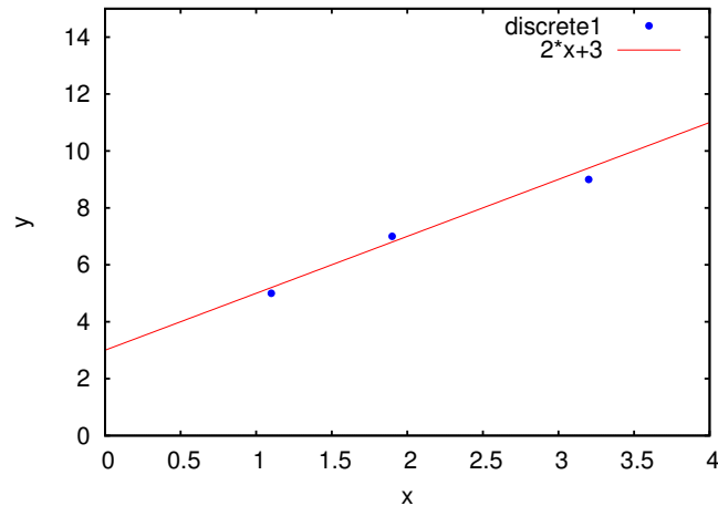
Figura A.5.: Gráfico de um conjunto de 3 pontos, conjuntamente com uma reta.
