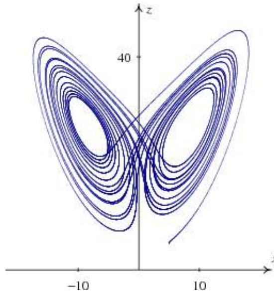
Figura 12.8.: Solução caótica do sistema de Lorenz, projetada no plano xz . Os parâmetros são os mesmos da figura 12.7, com x(0) = 5 .
