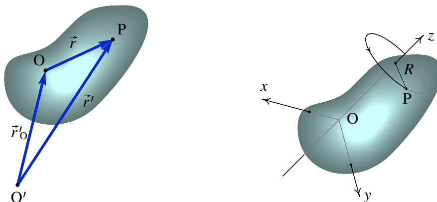
Figura 6.6.: O movimento de translação de um corpo rígido é a variação do vetor posição \vec{r}'_O de um ponto O do corpo e o movimento de rotação é a variação dos vetores posição \vec{r} dos pontos do corpo em relação ao ponto O.
