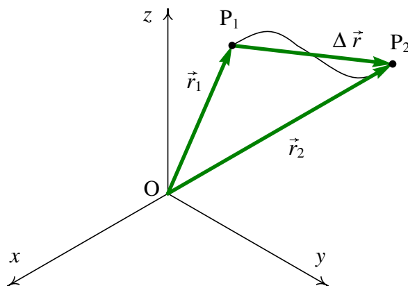
Figura 2.5.: Trajetória de um ponto e deslocamento \Delta \vec{r} entre dois instantes t_1 e t_2 .
