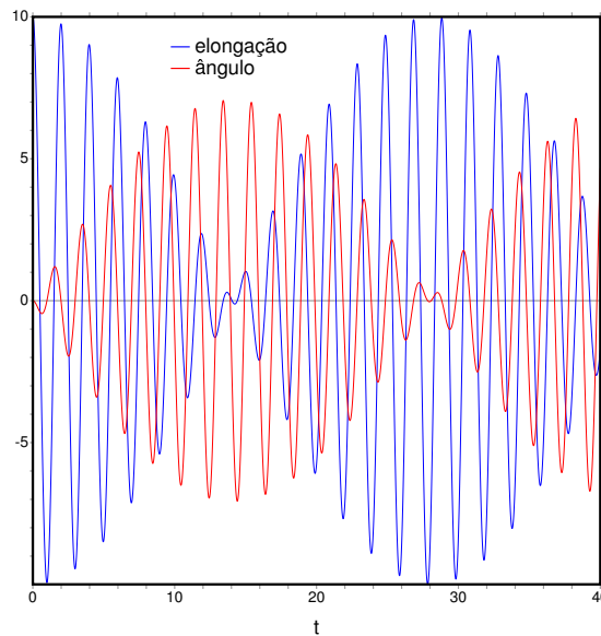
Figura 10.6.: Evolução da elongação e do ângulo de rotação no pêndulo de Wilberforce.
