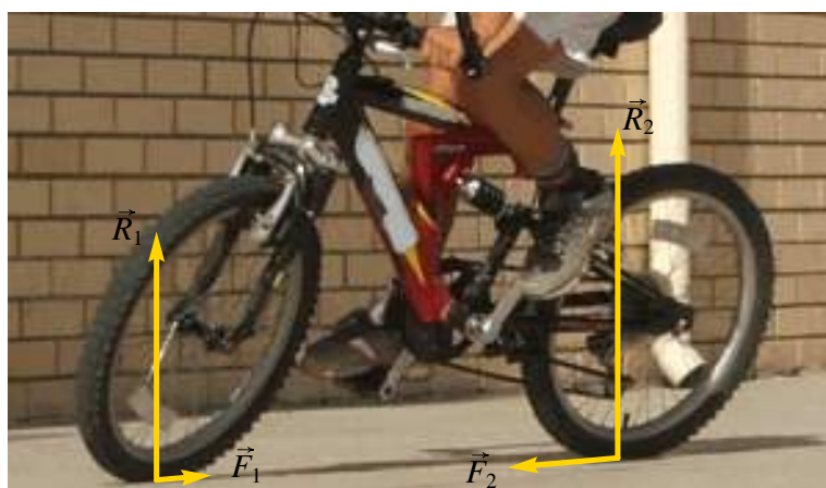
Figura 4.7.: Forças de atrito entre os pneus de uma bicicleta e a estrada.
