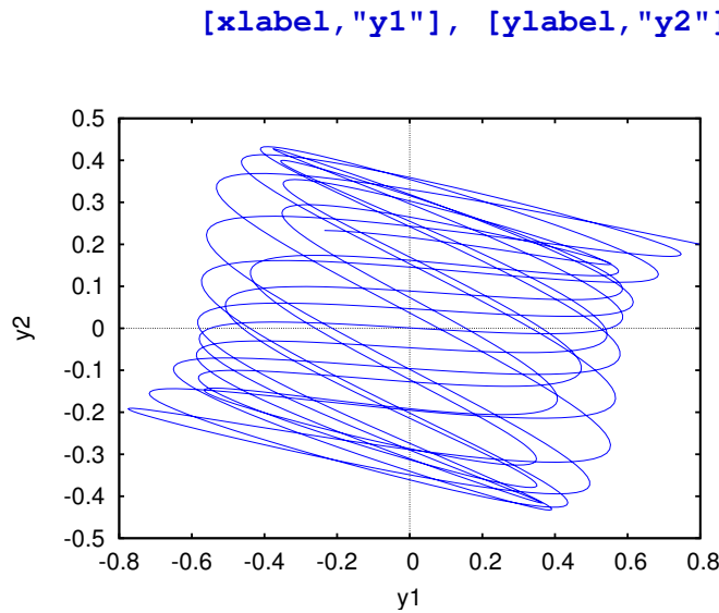
Figura 10.4.: Trajetória do sistema de duas molas no espaço de fase, projetada no plano (y_1, y_2) .
