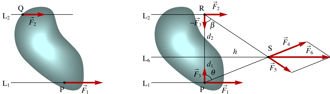
Figura 6.3.: Adição de forças paralelas.
