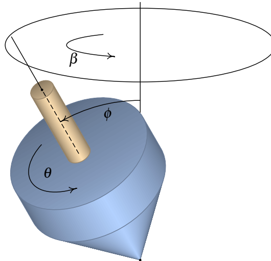
Figura 6.8.: Para definir a orientação de um corpo rígido, são precisos 3 ângulos e à variação de cada um deles corresponde uma velocidade angular.
