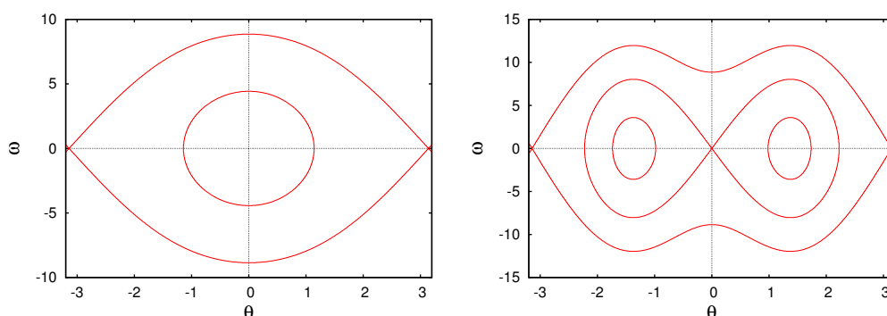
Figura 12.4.: Retrato de fase dum pêndulo com l = 0.5 m, quando a velocidade angular \omega_b da base é igual a 2 \text{ s}^{-1} (lado esquerdo) e 10 \text{ s}^{-1} (lado direito).
