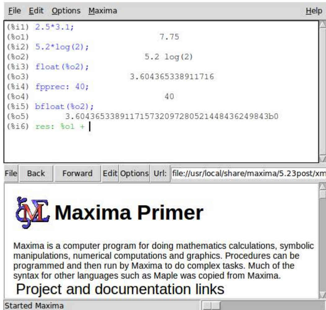
Figura A.1.: A interface gráfica xmaxima .
