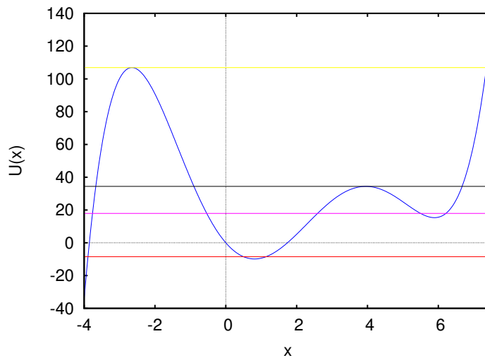
Figura 7.10.: Gráfico da energia potencial no exemplo 7.2, mostrando alguns níveis de energia mecânica.
