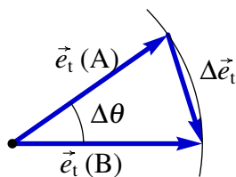
Figura 3.3.: Versores tangenciais em dois instantes diferentes.
