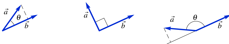
Figura 2.10.: O produto escalar entre dois vetores é positivo se o ângulo entre os vetores for agudo, nulo se os vetores forem perpendiculares, ou negativo, se o ângulo for obtuso.
