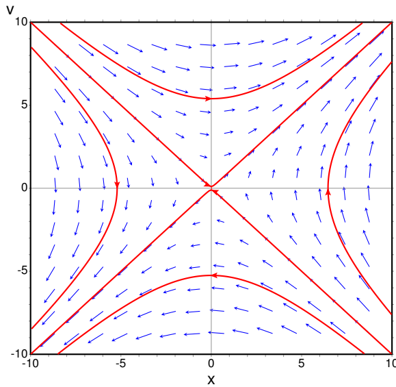
Figura 8.10.: Retrato de fase do oscilador invertido.
