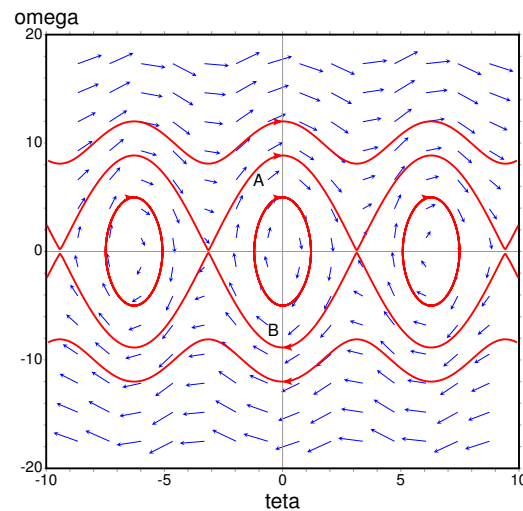
Figura 9.4.: Retrato de fase do pêndulo.
