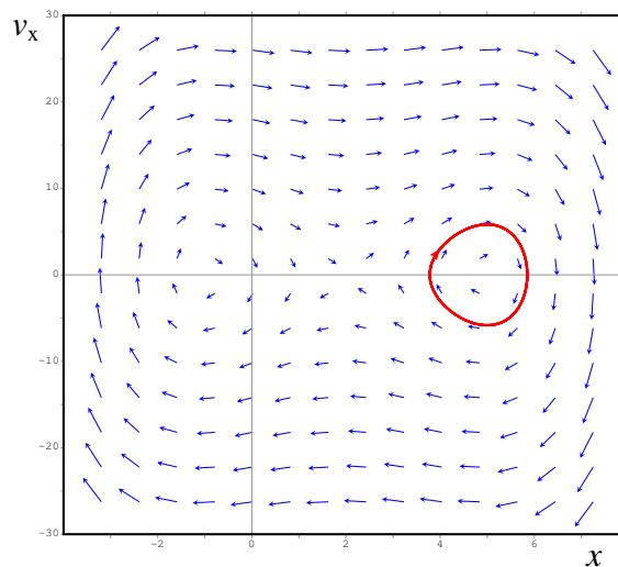
Figura 7.4.: Campo de direções do exemplo 7.1 e curva de evolução do sistema.
