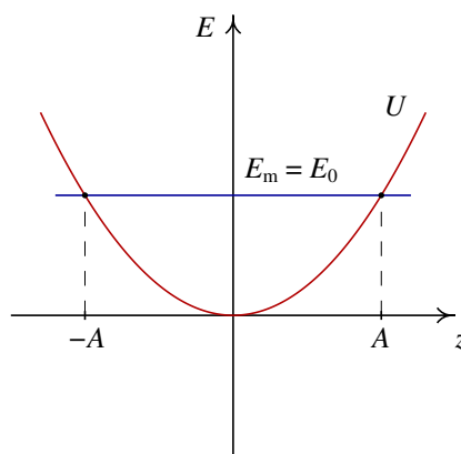
Figura 5.4.: Energia potencial e energia mecânica de um corpo pendurado de uma mola vertical.
