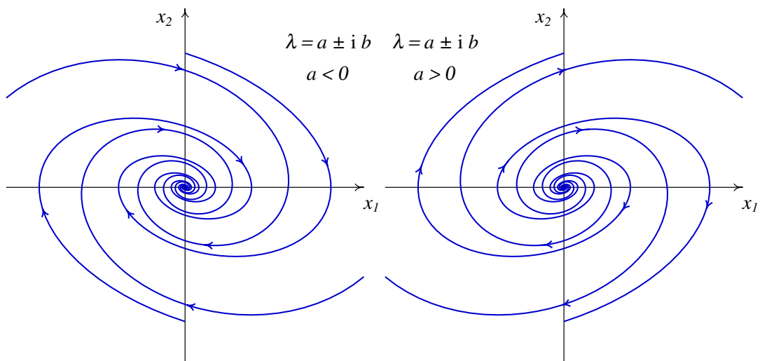
Figura 8.7.: Quando os valores próprios são complexos, o ponto de equilíbrio é um foco, estável (esquerda) ou instável (direita).
