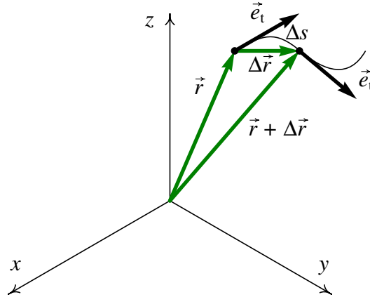
Figura 3.2.: Vetor deslocamento entre dois pontos numa trajetória. Os vetores posição, \vec{r} e \vec{r} + \Delta\vec{r} dependem da origem escolhida, mas o deslocamento \Delta\vec{r} não.
