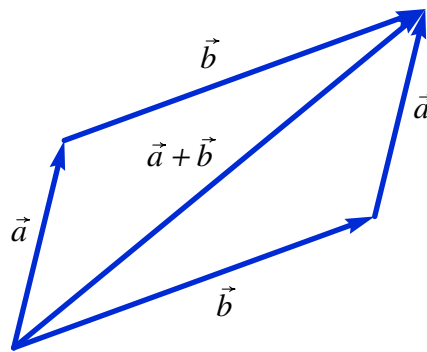
Figura 2.2.: Regra do paralelogramo para somar vetores.
