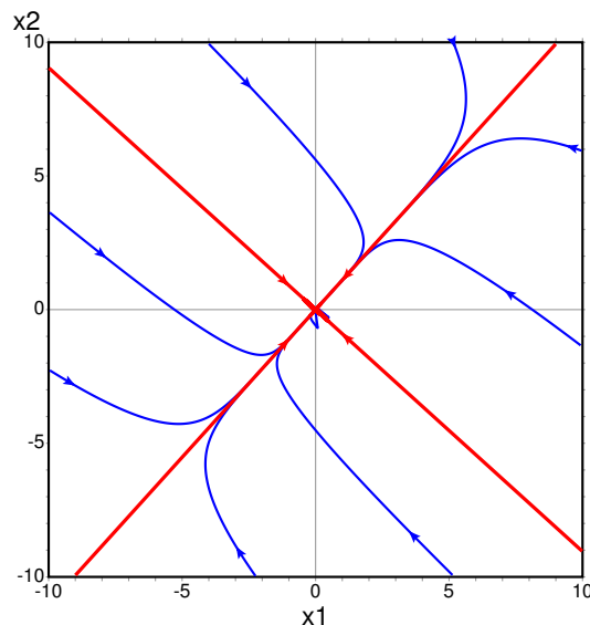
Figura 8.3.: Retrato de fase do exemplo 8.2. As duas retas, estão nas direções dos dois vetores próprios.
