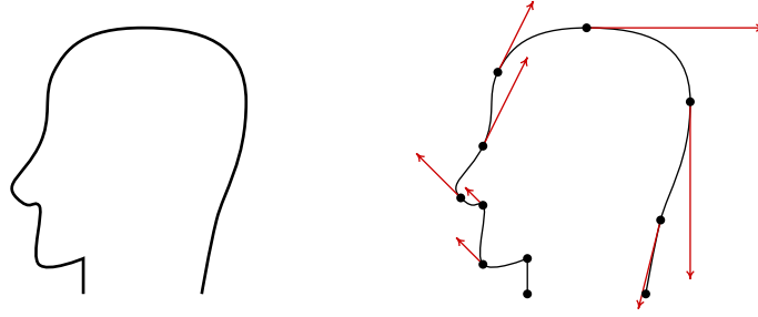
Figura 3.7.: Modelação de uma curva por meio de curvas de Bézier.
