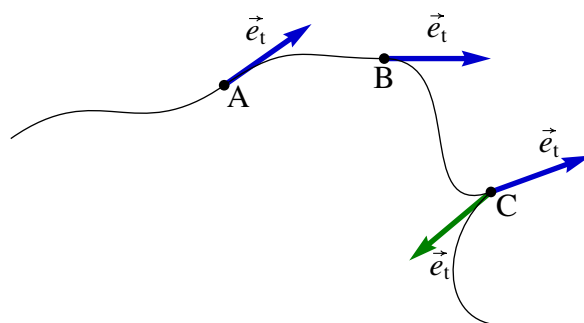
Figura 3.1.: Versor tangencial \vec{e}_t em três pontos da trajetória.
