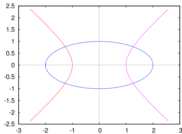
Figura 9.1.: Os pontos de equilíbrio são os pontos de interseção entre as curvas onde cada uma das funções é nula.
