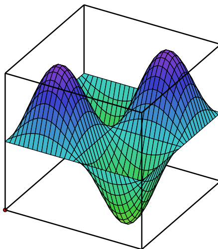
Figura A.7.: Gráfico da função \sin(x)\sin(y) , produzido por Xmaxima.
