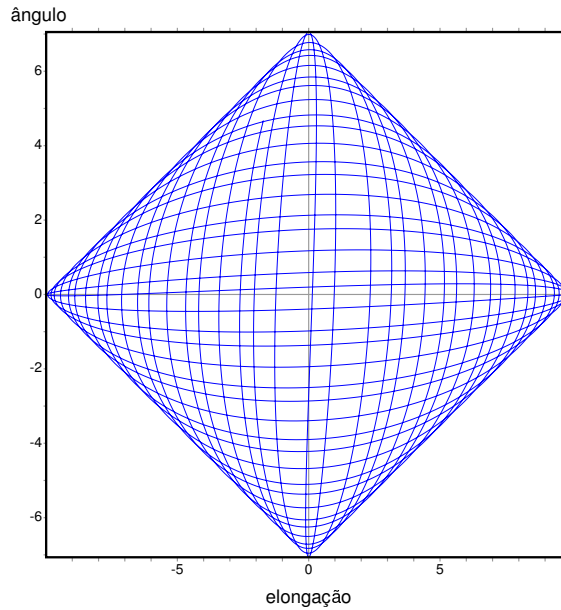
Figura 10.7.: Solução do sistema, no plano formado pela elongação e o ângulo.
