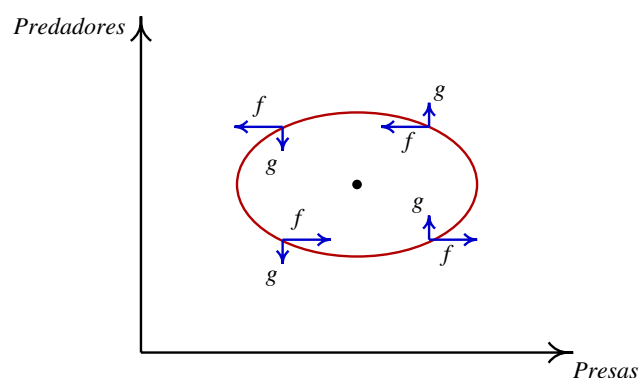
Figura 11.6.: Possível ciclo num sistema predador presa.
