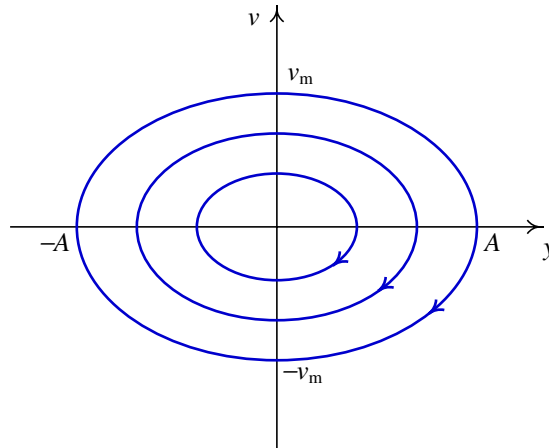
Figura 8.11.: As curvas de evolução do oscilador harmónico simples são todas ciclos.
