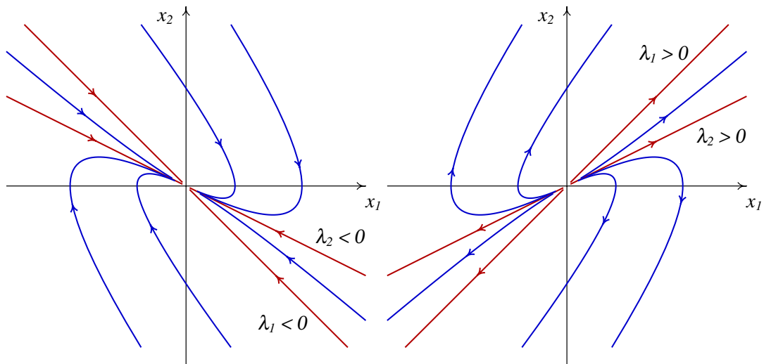
Figura 8.6.: Quando existem dois valores próprios reais, diferentes, com o mesmo sinal, o ponto de equilíbrio é um nó, estável (esquerda) ou instável (direita).
