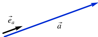
Figura 2.3.: A direção e sentido de um vetor \vec{a} pode ser indicada por um versor \vec{e}_a , com módulo igual a um.
