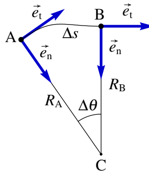
Figura 3.5.: Relação entre o ângulo de rotação da trajetória, o raio de curvatura e a distância percorrida.
