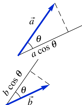
Figura 2.9.: Dois vetores \vec{a} e \vec{b} e o ângulo \theta entre as suas direções.
