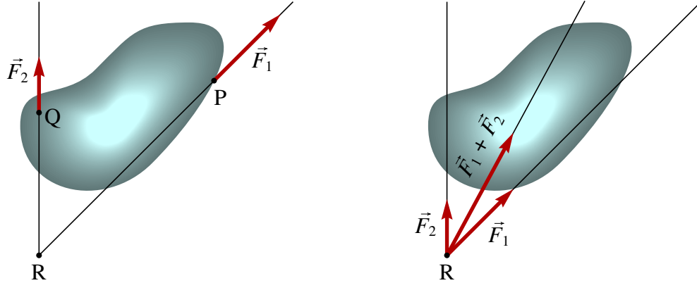
Figura 6.2.: Adição de forças com linhas de ação que se cruzam num ponto comum.
