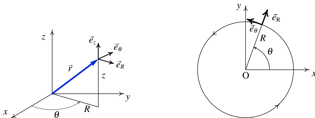
Figura 6.7.: Coordenadas cilíndricas e vista perpendicular ao plano xy do movimento de rotação de um ponto no corpo rígido.
