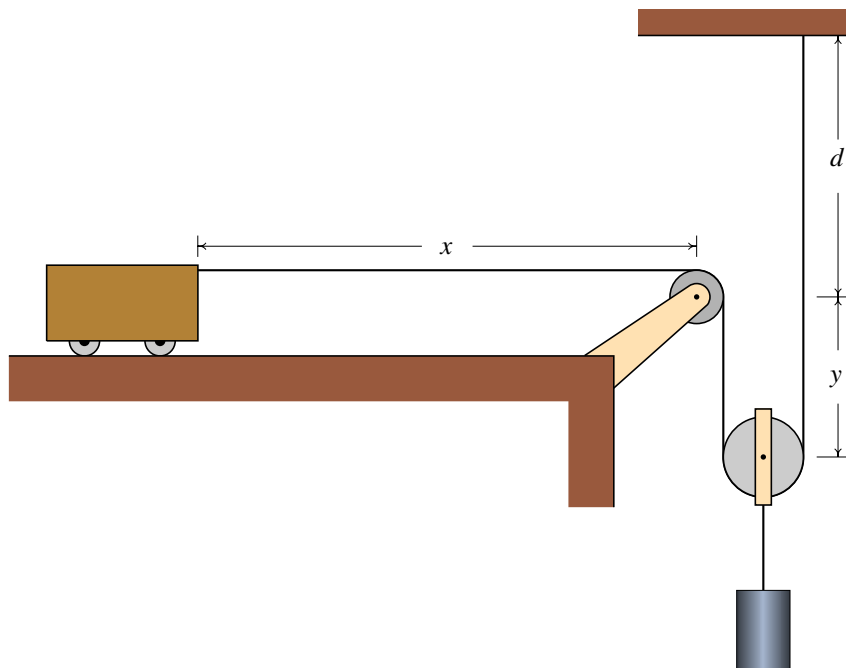
Figura 2.11.: Sistema com dois movimentos dependentes e um único grau de liberdade.
