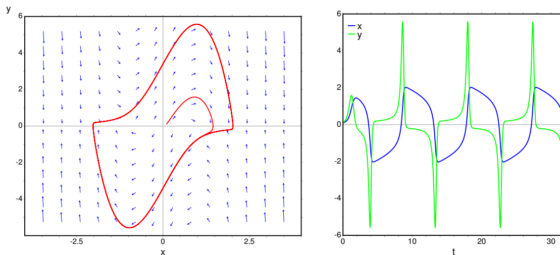
Figura 11.3.: Solução da equação de van der Pol para um valor elevado do parâmetro \varepsilon = 1.7 e com estado inicial próximo da origem.
