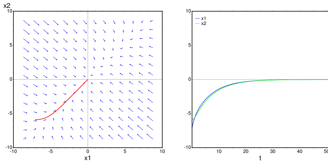
Figura 8.4.: Curva de evolução e temperaturas em função do tempo, quando as duas temperaturas iniciais são de 8^\circ \text{C} .
