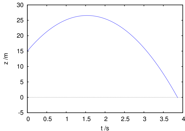
Figura 3.9.: Altura da esfera do exemplo 3.3, em função do tempo.
