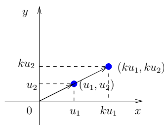
Figura 1.8: Multiplicação de vectores de \mathbb{R}^2 pelo escalar k > 0 .
