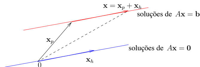
Figura 3.7: A solução geral de um sistema não homogêneo.
