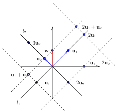
Figura 1.11: Combinação linear de vetores de \mathbb{R}^2 . O vector \mathbf{w} é \mathbf{w} = \frac{1}{2}\mathbf{u}_1 + \mathbf{u}_2 .
