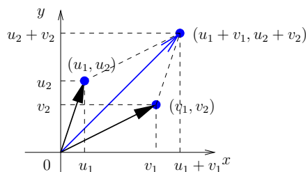
Figura 1.7: Adição de vectores de \mathbb{R}^2 .
