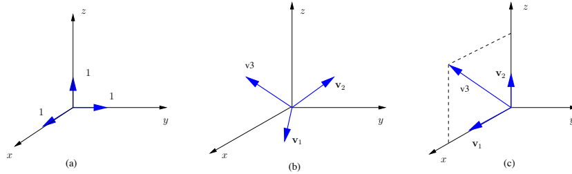
Figura 3.3: (a) Base canónica de \mathbb{R}^3 : \{(1, 0, 0), (0, 1, 0), (0, 0, 1)\} ; (b) \{\mathbf{v}_1, \mathbf{v}_2, \mathbf{v}_3\} é uma base de \mathbb{R}^3 ; (c) \{\mathbf{v}_1, \mathbf{v}_2, \mathbf{v}_3\} não é uma base de \mathbb{R}^3 .
