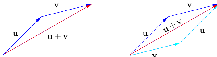
Figura 1.3: A soma u + v e u + v = v + u .
