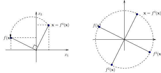
Figura 4.3: A função f(\mathbf{x}) = A\mathbf{x} , em que A tem valores próprios \pm i representa uma rotação em \mathbb{R}^2 .
