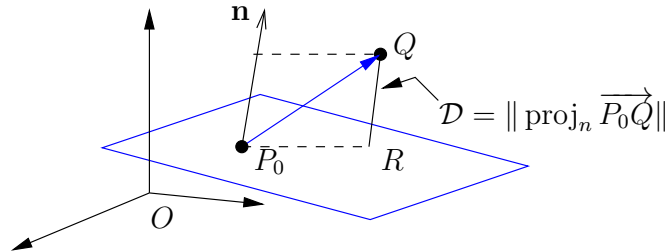
Figura 5.13: Sendo \mathbf{n} um vector normal ao plano, \mathcal{D} designa a distância de Q ao plano.
