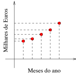
Figura 5.18: Dados do Exemplo 5.19.
