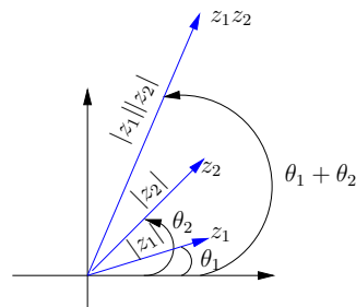
Figura A.3: O produto de dois complexos.
