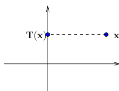
Figura 6.6: Projectção ortogonal sobre o eixo dos yy .
