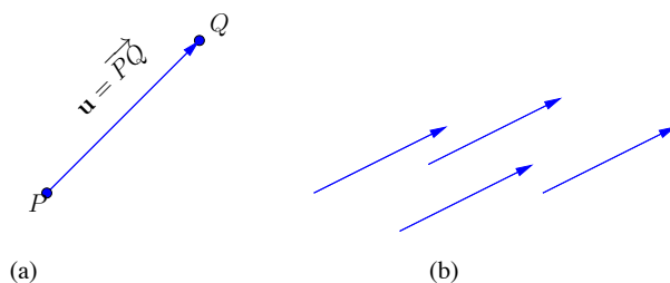
Figura 1.2: (a) O vector \mathbf{u} é representado pelo segmento orientado \overrightarrow{PQ} . (b) Vectores equivalentes.
