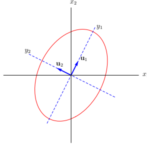
Figura 7.4: Elipse cujos eixos têm as direcções dos vectores próprios (unitários) u_1 e u_2 da matriz A do Exemplo 7.7.
