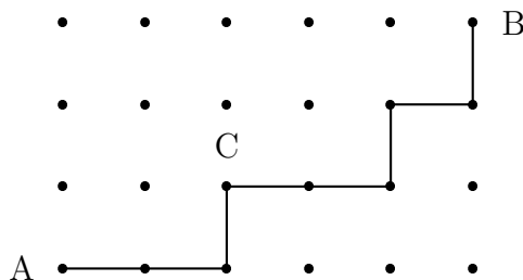
Figure 4.1: Path EENEENEN
