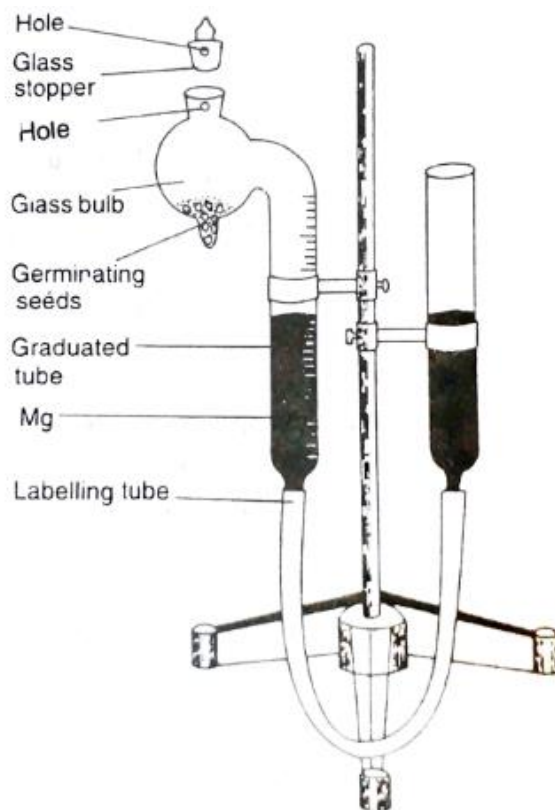
Fig: 5.6. Ganong's respirometer
