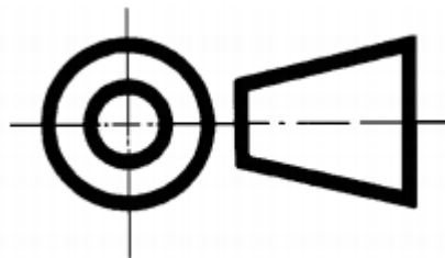
FIGURA 21 - REPRESENTAÇÃO ORTOGRÁFICA PELO MÉTODO DO 3º DIEDRO
