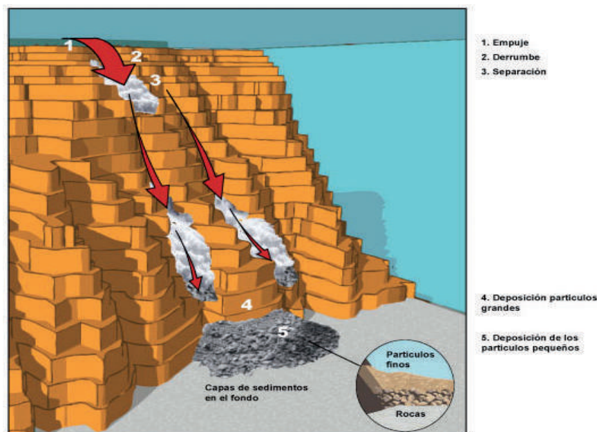
Figura 1.14. Cañón submarino resultado de la acción erosiva de las corrientes de turbidez.
