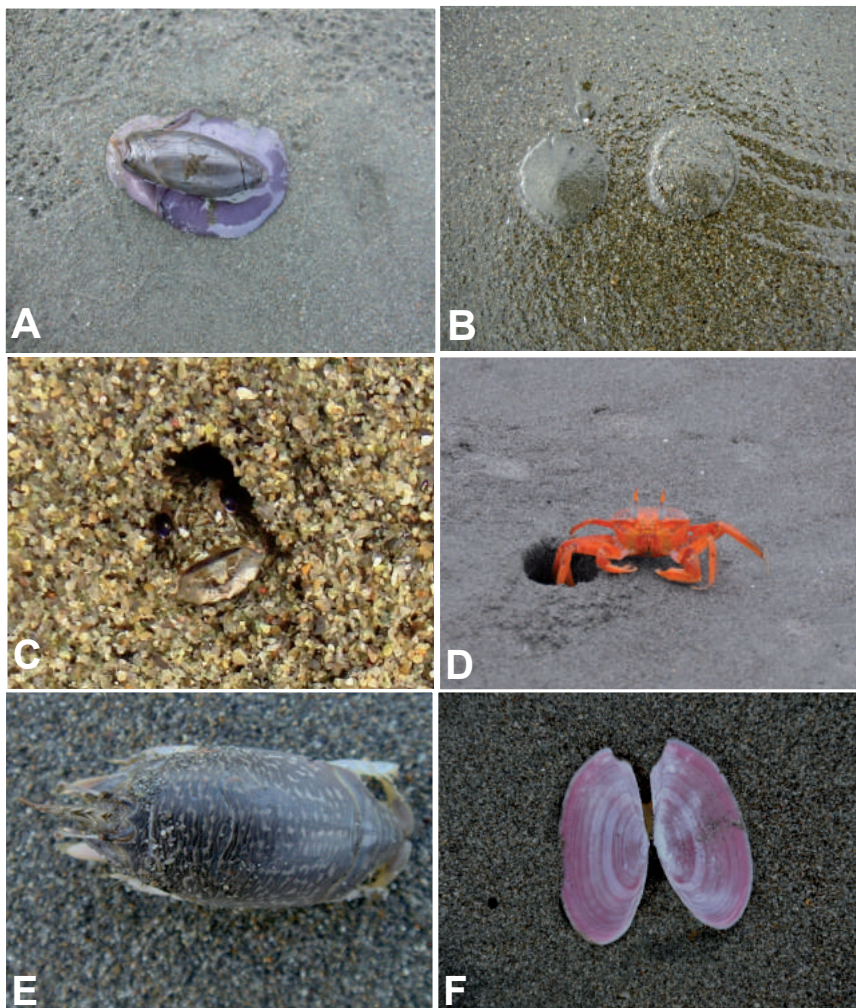
Figura 3.5. Fauna de las playas arenosas. A: Oliva de playa ( Agaronia sp.), B: Dólar de mar ( Encope sp.), C: Pez gobiidae que vive en agujero de la arena, D: Cangrejo fantasma ( Ocypode sp.), E: Crustáceo de playa “Reculambai” ( Emerita sp.), F: Tellina sp. Bivalvo que habita en zonas arenosas sumergidas a poca profundidad. Cortesía: Jaime Cantera Kintz.
