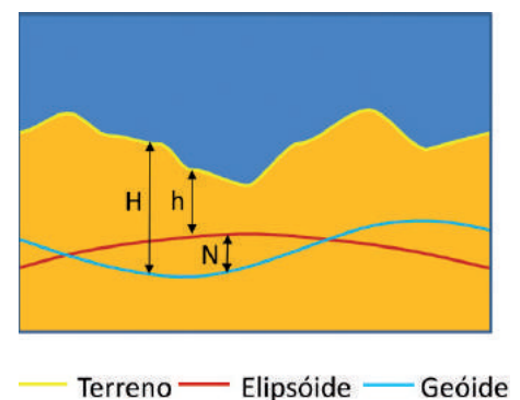
Figura 1.34. Modelo geodésico general. Fuente: El autor.
