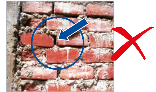
Figura 22 Fraguado deficiente. Zona débil susceptible al agrietamiento.
