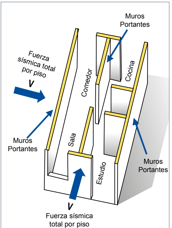
Figura 11 Efectos de un sismo en una vivienda: Fuerzas horizontales actuando sobre ella.
