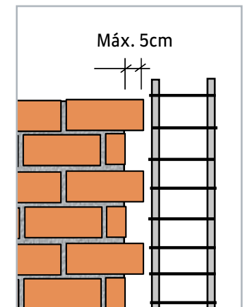
Figura 23 Longitud del diente
