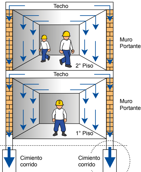
Figura 10 Proceso de transferencia de cargas.
