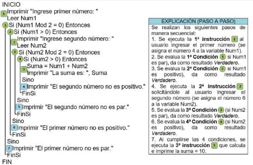
Figura 126. Primer seguimiento a una estructura de decisión anidada.
