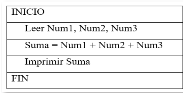
Figura 17. Tercer ejemplo de un algoritmo en diagramación rectangular.
