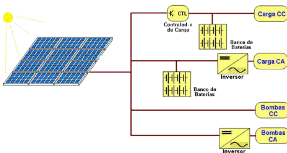
Figura 78: Possíveis configurações para um sistema fotovoltaico offgrid , disponível em: < http://cresesb.cepel.br/index.php?section=com_content&cid=341 >, acesso em 14/07/2016.
