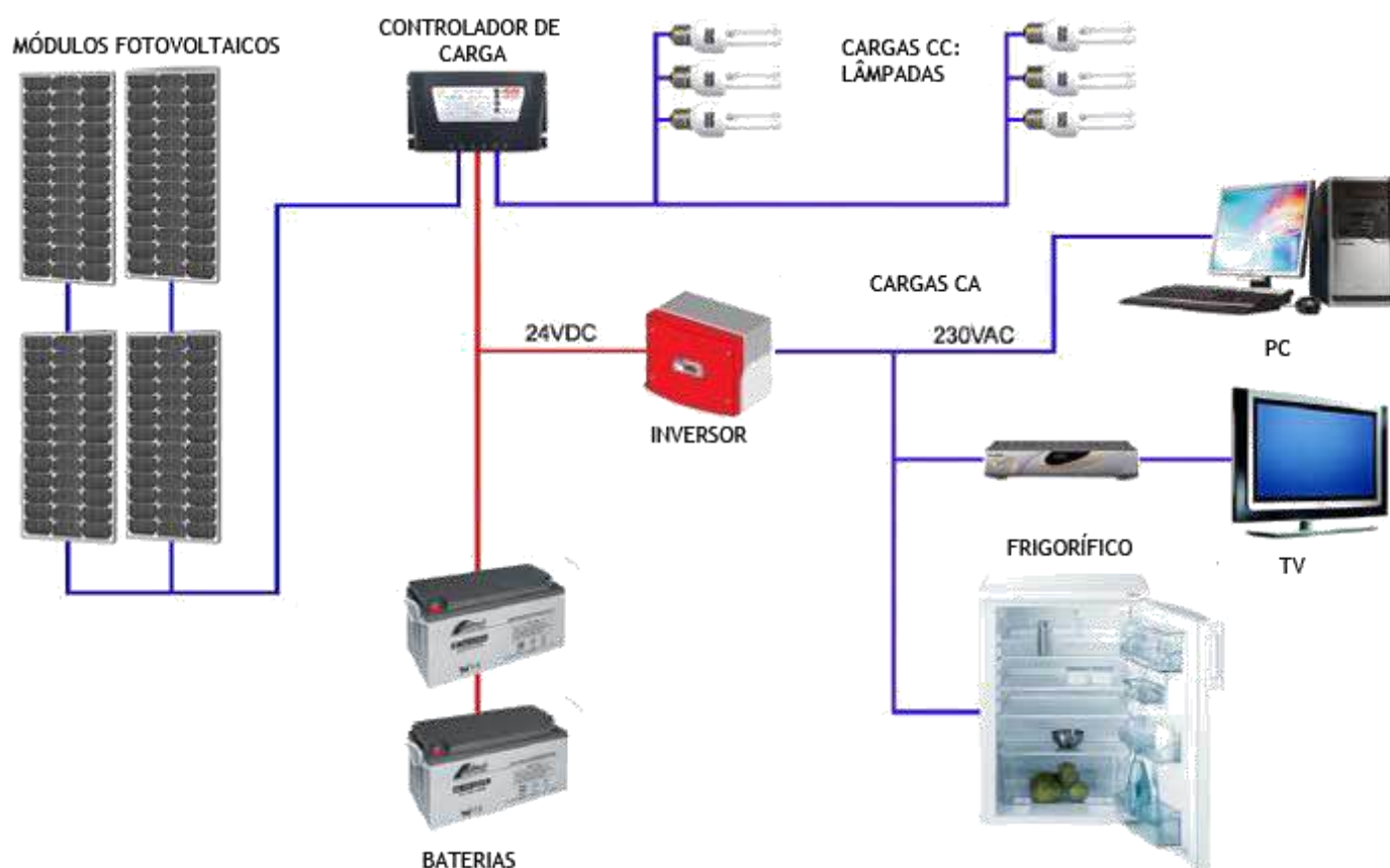
Figura 75: representação esquemática do fluxo de energia em um sistema fotovoltaico autônomo, disponível em: < http://www.metalica.com.br/energia-a-abundancia-solar >, acesso em 14/07/2016.
