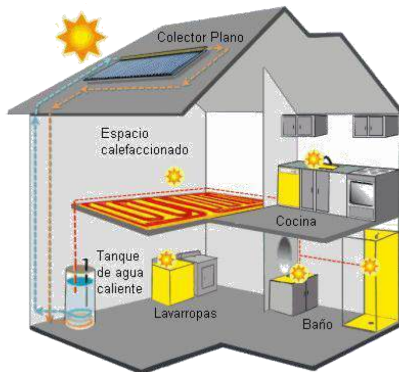
Figura 8: Energia solar térmica destinada a aplicações residenciais, disponível em: < http://javiponce-formatec.blogspot.com.br/2012_01_01_archive.html >. Acesso em 02/06/2016.
