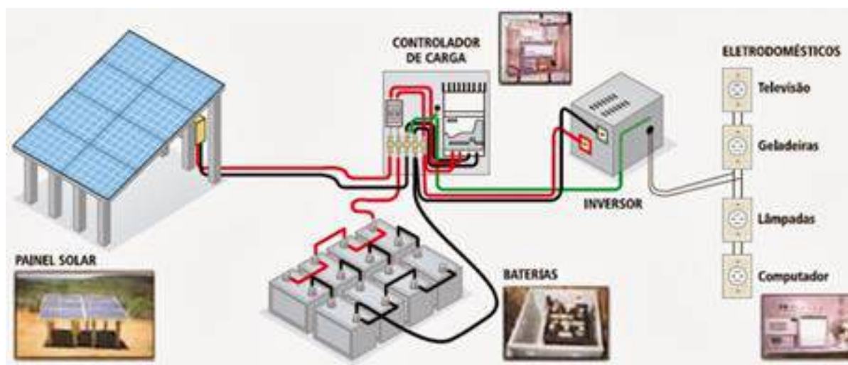
Figura 21: Representação esquemática de um sistema fotovoltaico não conectado à rede, disponível em: < http://www.reformaai.com/2013/10/energia-fotovoltaica.html >. Acesso em 02/06/2016.
