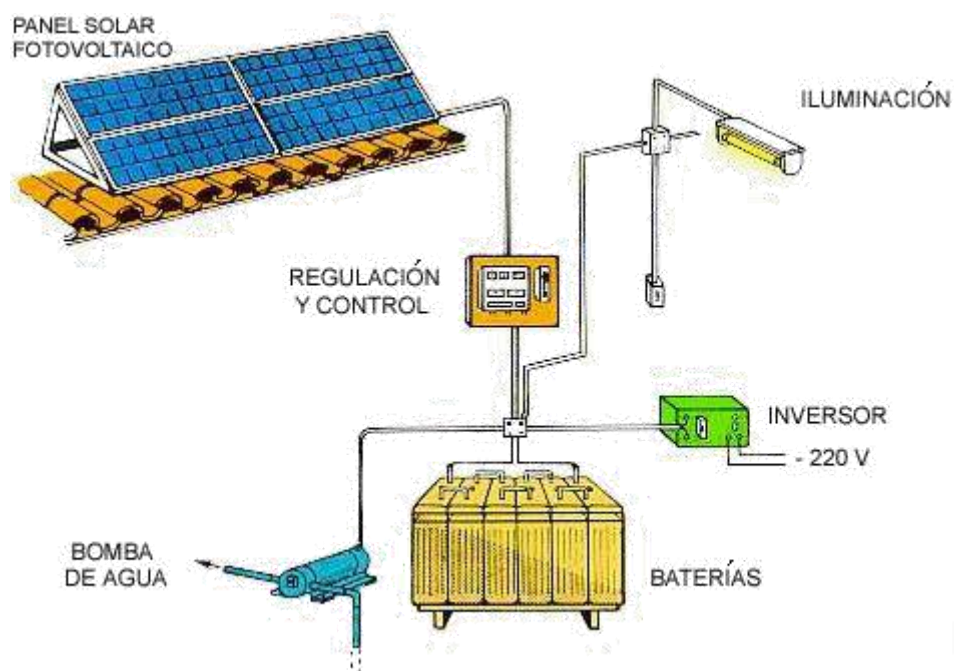
Figura 79: Sistema FV autônomo alimentando circuito de iluminação e bomba de água em CC, disponível em: < http://www.diariodeciencias.com.ar/energia-solar-fotovoltaica-y-termica-diferencias-y-aplicaciones/ >, acesso em 14/07/2016.
