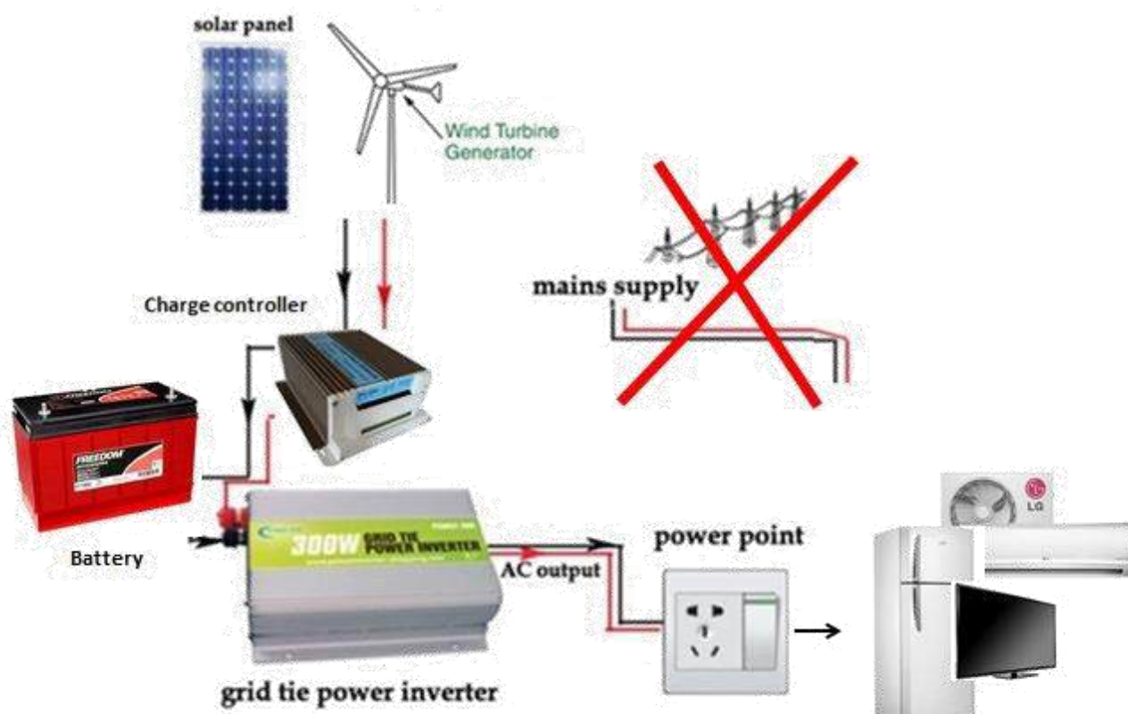
Figura 96: Exemplo de sistema híbrido off grid, disponível em: < http://produto.mercadolivre.com.br/MLB-713979351-kit-off-eolico-aerogerador-ista-500w-inversor-controlador- JM >, acesso em 15/07/2016.
