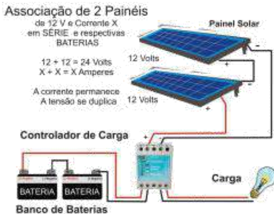
Figura 62: Exemplo de instalação FV utilizando painéis conectados em série, disponível em: < http://www.sunlab.com.br/Dimensionamento_solar_fotovoltaico.htm >. Acesso em 03/06/2016.
