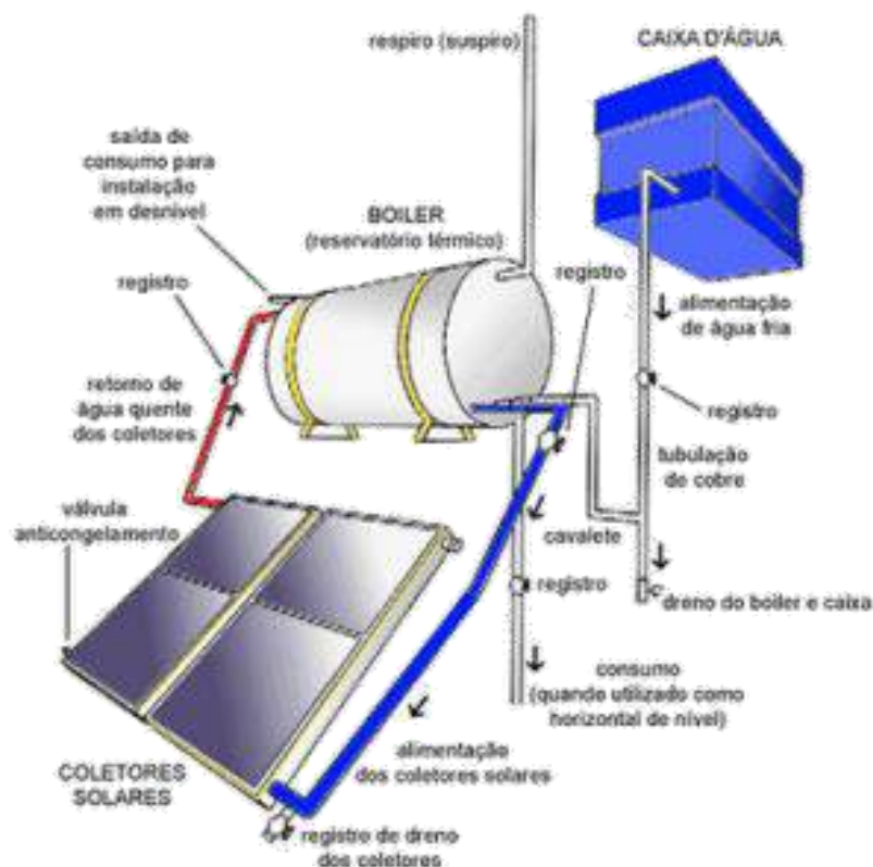
Figura 7: Representação esquemática de sistema de aquecimento térmico, disponível em: < http://www.upf.br/comarte/?p=737 >. Acesso em 02/06/2016.
