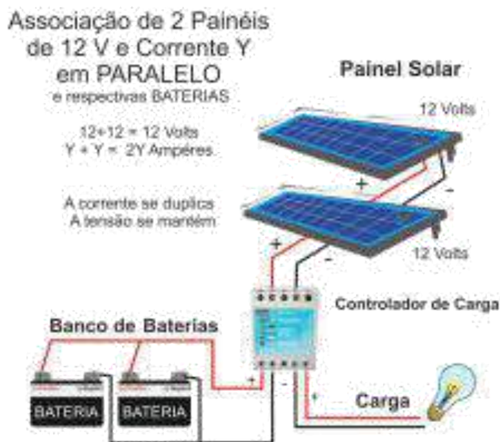
Figura 65: Exemplo de instalação FV utilizando painéis conectados em paralelo, disponível em: < http://www.sunlab.com.br/Dimensionamento_solar_fotovoltaico.htm >. Acesso em 03/06/2016.
