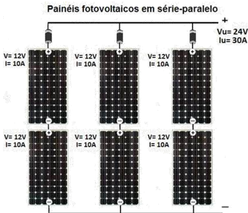
Figura 67: Exemplo de conexão de painéis FV em série-paralelo, disponível em: < https://br.pinterest.com/pin/527976756291607681/ >. Acesso em 03/06/2016.
