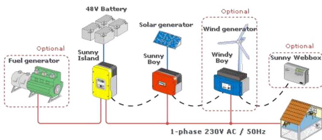
Figura 97: Sistema de geração híbrida com múltiplos inversores, disponível em: < http://personal.unizar.es/rdufo/index.php?option=com_content&view=article&id=13:sistemas-hibridos&catid=10&Itemid=120&lang=es >, acesso em 15/07/2016.
