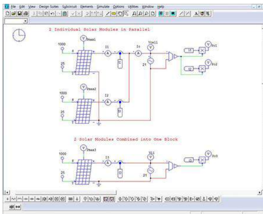
Figura 105: Exemplo de simulação fotovoltaica utilizando o software PSIM , disponível em: < http://www.powersimtech.co.kr/category/ren_energy_package >, acesso em 22/08/2016.
