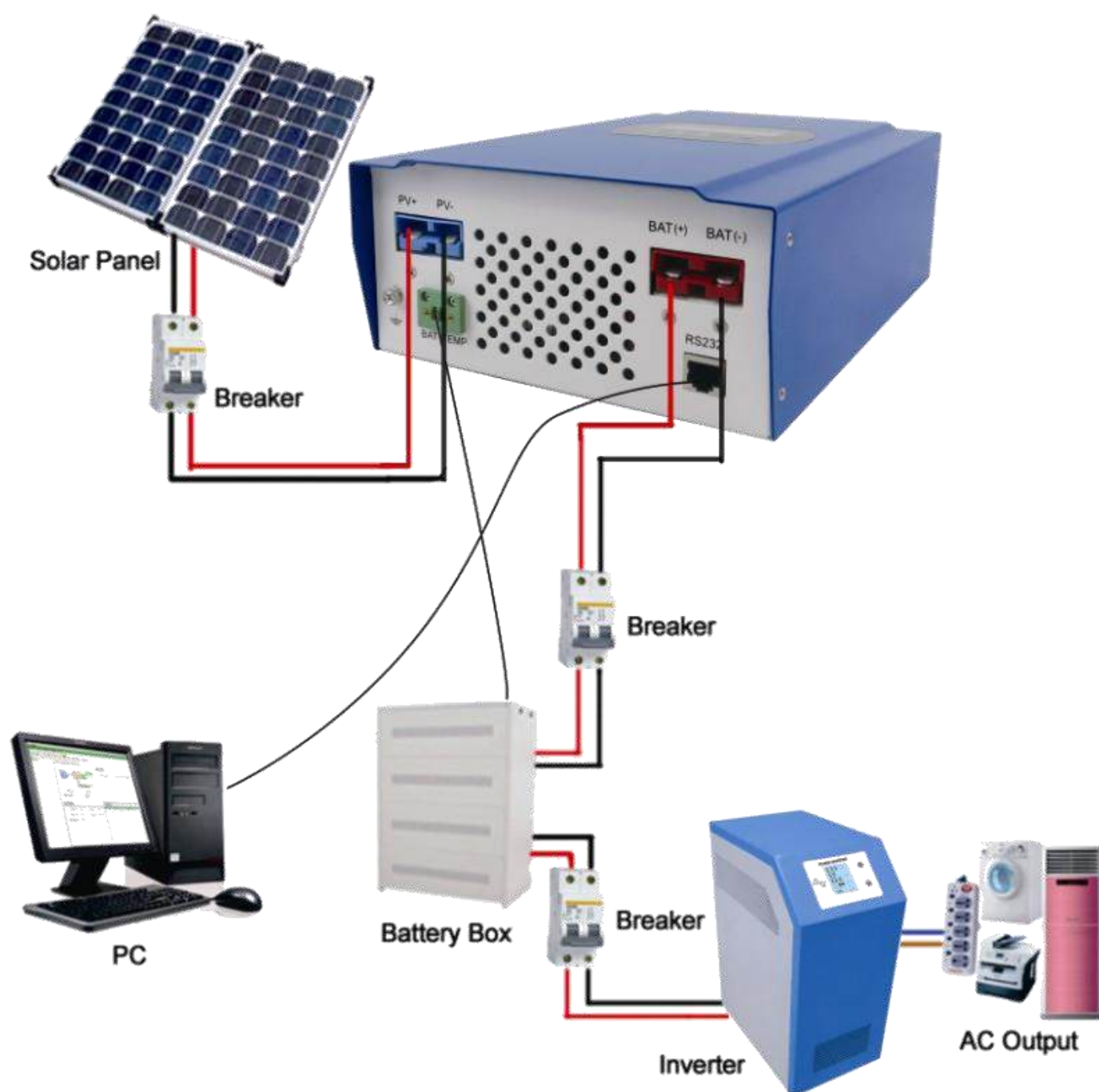
Figura 82: Exemplo das ligações em um controlador de carga destinado a sistemas fotovoltaicos autônomos, disponível em: < >, acesso em 14/07/2016.
