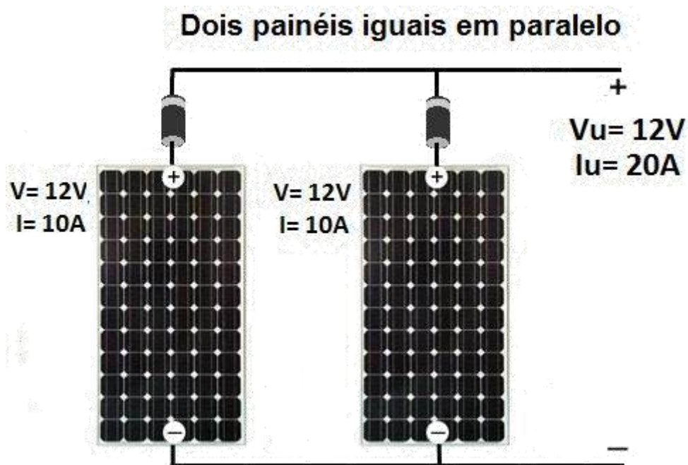
Figura 63: Exemplo de conexão paralela de painéis com as mesmas especificações elétricas, disponível em: < https://br.pinterest.com/pin/527976756291607681/ >. Acesso em 03/06/2016.
