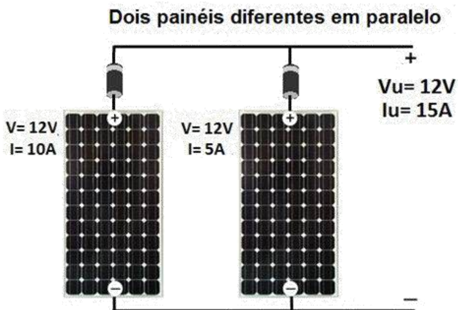
Figura 64: Exemplo de conexão paralela entre painéis com especificações elétricas distintas, disponível em: < http://www.mpptsolar.com/pt/paineis-solares-em-paralelo.html >. Acesso em 03/06/2016.
