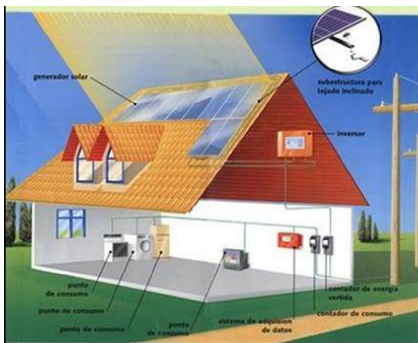
Figura 22: Exemplo de sistema fotovoltaico aplicado a uma residência, disponível em: < https://www.youtube.com/watch?v=u4wMc05Th3I >. Acesso em 02/06/2016.
