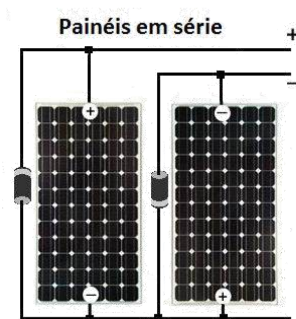
Figura 60: Exemplo de conexão de painéis FV em série, disponível em: < http://www.mpptsolar.com/pt/paineis-solares-em-serie.html >. Acesso em 03/06/2016.
