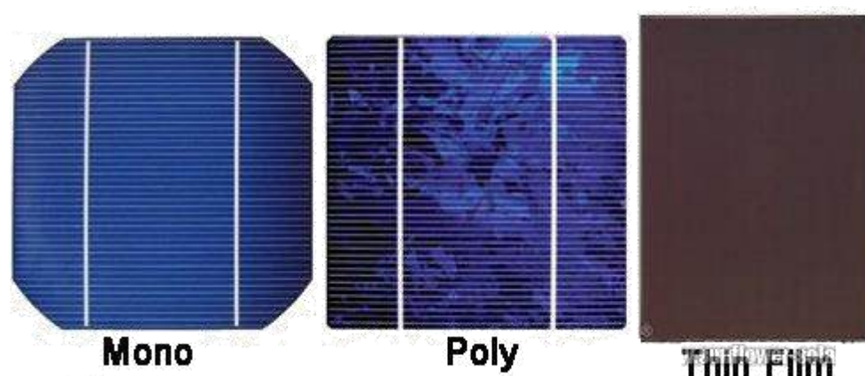
Figura 58: Células de silício monocristalino, policristalino e filme fino, disponível em: < www.sunflower-solar.com >, acesso em 24/06/2016.
