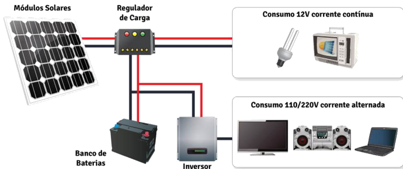
Figura 77: Aplicação FV isolada com consumidores alimentados em corrente contínua e em corrente alternada, disponível em: < http://real-solar.com/como-funciona.php >, acesso em 14/07/2016.
