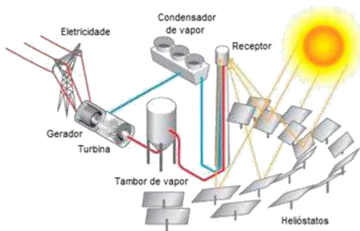
Figura 3: Geração de vapor para acionamento de conjunto turbina + gerador a partir de sistema concentrador do tipo torre, disponível em: < http://focusolar.com.br/concentracao-de-energia-solar-para-geracao-de-potencia-eletrica/ >, acesso em 02/06/2016.
