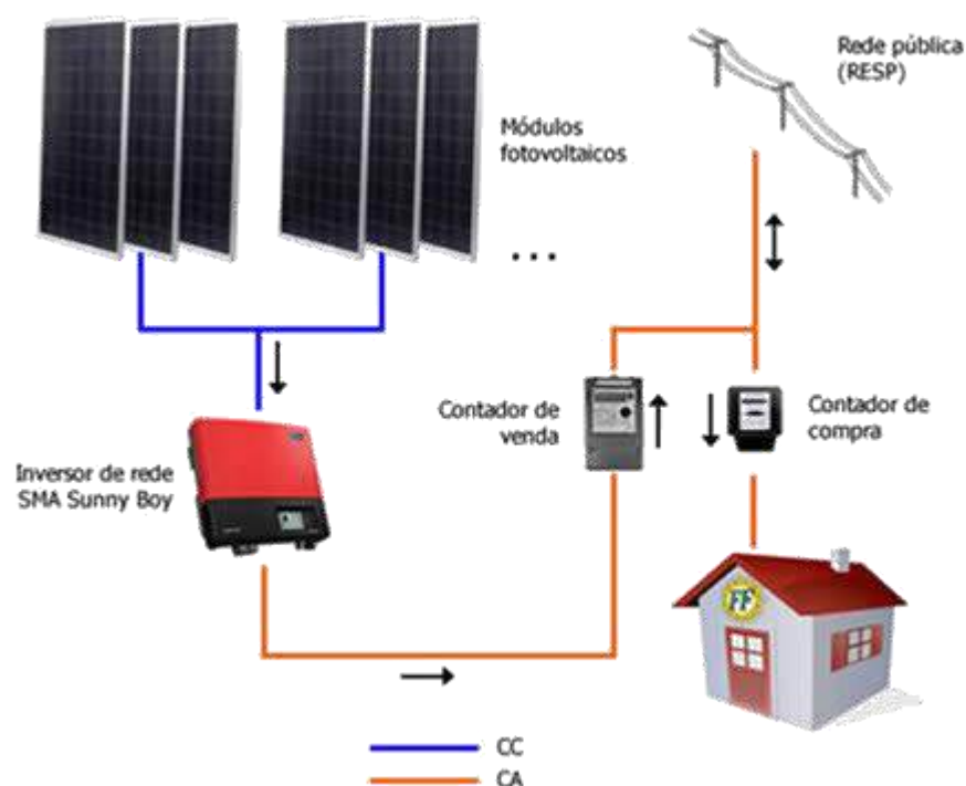
Figura 86: Fluxo de corrente CC e CA em um sistema FV integrado a rede, disponível em: < http://behinniro.com/?category >, acesso em 14/07/2016.
