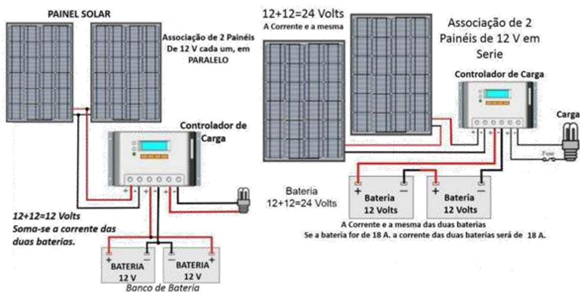
Figura 66: Comparativo entre a conexão de painéis em série ou em paralelo, disponível em: < http://www.osol.com.br/dimensionamento-de-sistema-solar-autonomo-off-grid/ >. Acesso em 03/06/2016.
