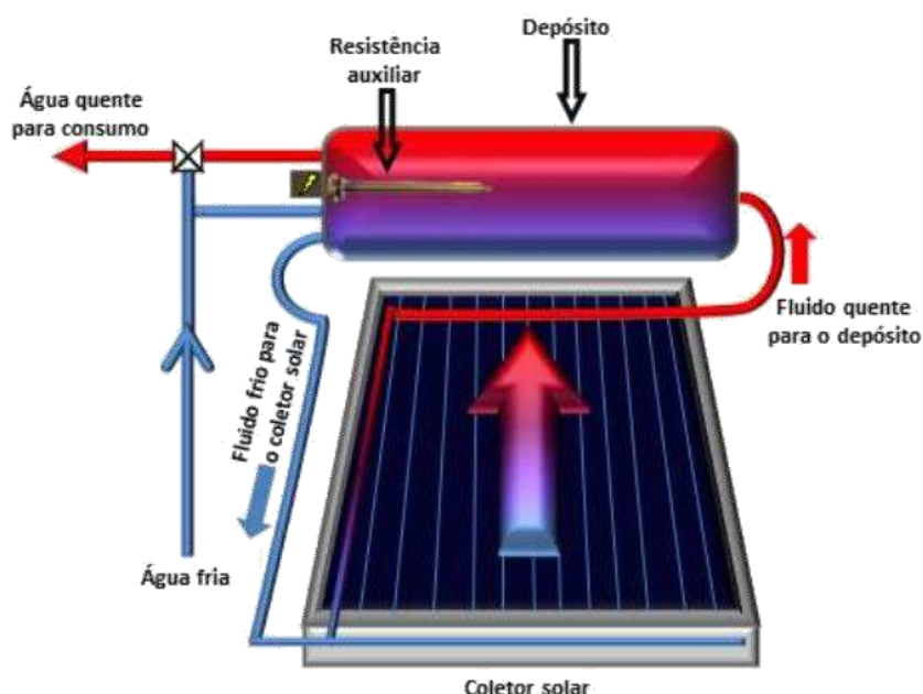
Figura 6: Deslocamento do fluido entre o coletor solar e reservatório térmico, disponível em: < http://pt.slideshare.net/lukeduarte/coletores-solares >. Acesso em 02/06/2016.
