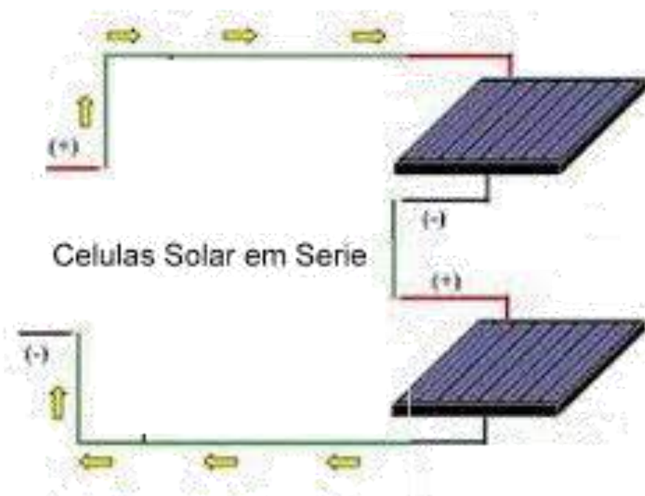
Figura 55: Exemplo de associação de células FV em série, disponível em: < https://plus.google.com/+IbytesBr >. Acesso em 03/06/2016.
