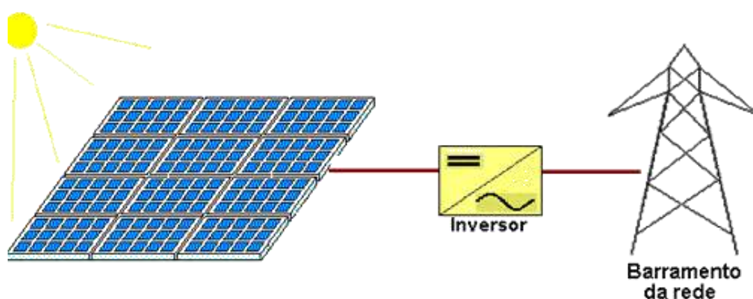
Figura 83: Configuração básica de um sistema FV conectado a rede elétrica de distribuição da concessionária, disponível em: < http://cresesb.cepel.br/index.php?section=com_content&cid=341 >, acesso em 14/07/2016.
