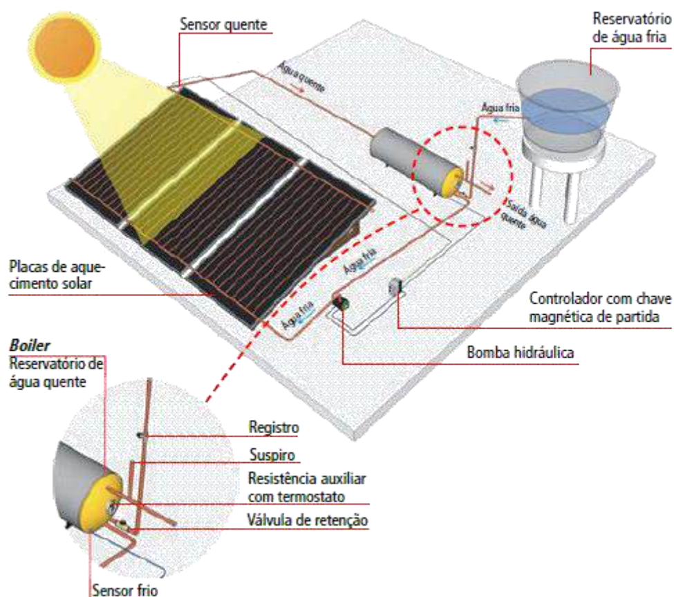
Figura 69: Exemplo de sistema de aquecimento via energia solar térmica utilizando circulação através de bomba hidráulica, disponível em: < http://www.metalica.com.br/energia-a-abundancia-solar >, acesso em 14/06/2016.
