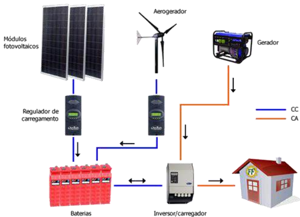
Figura 98: Exemplo de sistema híbrido autônomo, disponível em: < http://www.ffsolar.com/index.php?lang=PT&page=sistemas-autonomos >, acesso em 15/07/2016.
