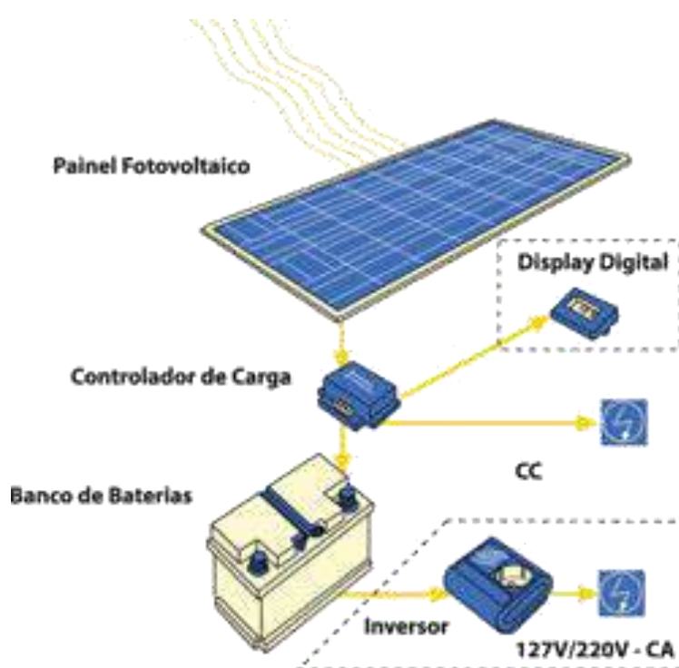
Figura 80: Controlador de carga com display digital, disponível em: < http://www.preservasolar.com.br/s_isolados_minirede.php?act=produtos >, acesso em 14/07/2016.
