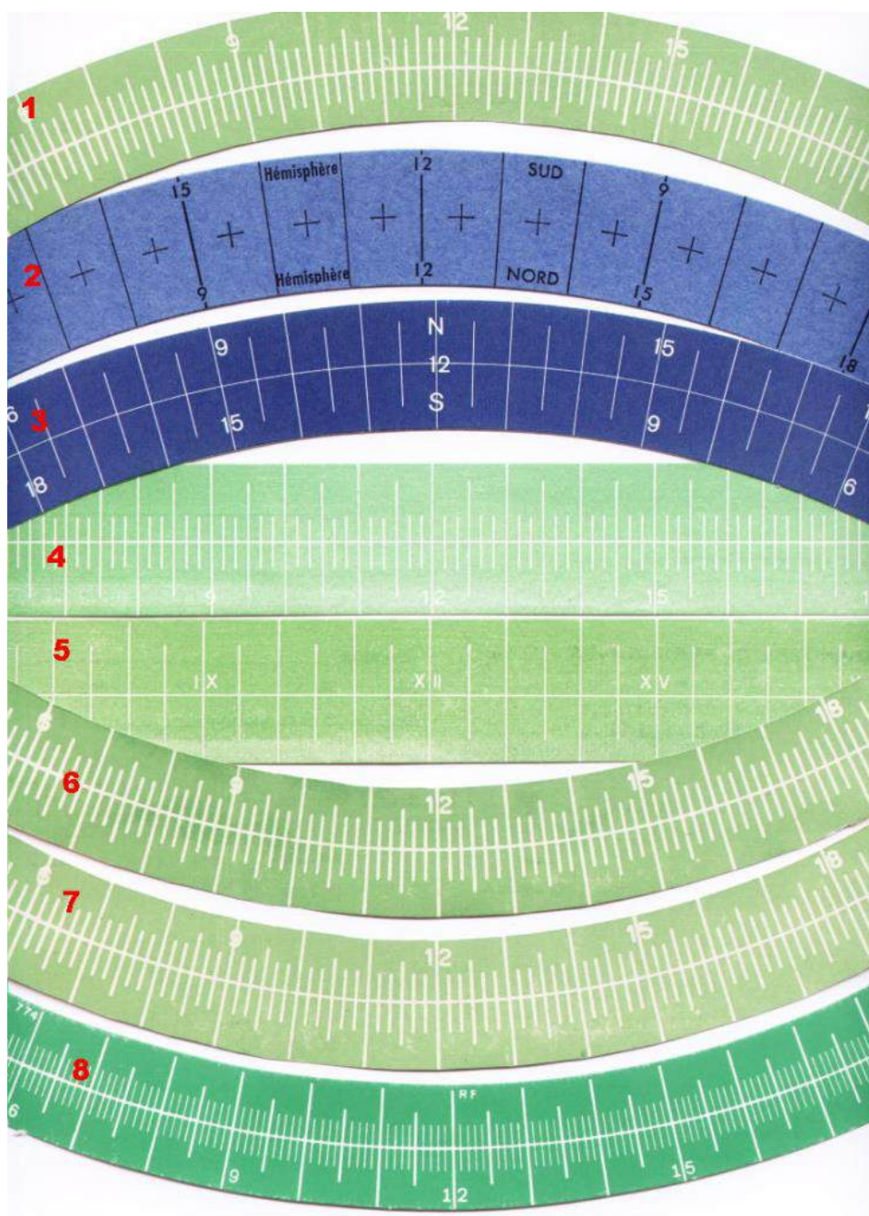
Figura 42: Diferentes modelos de fitas de heliógrafo. 1, 2 e 3 - modelo curva comprida, 4 e 5 modelo reto, 6,7 e 8 - modelo curva curta, disponível em: < http://meteoropole.com.br/2012/03/bola-de-cristal/ >, acesso em 06/05/2016.
