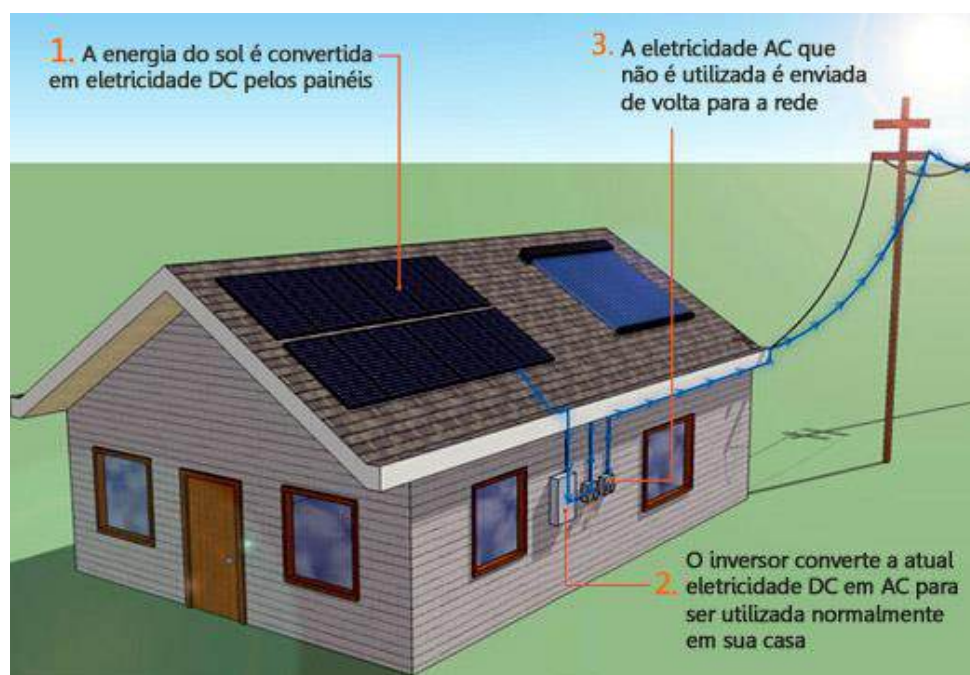
Figura 84: Exemplo de sistema FV interligado a rede, disponível em: < https://www.energiapura.com/content/sistema-solar-fotovoltaico-grid-tie-7-kw >, acesso em 14/07/2016.
