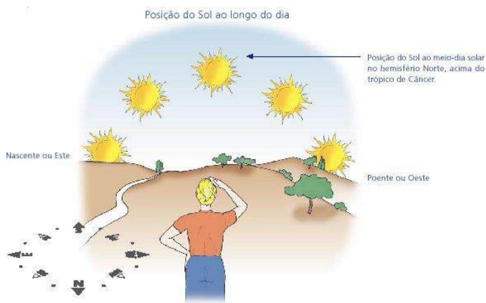
Figura 52: Movimento do sol ao longo do dia, disponível em: < http://www.cienciaviva.pt/equinocio/lat_long/cap4.asp >, acesso 06/05/2016.
