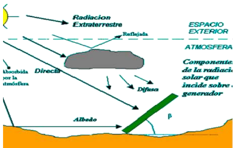
Figura 35: Radiação devido ao albedo incidindo sobre a superfície receptora, disponível em: < http://docplayer.com.br/8204762-Faculdade-de-engenharia-da-universidade-do-porto.html >, acesso 06/05/2016.
