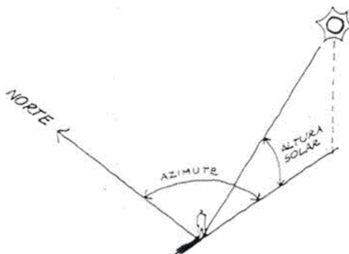
Figura 37: Representação gráfica da altura solar e do ângulo de azimuth, disponível em: < https://radiobarrio.wordpress.com/rain-space/ >, acesso em 06/05/2016.
