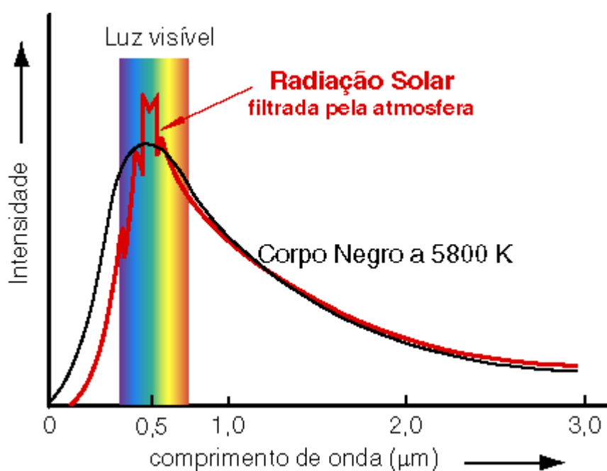
Figura 29: Comportamento da radiação solar em relação a radiação do corpo negro, disponível em: < http://www.oal.ul.pt/vt2004/Venus%20Transit%20Safety_radiacao.htm >, acesso em 05/05/2016.
