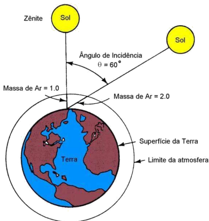
Figura 39: Caminhos distintos que a radiação solar percorre para atravessar a atmosfera, disponível em: < http://docplayer.com.br/8204368-Eee934-impactode-gd-asredes-eletricas-http-www-cpdee-ufmg-br-selenios.html >, acesso em 06/05/2016.
