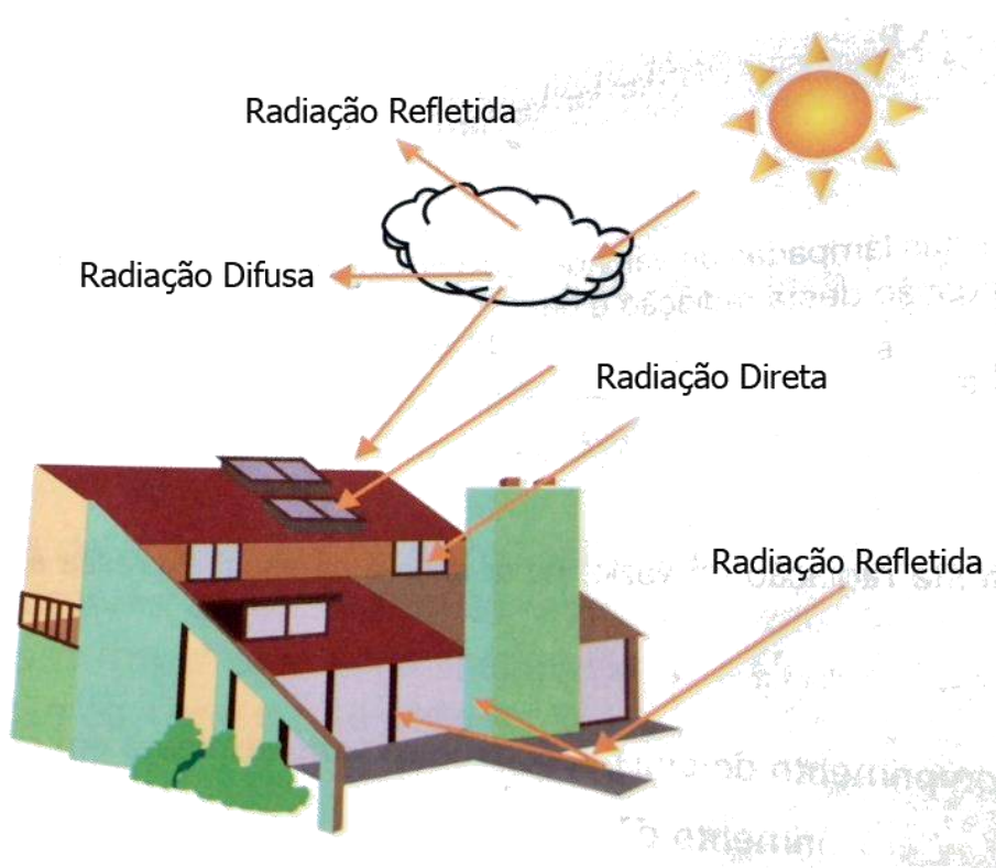
Figura 30: Tipos de radiação solar, disponível em: < http://www.ebah.com.br/content/ABAAAAsG8AL/energia-renovaveis?part=4 >, acesso em 05/05/2016.
