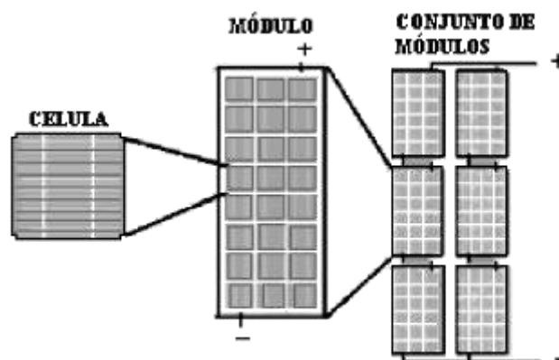
Figura 53: Representação da célula, módulo e painel/arranjo fotovoltaico, disponível em: < http://inergiae.com.br/site/paineis-fotovoltaicos/ >. Acesso em 03/06/2016.
