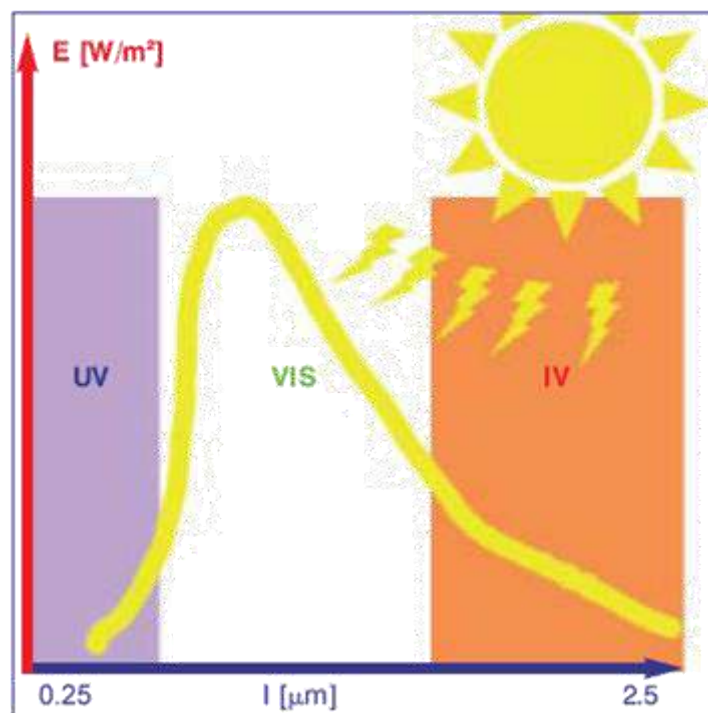
Figura 28: Comportamento da radiação solar em relação ao espectro eletromagnético, disponível em: < http://energiasrenovaveis.com/DetalheNoticias.asp?ID_conteudo=102&ID_area=15 >, acesso em 05/05/2016.
