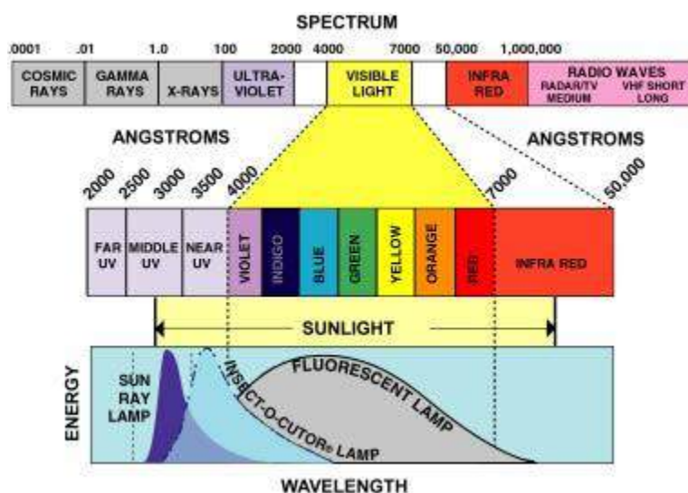
Figura 27: Detalhamento do espectro eletromagnético, disponível em: < http://www.areaseg.com/luz/ >, acesso em 05/05/2016.
