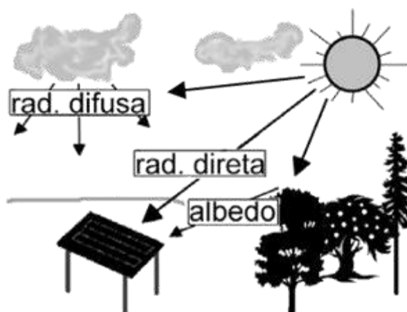
Figura 34: Representação da radiação devido ao albedo, disponível em: < http://www.proceedings.scielo.br/scielo.php?pid=MSC0000000022002000100036&script=sci_arttext >, acesso em 06/05/2016.
