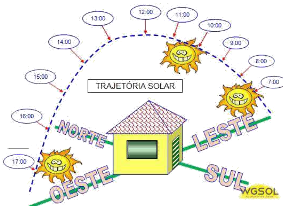
Figura 51: Trajetória solar, disponível em: < http://wgsol.com.br/energia-solar-parte-1/ >, acesso em 06/05/2016.
