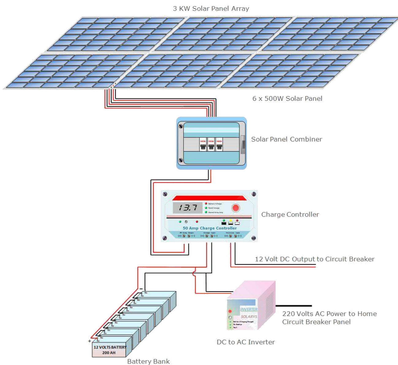
Figura 81: Representação de arranjo FV autônomo de 3KW, disponível em: < https://plus.google.com/106472163037129415313 >, acesso em 14/07/2016.
