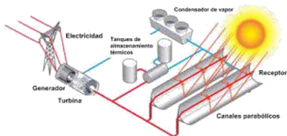
Figura 4: Geração de vapor para acionamento de conjunto turbina + gerador através de coletores côncavos, disponível em: < http://www.sustentator.com/blog-es/2009/04/planta-solar-termica-mas-grande-del-mundo-a-ser-construida-en-arizona/ >. Acesso em 02/06/2016.
