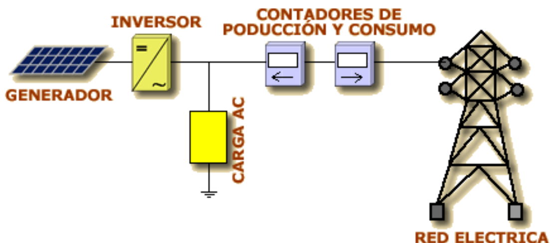
Figura 90: Diagrama esquemático de sistema FV interligado a rede utilizando dois medidores (produção e consumo), disponível em: < http://www.energiasolar.com.es/seccion/placa-solar-luz/instalaciones-conectadas-a-red >, acesso em 14/07/2016.
