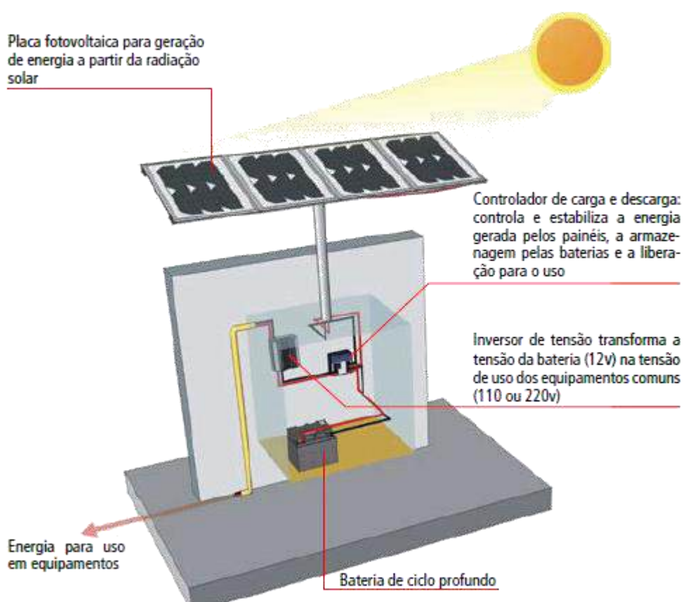
Figura 75: representação esquemática do fluxo de energia em um sistema fotovoltaico autônomo, disponível em: < http://www.metalica.com.br/energia-a-abundancia-solar >, acesso em 14/07/2016.
