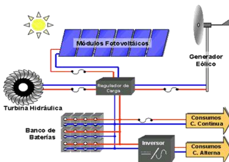
Figura 100: Sistema híbrido incluindo turbina hidráulica, disponível em: < http://blogdfely.blogspot.com.br/2010/11/sistemas-hibridos.html >, acesso em 15/07/2016.
