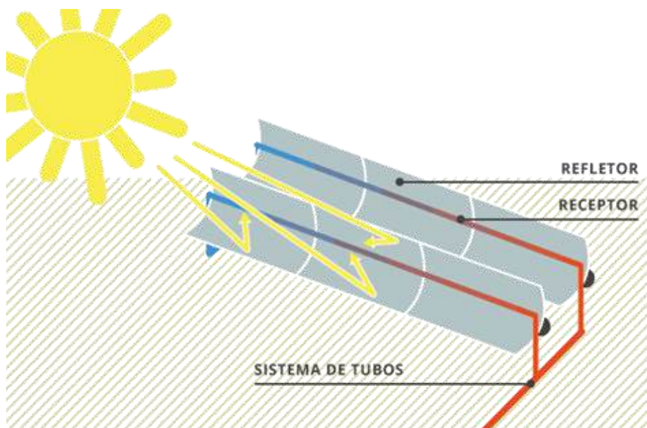
Figura 12: Representação simplificada do sistema térmico via coletores côncavos, disponível em: < http://energiaheliotermica.gov.br/pt-br/energia-heliotermica/como-funciona >, acesso em 02/06/2016.
