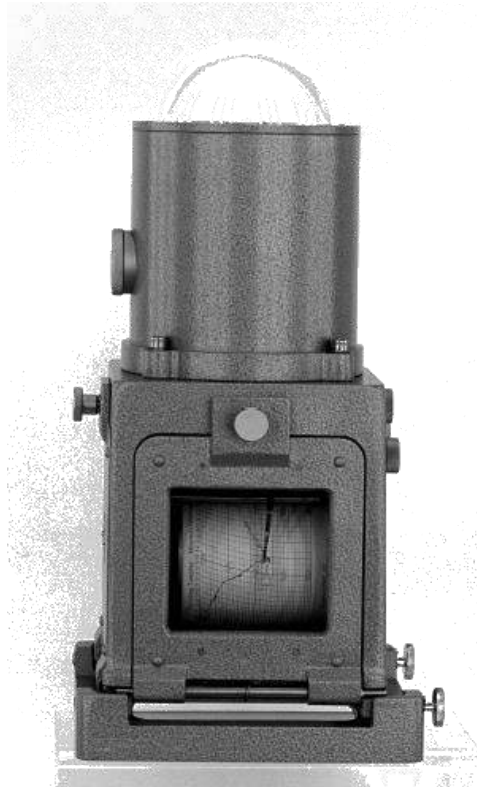
Figura 43: Aspecto visual do actinógrafo, disponível em: < https://www.flickr.com/photos/87668408@N04/8024342930 >, acesso em 06/05/2016.
