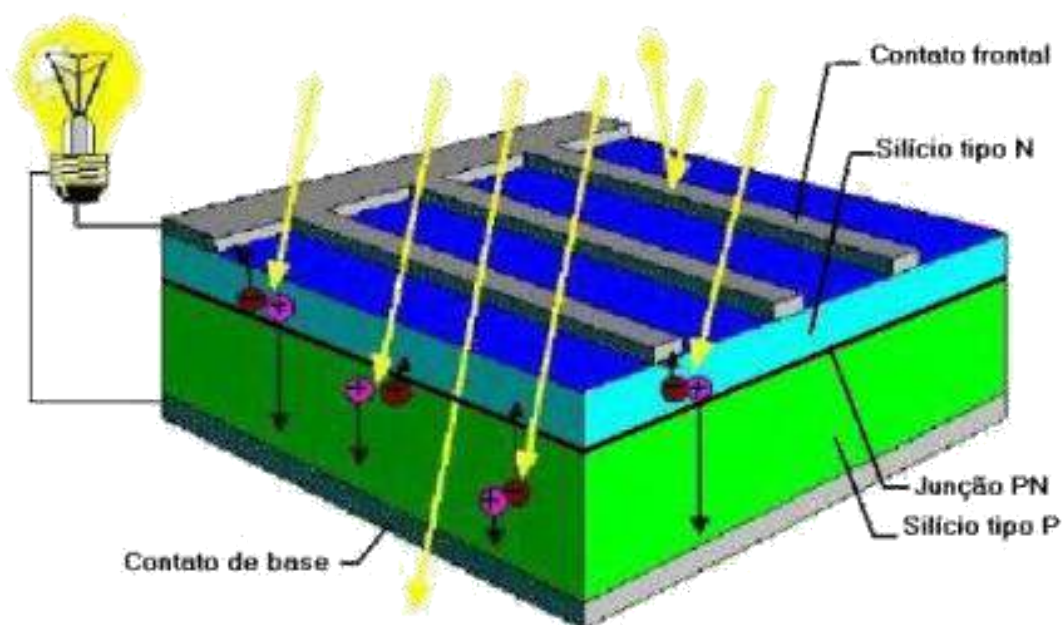
Figura 24: Representação simplificada do efeito fotovoltaico em uma célula fotovoltaica, disponível em: < http://www.ebah.com.br/content/ABAAFrAgAK/metodos-dimensionamento-sistemas-fotovoltaicos?part=2 >, acesso em 19/08/2016.
