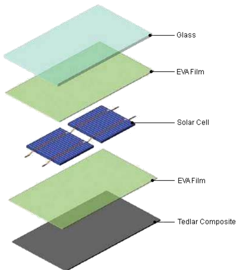
Figura 57: Vista explodida do painel solar, disponível em: < http://produto.mercadolivre.com.br/MLB-706861504-painel-solar-75w-JM >, acesso em 24/06/2016.
