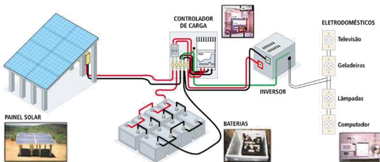
Figura 73: Exemplo de sistema fotovoltaico autônomo, disponível em: < http://www2.aneel.gov.br/aplicacoes/atlas/energia_solar/3_3_2.htm >, acesso em 25/06/2016.
