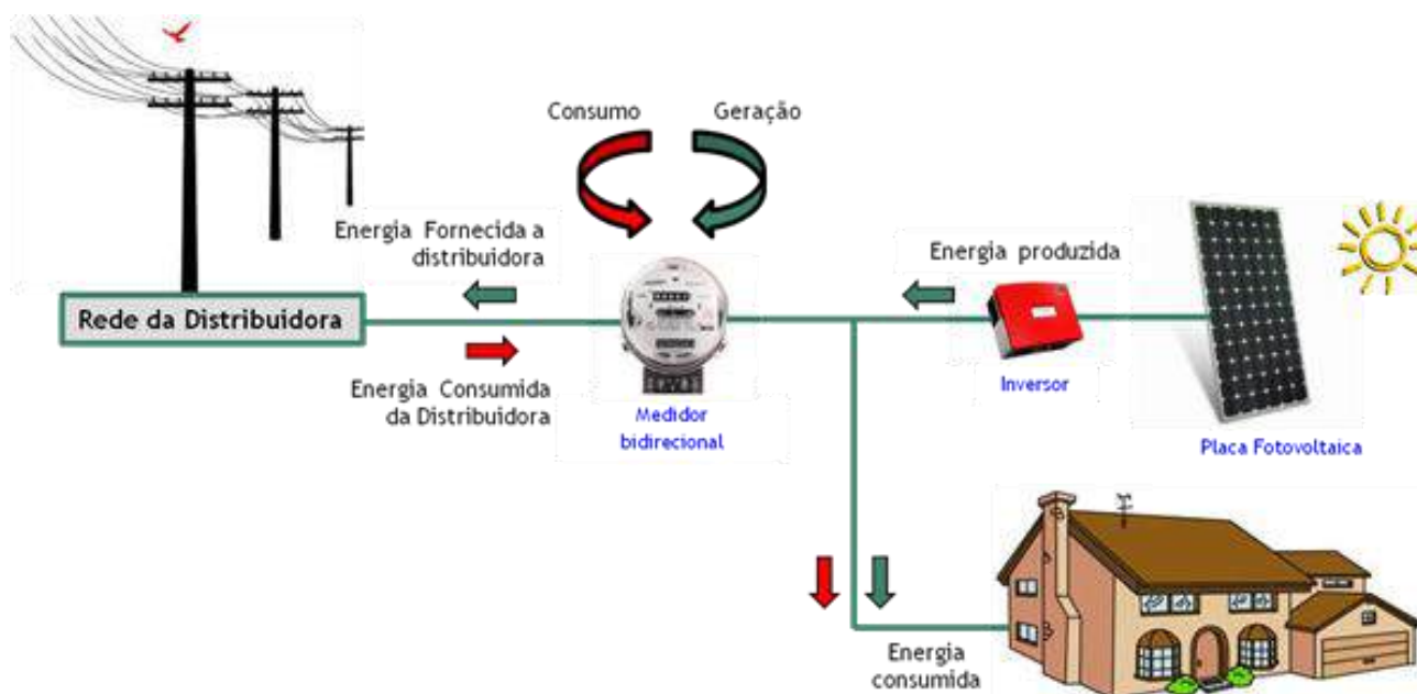
Figura 89: Exemplo de sistema FV interligado a rede utilizando medidor bidirecional, disponível em: < http://www.viridian.com.br/tecnologia/energia+solar+fotovoltaica/4 >, acesso em 14/07/2016.
