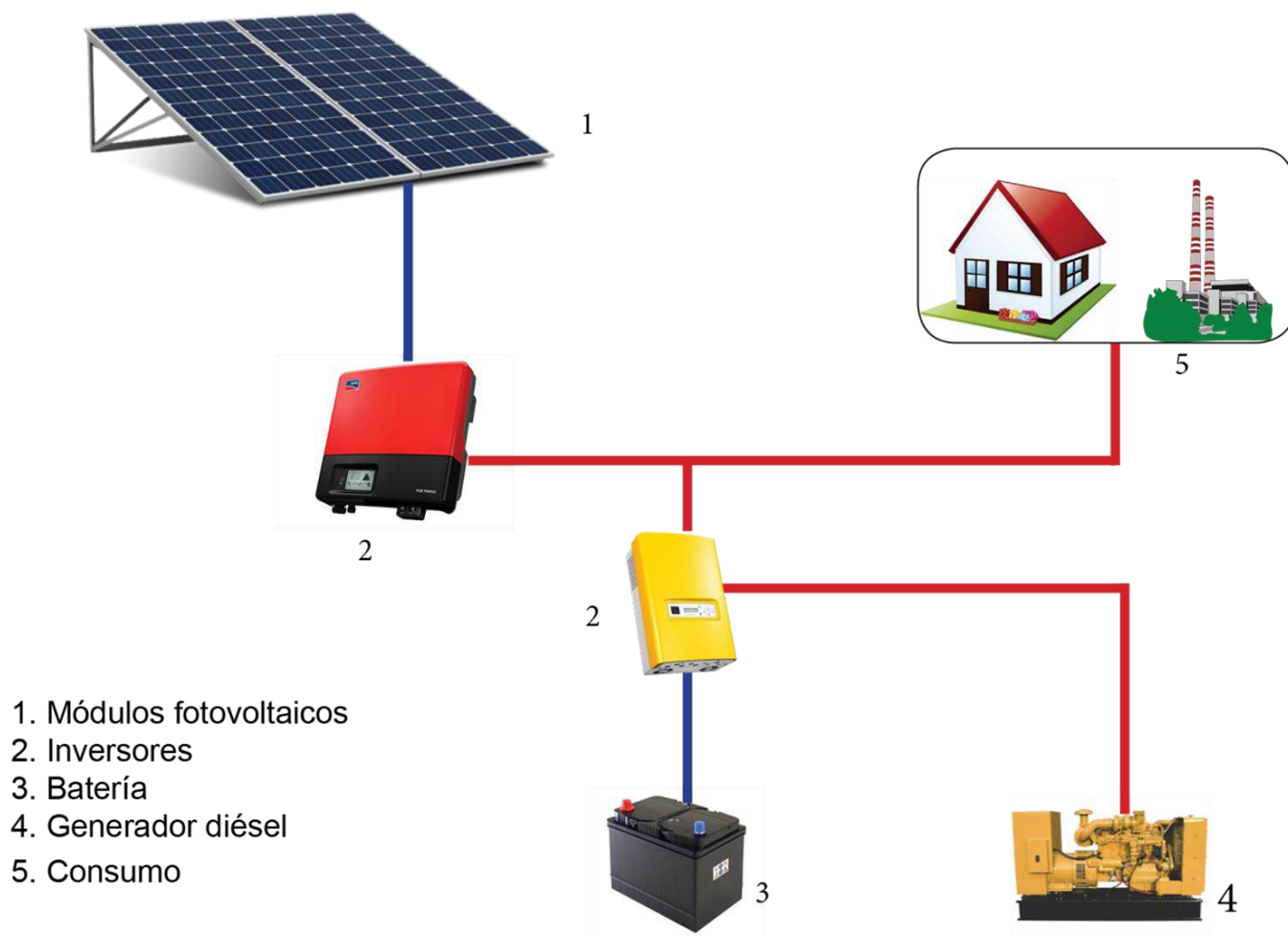
Figura 95: Sistema de geração híbrida com 2 inversores, disponível em: < http://www.sitecnosolar.com/pt/sistema-hibrido-compatible-con-generator-diesel-sin-red/ >, acesso em 15/07/2016.
