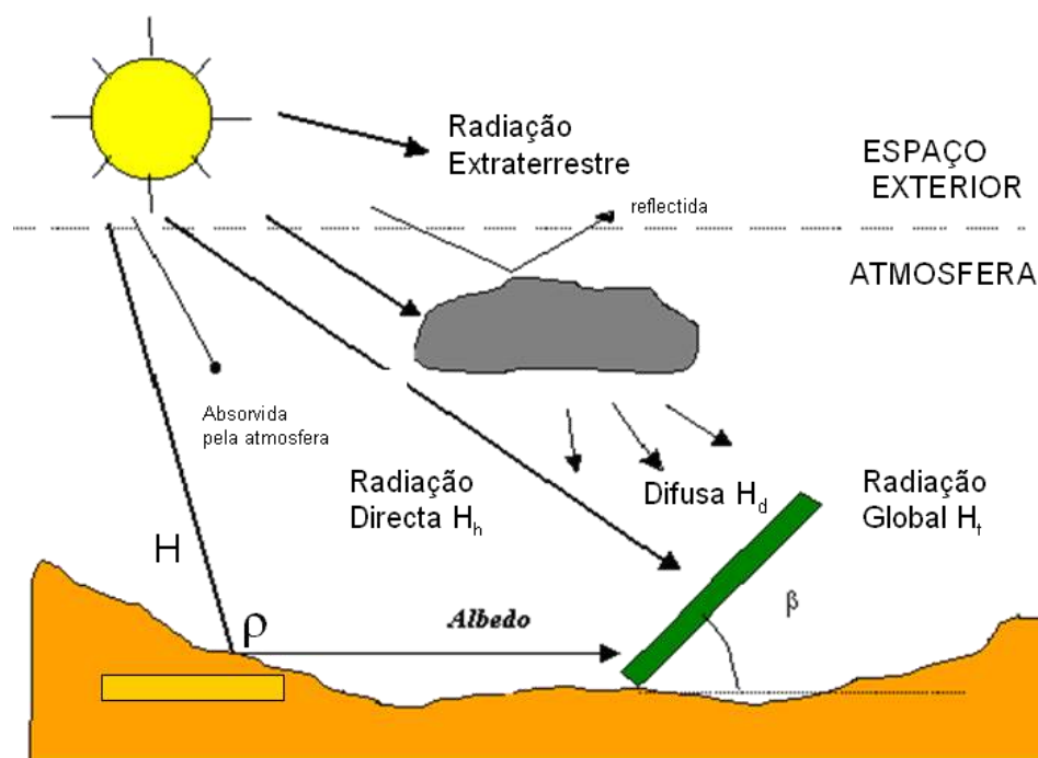
Figura 36: Representação dos tipos de radiações solares, disponível em: < http://docplayer.com.br/8395823-Requisitos-para-a-certificacao-pv.html >, acesso em 06/05/2016.
