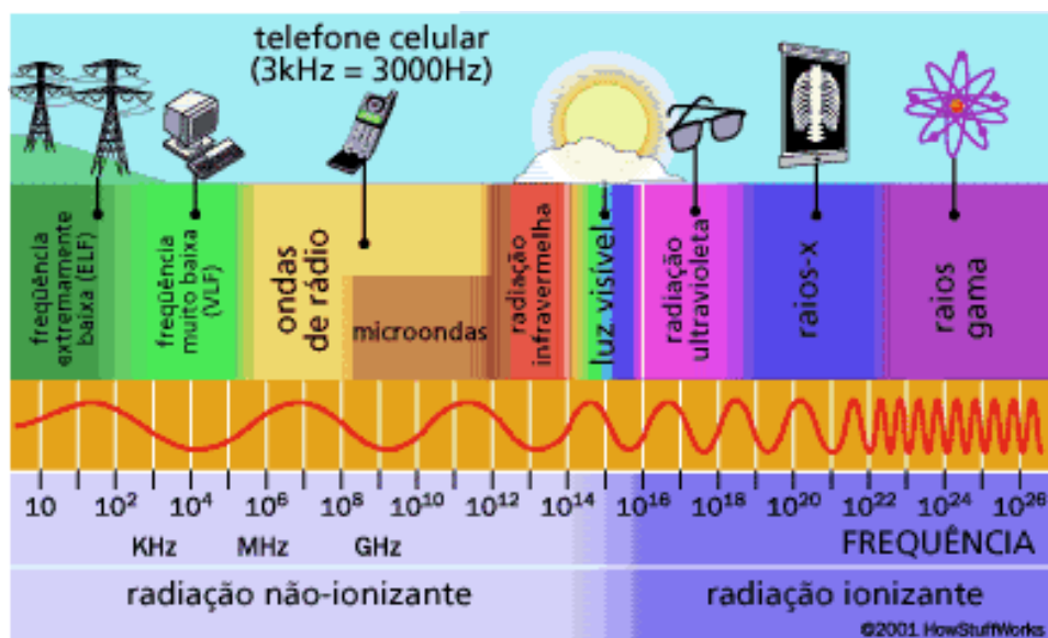
Figura 26: Representação do espectro eletromagnético, disponível em: < http://blog.clickgratis.com.br/radicacoes2/ >, acesso em 05/05/2016.
