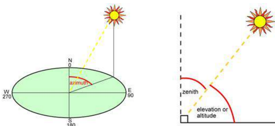
Figura 38: Ângulos relativos à posição do sol, disponível em: < http://docplayer.com.br/12817568-Sistema-de-seguimento-solar-em-producao-de-energia-fotovoltaica.html >, acesso em 06/05/2016.
