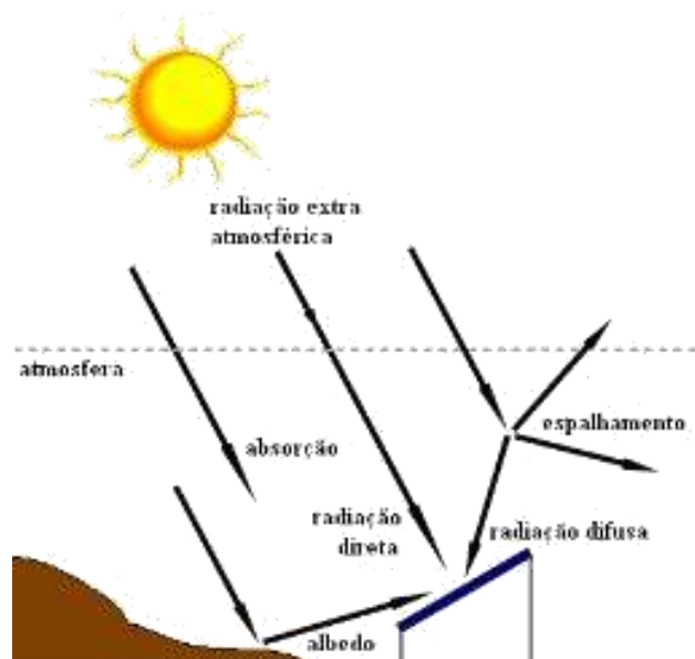
Figura 30: Tipos de radiação solar, disponível em: < http://www.ebah.com.br/content/ABAAAAsG8AL/energia-renovaveis?part=4 >, acesso em 05/05/2016.
