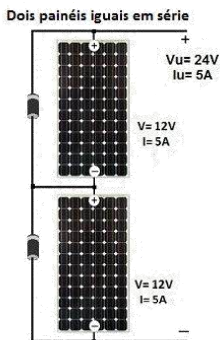
Figura 61: Exemplo de conexão série entre dois painéis com as mesmas especificações elétricas, disponível em: < http://www.mpptsolar.com/pt/paineis-solares-em-serie.html >. Acesso em 03/06/2016.
