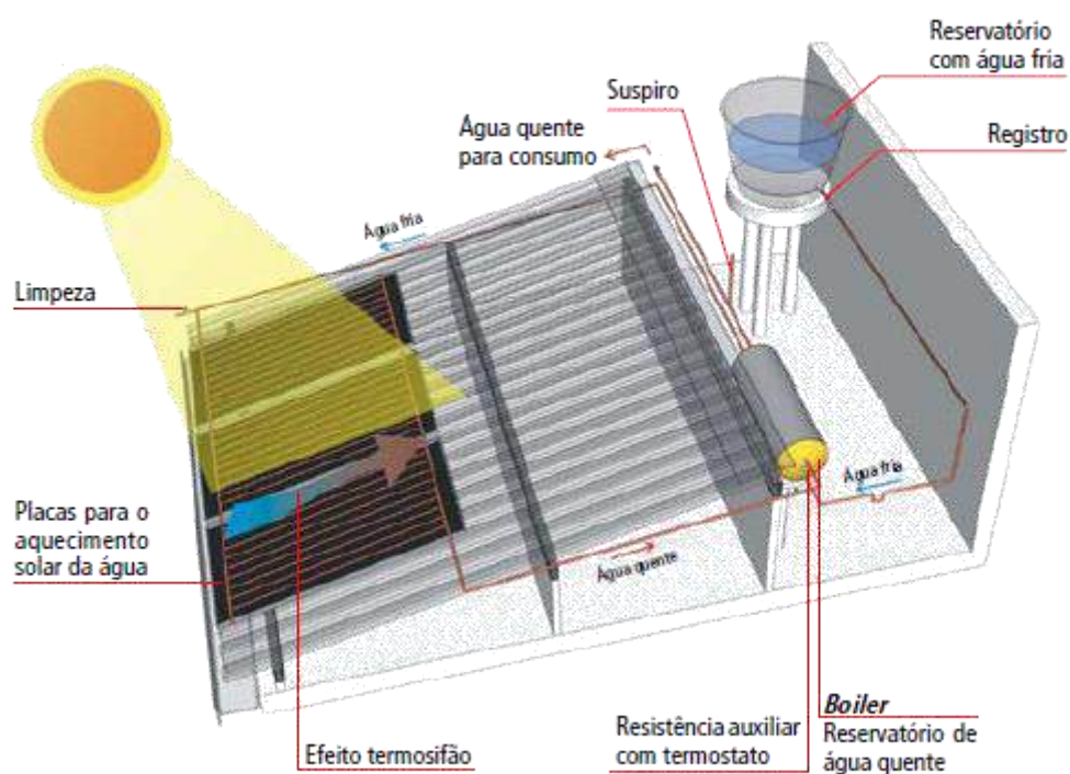
Figura 68: Exemplo de sistema de aquecimento via energia solar térmica por circulação "natural", disponível em: < http://www.metalica.com.br/energia-a-abundancia-solar >, acesso em 14/07/2016.
