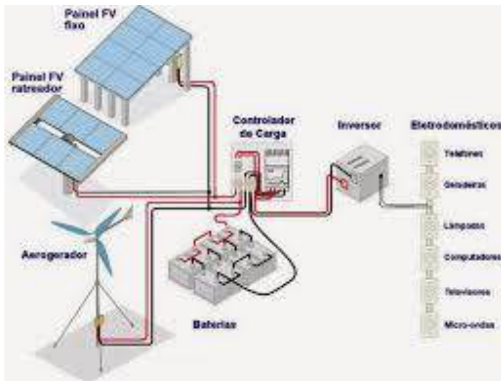
Figura 93: Exemplo de sistema FV híbrido constituído por painéis FV fixos, painéis FV com rastreador solar e aero geradores, disponível em: < https://processo-industrial.blogspot.com.br/2014_01_01_archive.html >, acesso em 15/07/2016.
